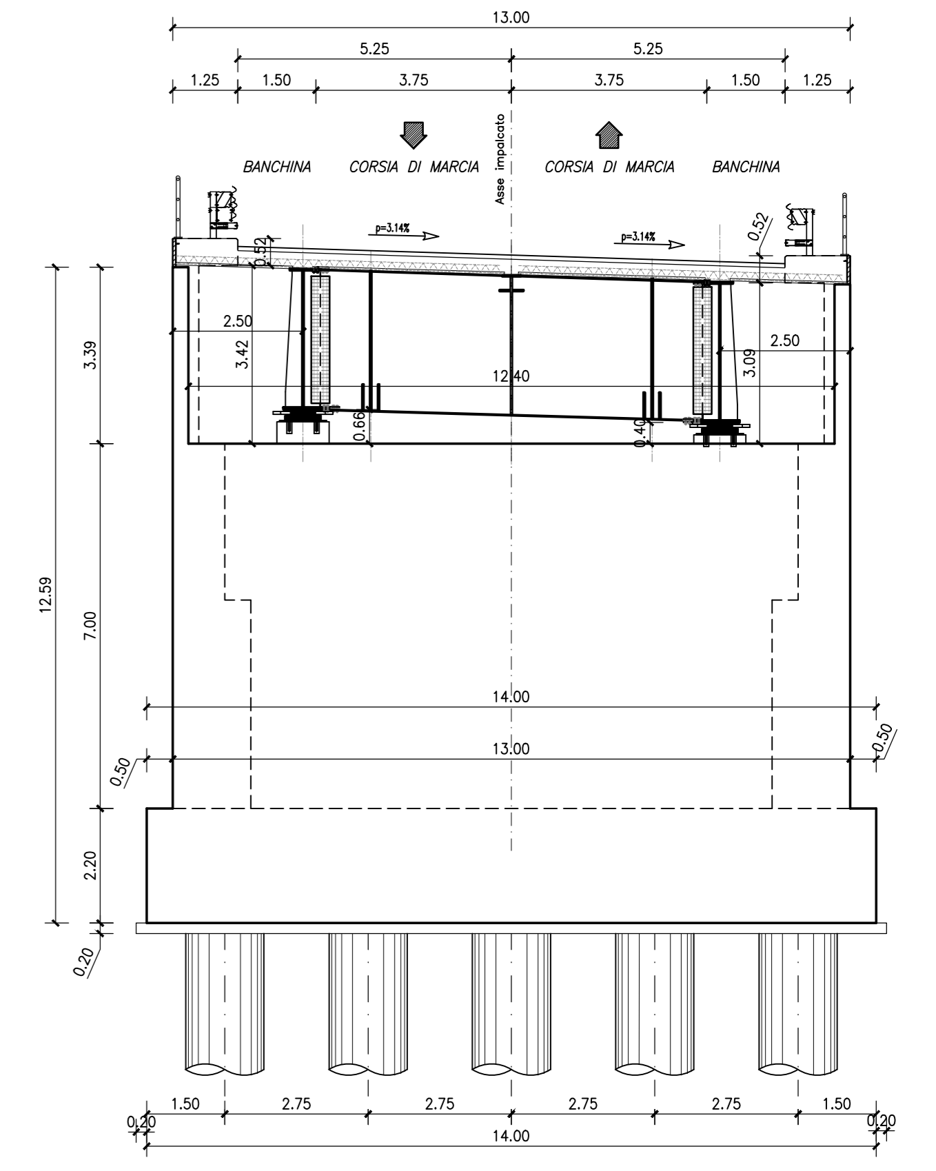
SEZIONE TRASVERSALE CORRENTE – Scala 1:100
