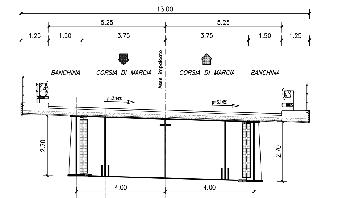
SEZIONE TRASVERSALE CORRENTE – Scala 1:100
