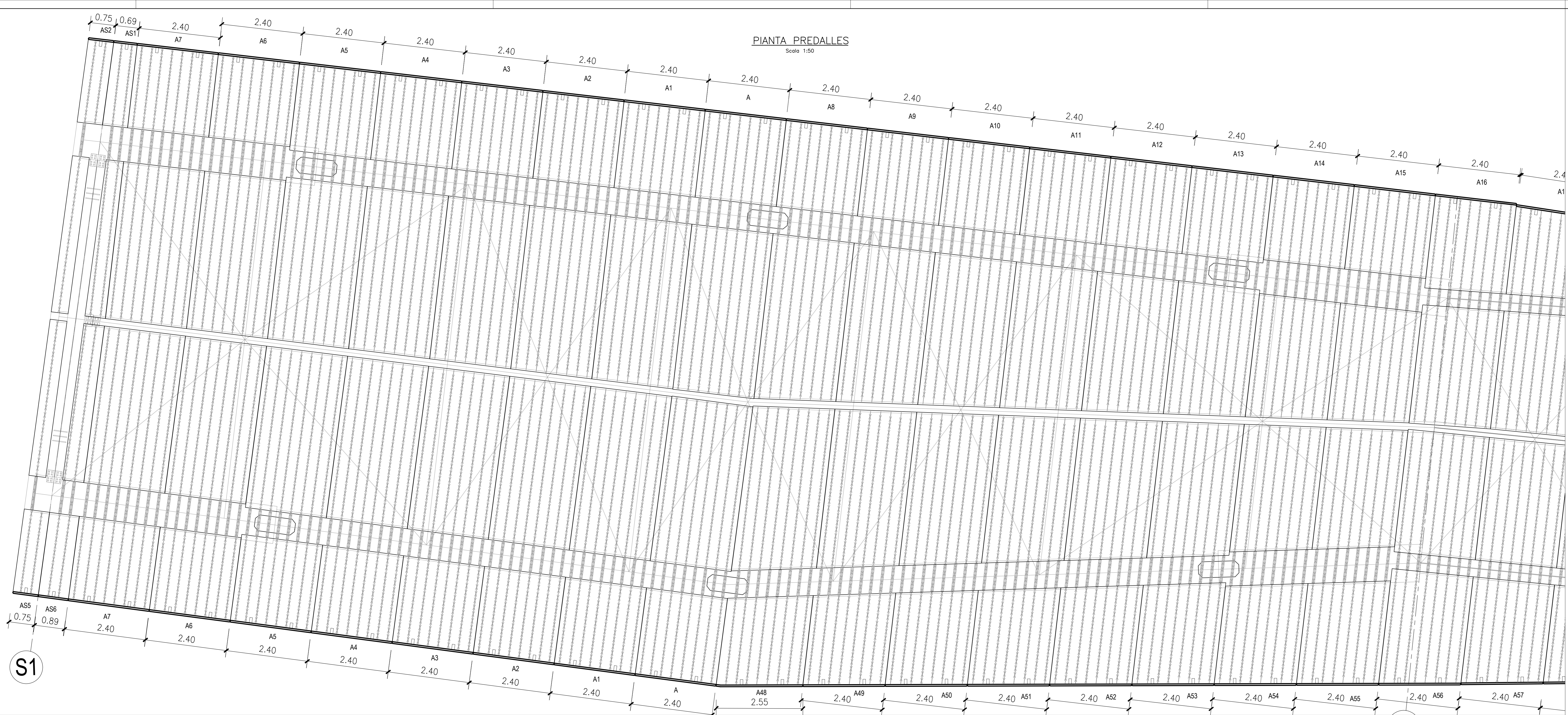
PIANTA PREDALLES Scala 1:50
