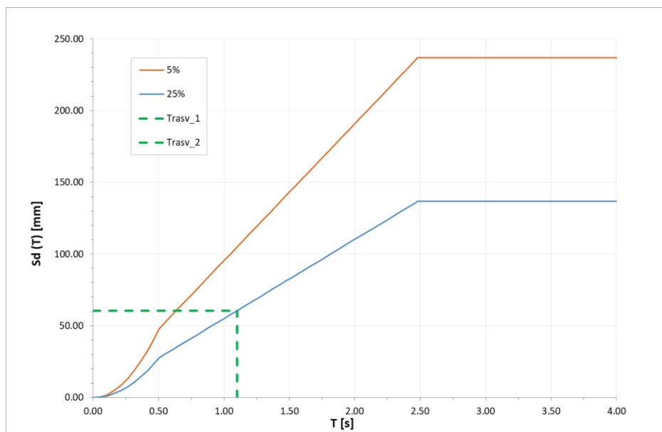
Figura 25 – Relazione fra spostamento di soglia e periodo di progetto (direzione trasversale)
