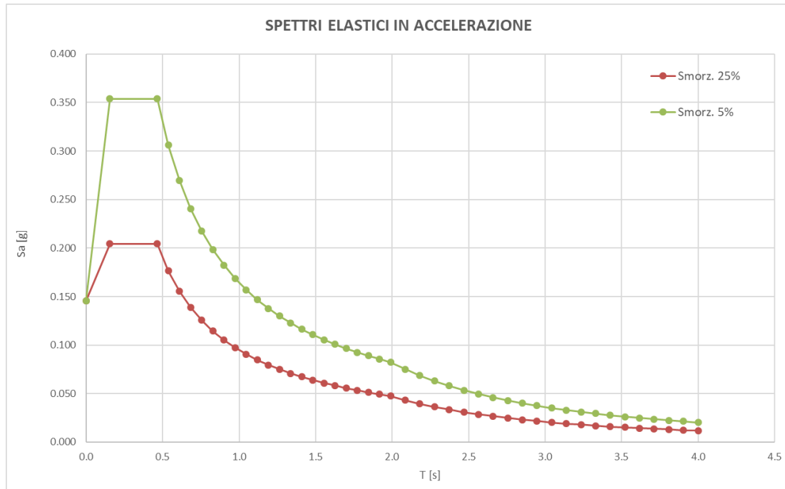
Figura 14 – Spettri elastici in accelerazione allo SLD
