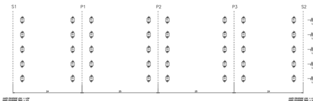
Figura 38 – Schema di appoggi e isolatori
