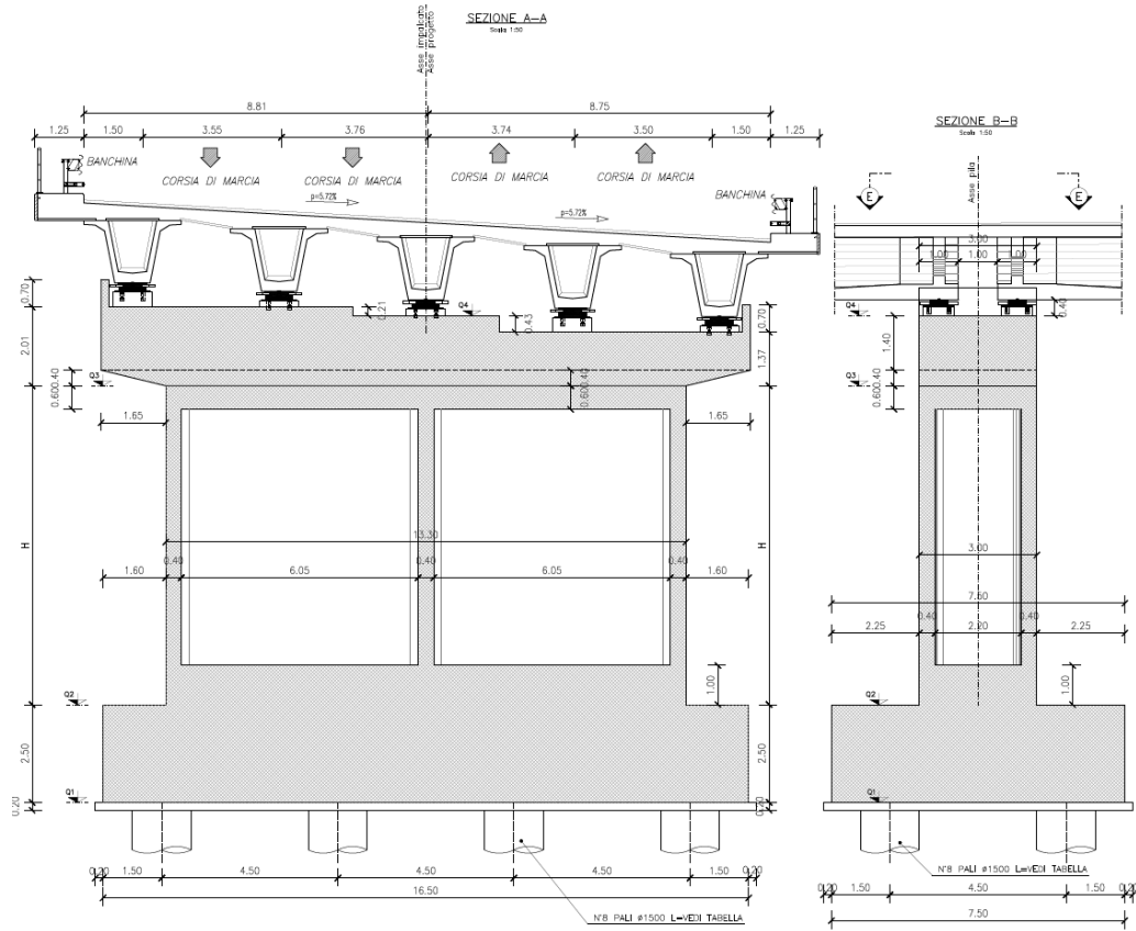
Figura 2 – Pile
