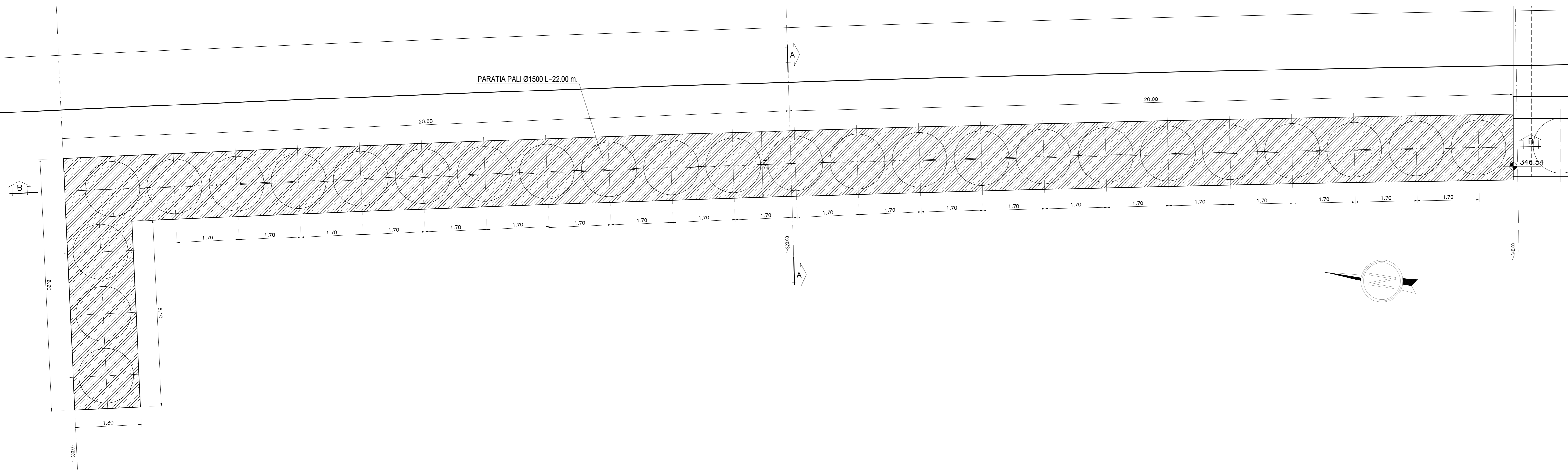
PIANTA PARATIA SX - SCALA 1:50
