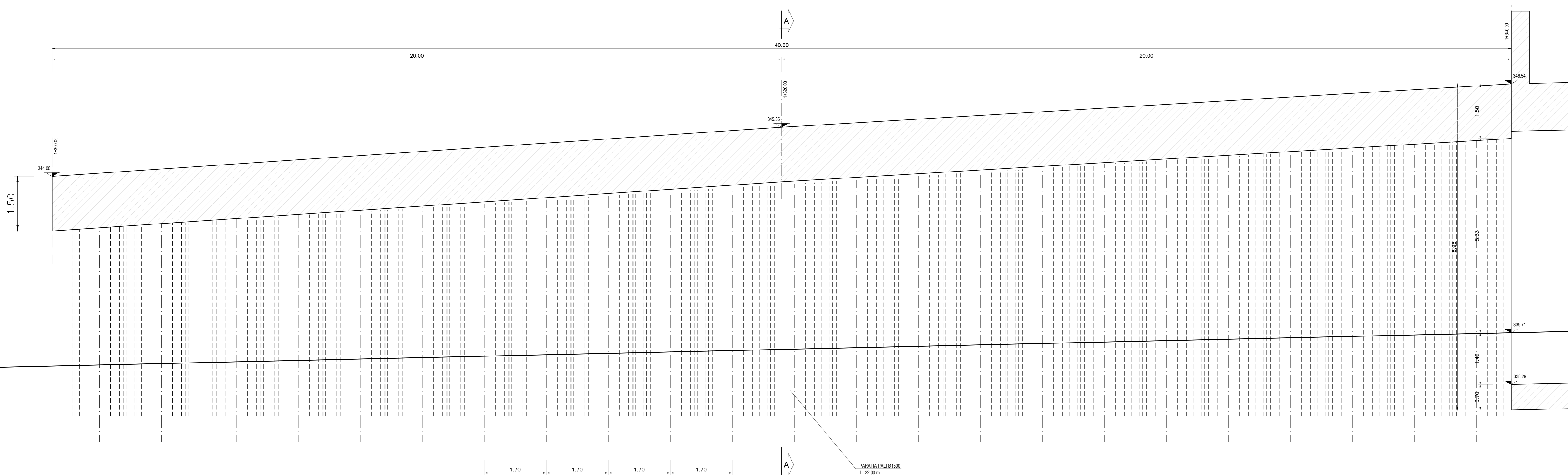
SEZIONE B-B - SCALA 1:50
