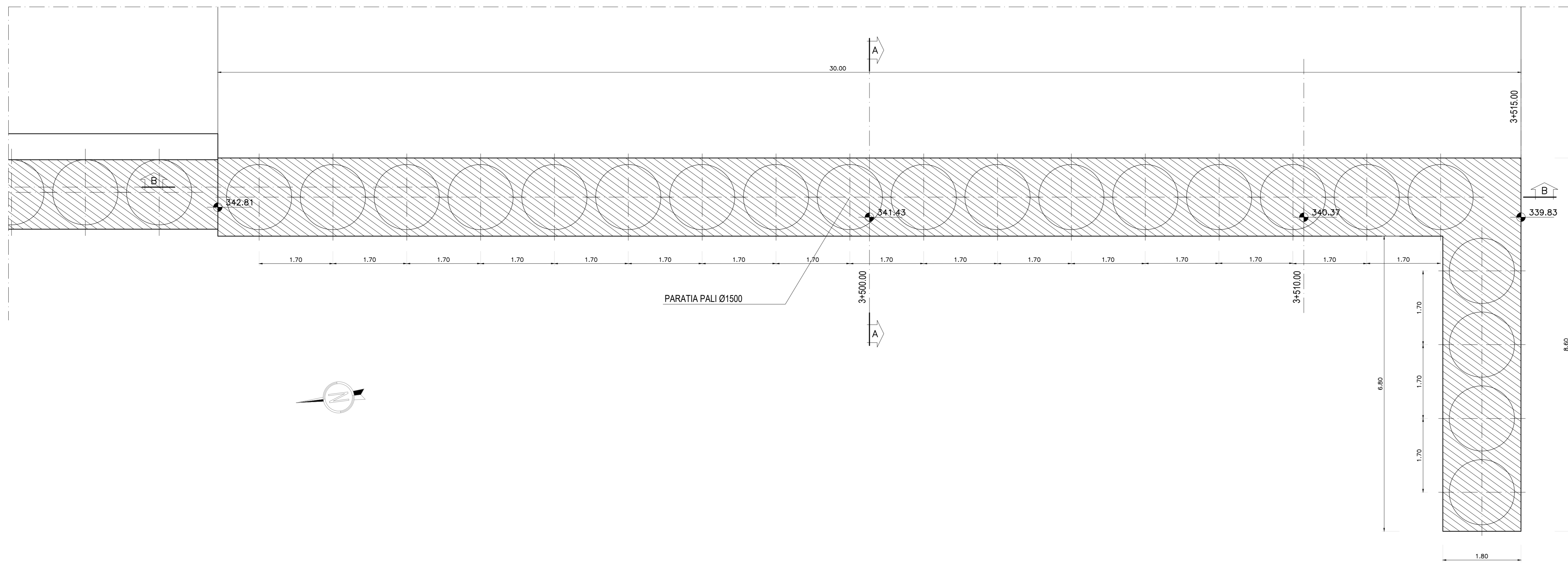
PIANTA PARATIA DX - SCALA 1:50
