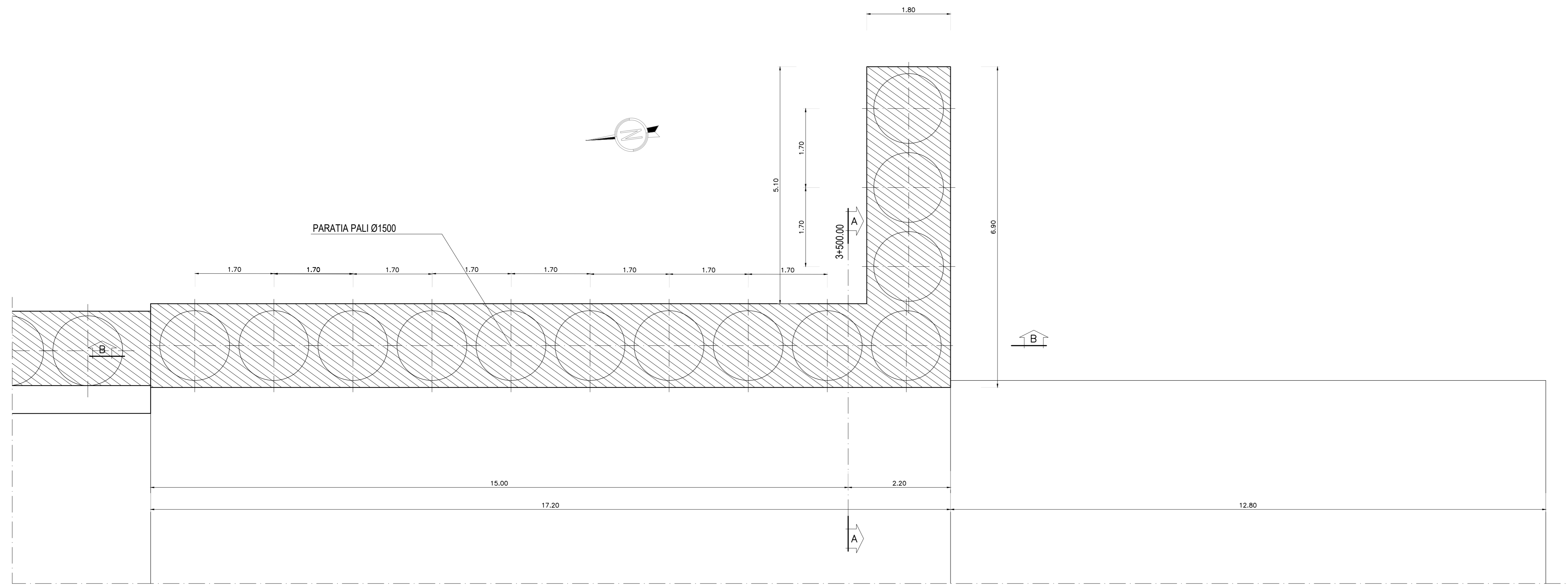
PIANTA PARATIA SX - SCALA 1:50
