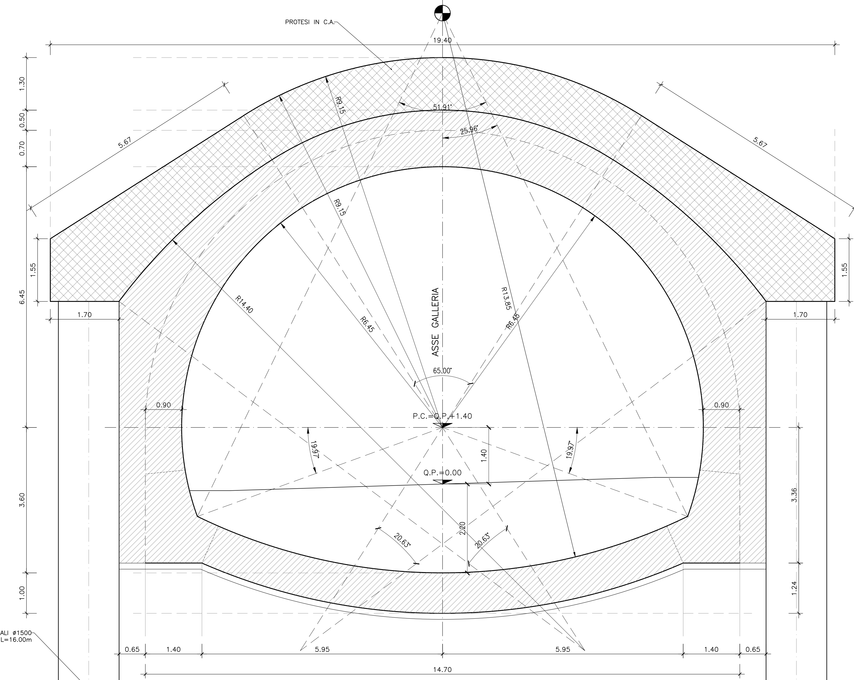
SEZIONE TRASVERSALE A-A - CARPENTERIA -
