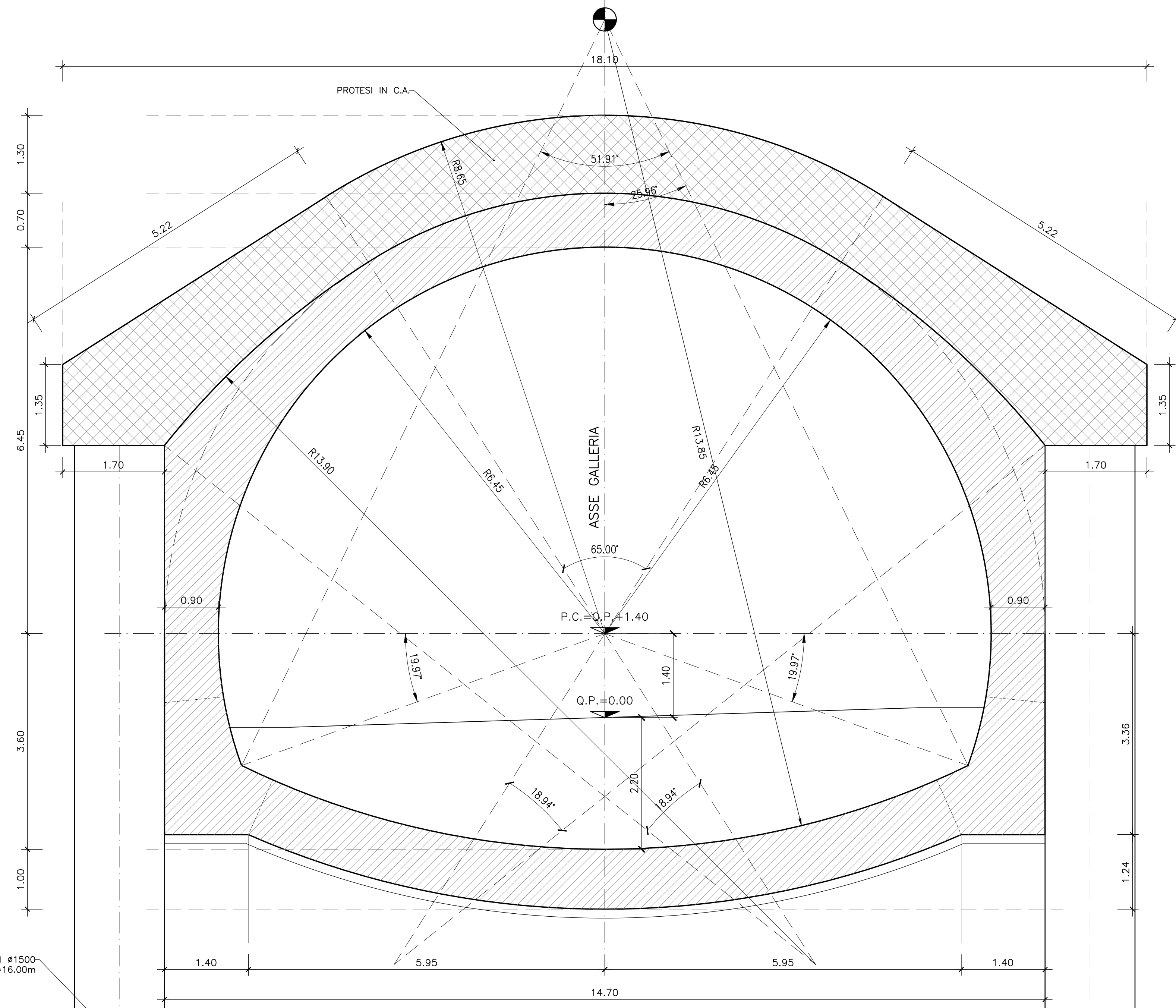
SEZIONE TRASVERSALE B-B - CARPENTERIA -
