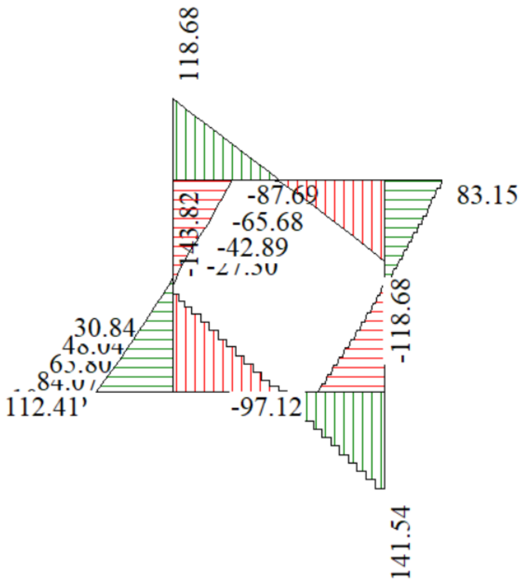
Inviluppo diagrammi del momento flettente – SLU statico e sismico
