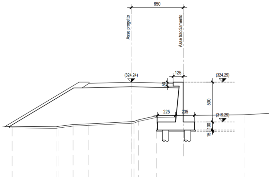
Figura 2.2 – Sezione opera di sostegno di tipo 2, Hparam=5.0m
