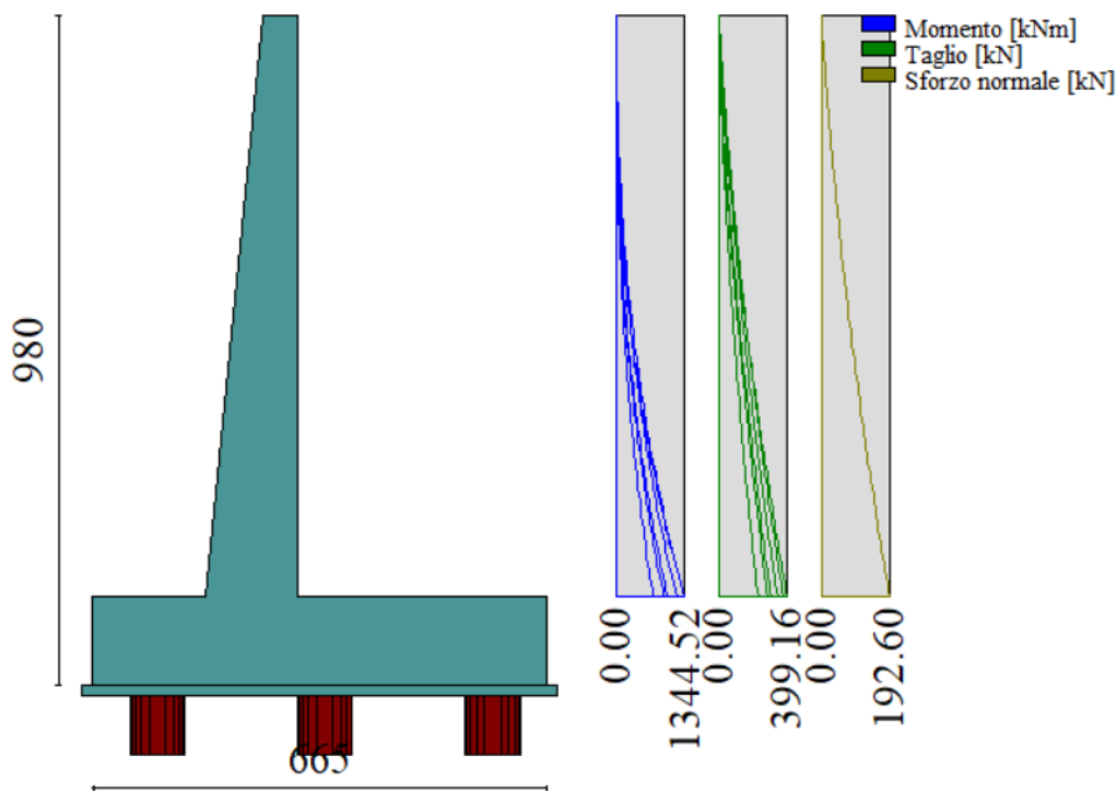
Inviluppo sollecitazioni sul muro
