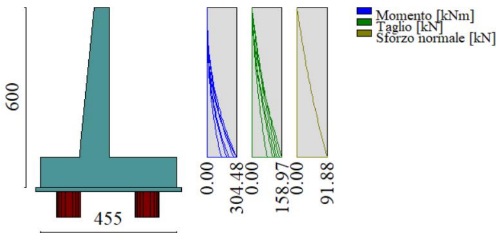
Inviluppo sollecitazioni sul muro
