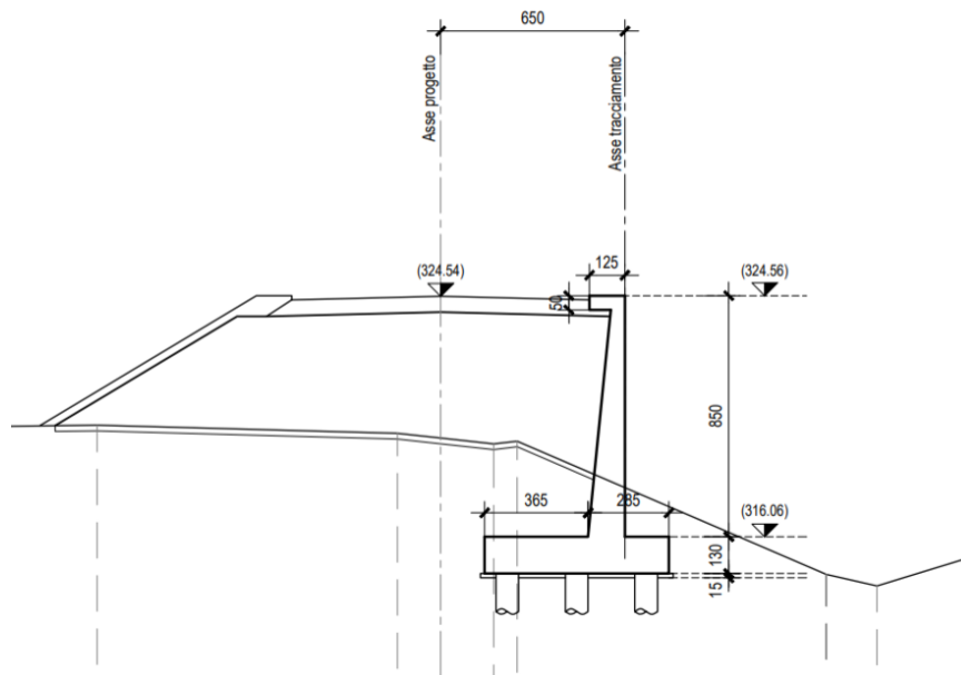
Figura 2.3 – Sezione opera di sostegno di tipo 3, Hparam=8.5m
