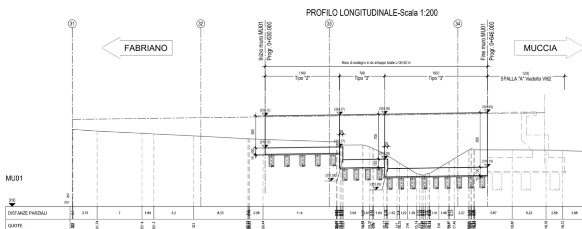
Figura 2.1 - Profilo longitudinale opera di sostegno MU01
