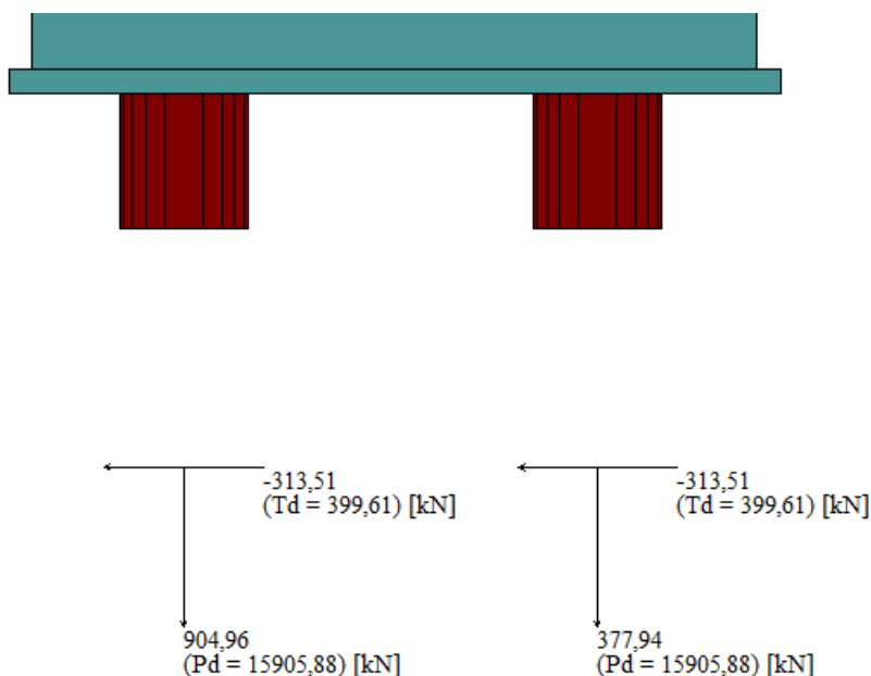
Sollecitazioni massime testa palo – SLU
