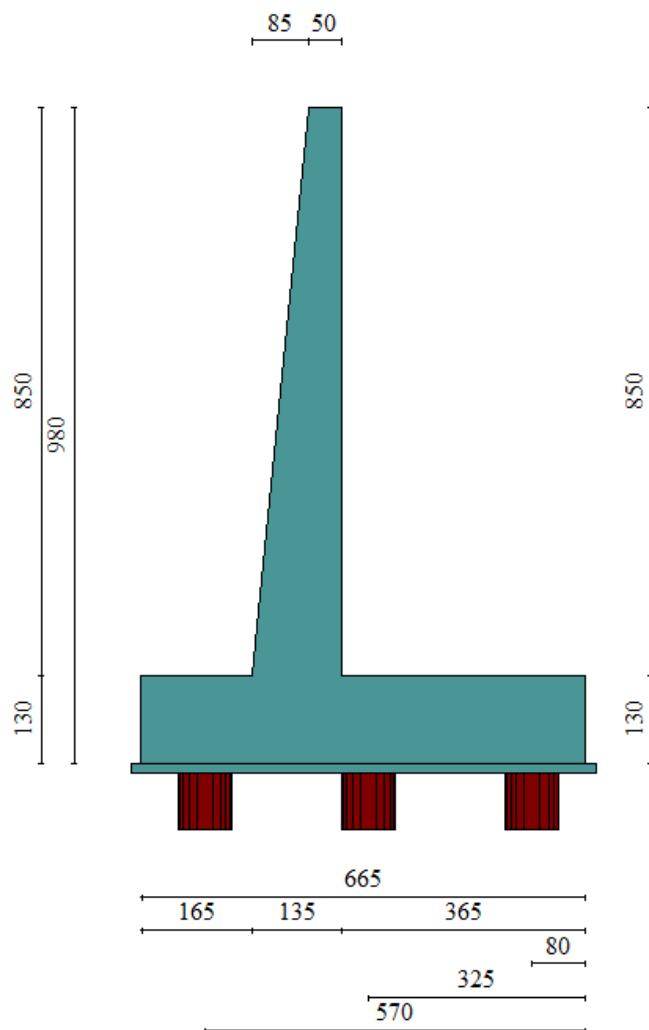
Geometria muro
