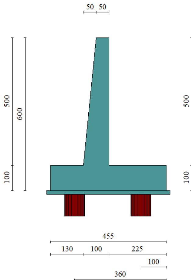
Geometria muro
