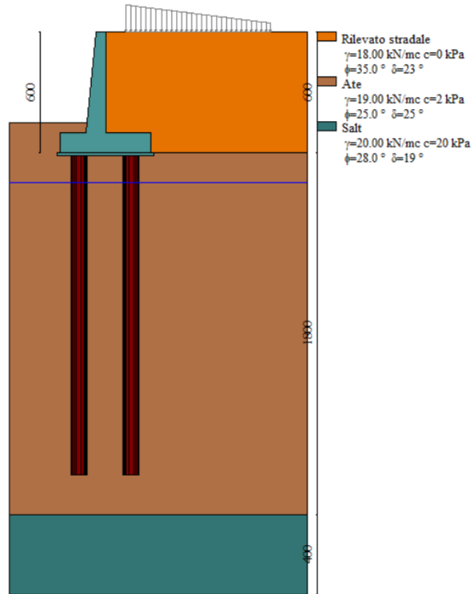
Modello di calcolo muro su PALI
