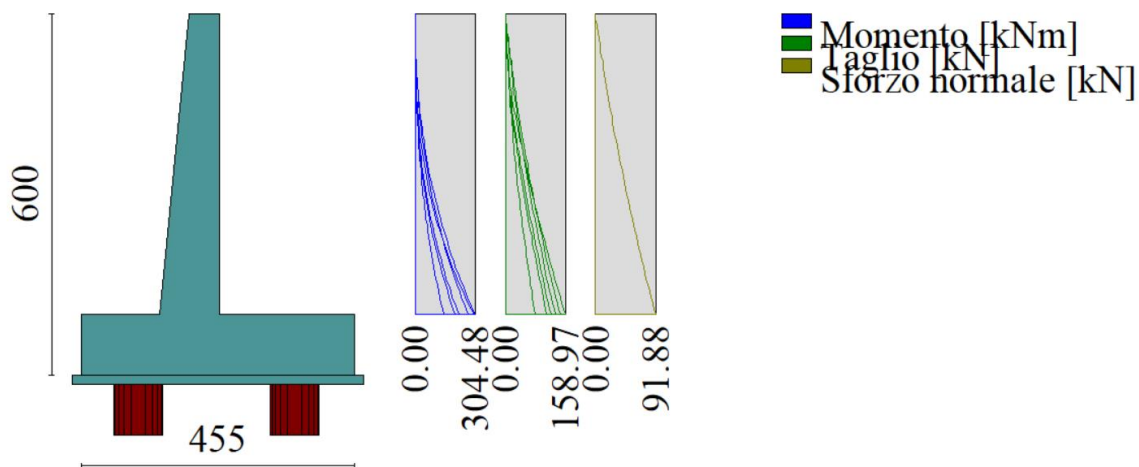
Inviluppo sollecitazioni sul muro
