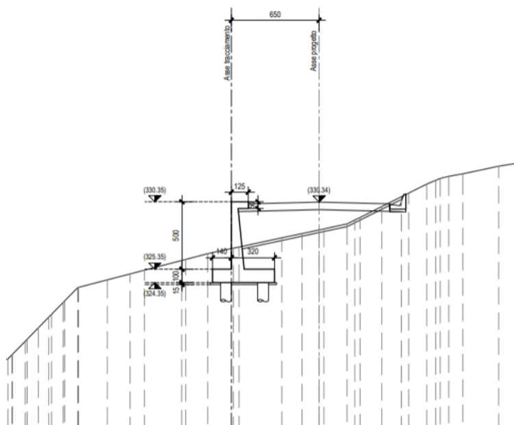
Figura 2.3 – Sezione opera di sostegno di tipo 2, Hparam=5m
