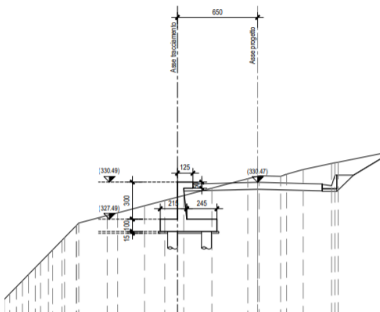
Figura 2.4 – Sezione opera di sostegno di tipo 2, Hparam=3m
