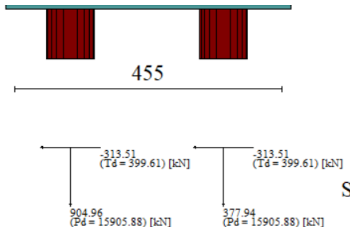
Sollecitazioni massime testa palo – SLU
