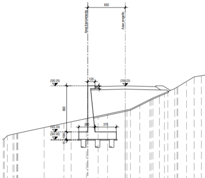
Figura 2.2 – Sezione opera di sostegno di tipo 3, Hparam=8.0m
