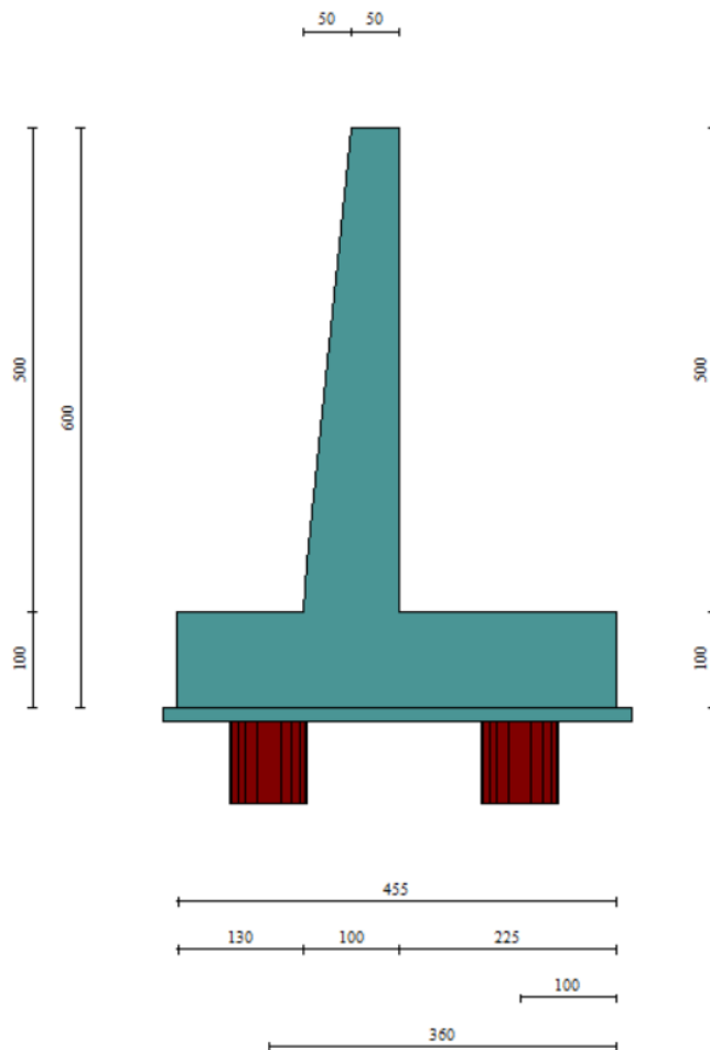
Geometria muro
