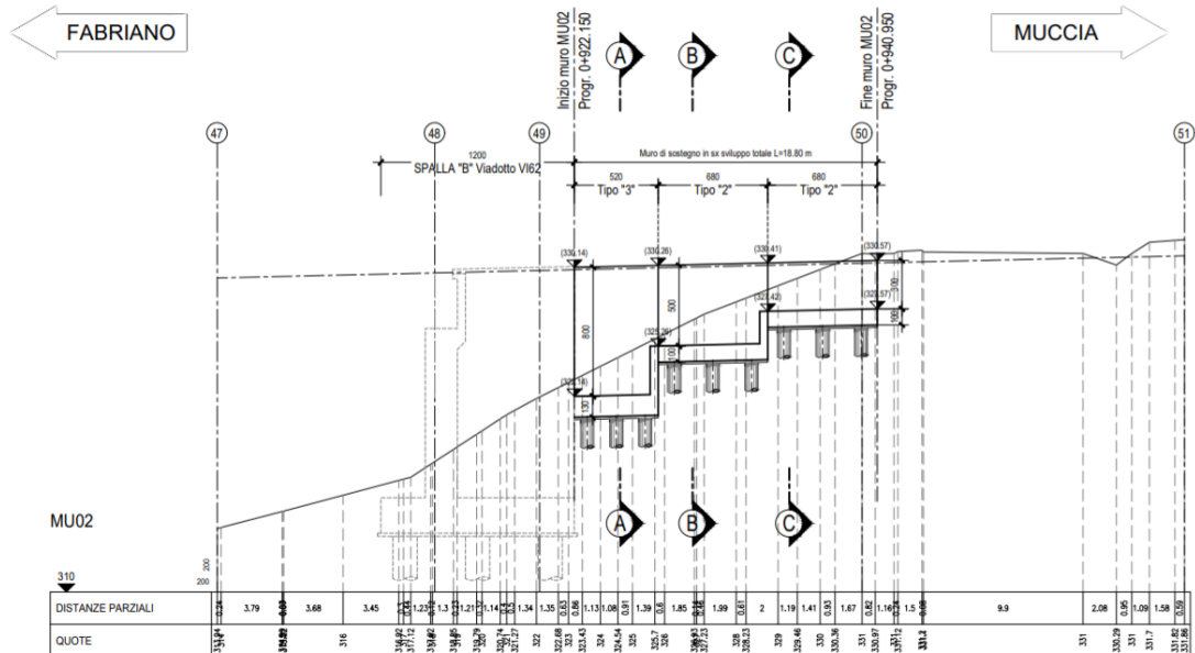
Figura 2.1 - Profilo longitudinale opera di sostegno MU02
