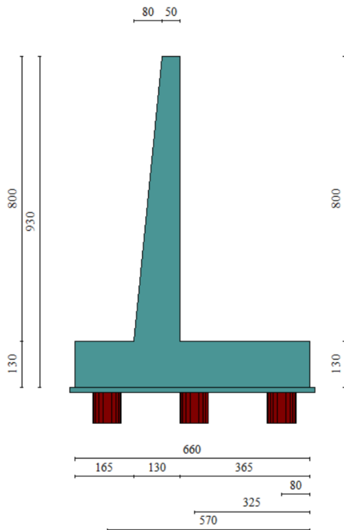
Geometria muro
