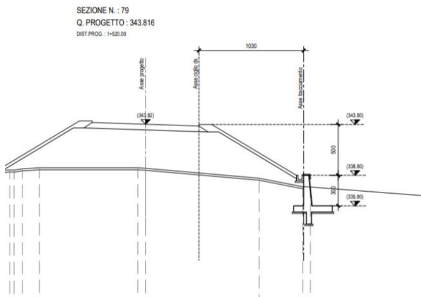
Figura 2.2 – Sezione opera di sottoscarpa di tipo 1, Hparam=3.0m
