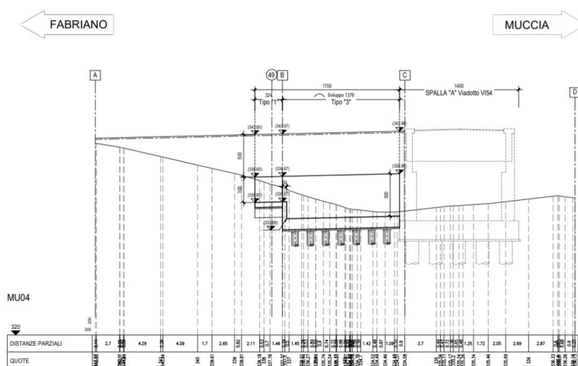
Figura 2.1 - Profilo longitudinale opera di sottoscarpa MU04
