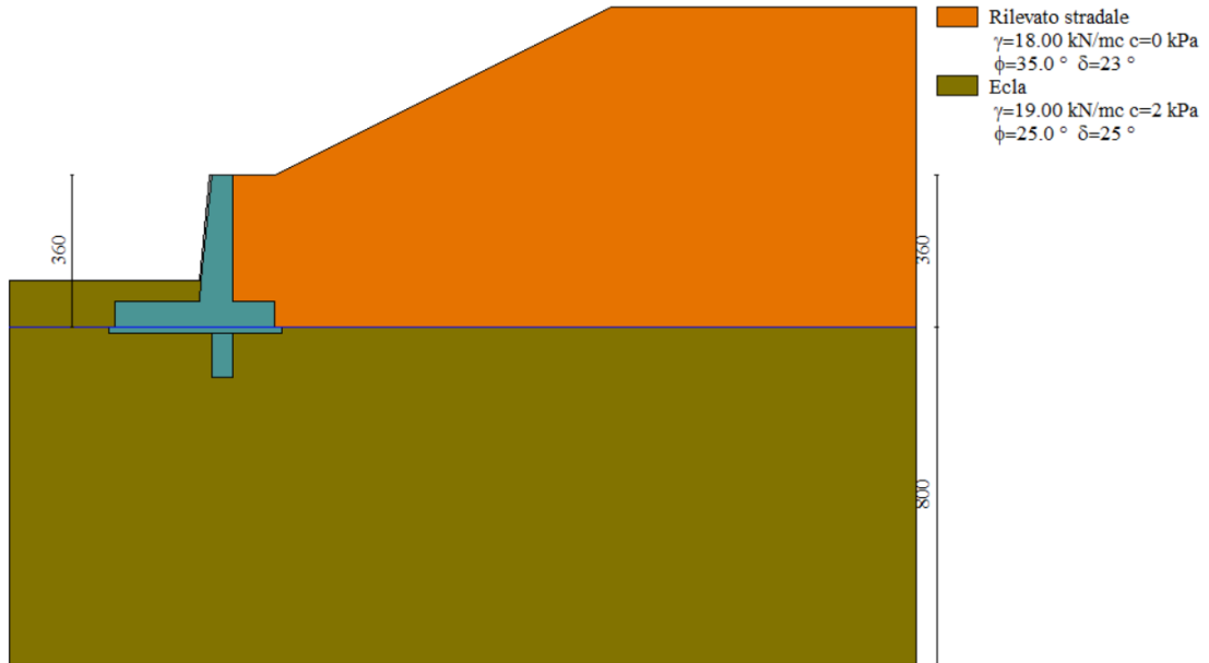
Modello di calcolo muro
