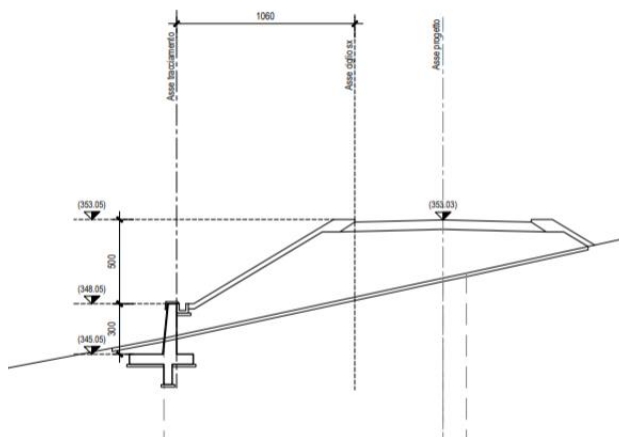
Figura 2.2 – Sezione opera di sottscarpa di tipo 1, Hparam=3.0m
