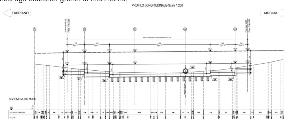
Figura 2.1 - Profilo longitudinale opera di sottoscarpa MU06
