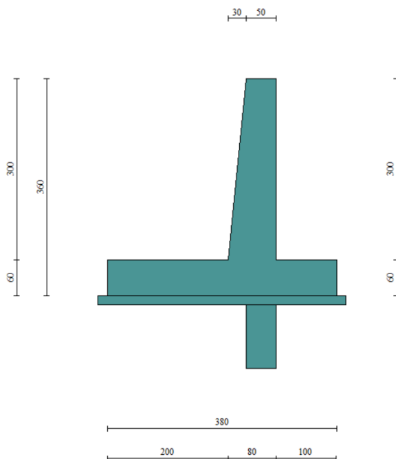
Geometria muro
