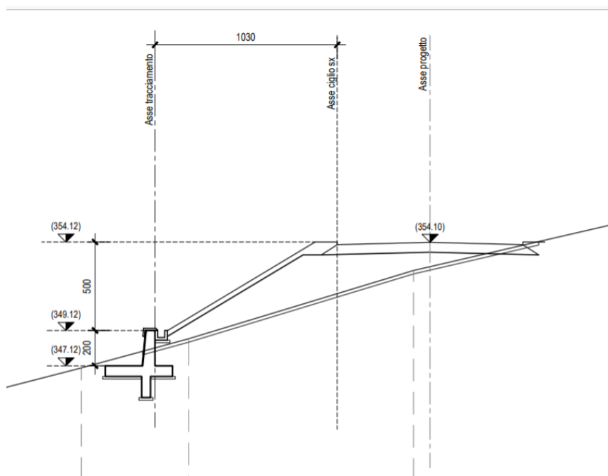
Figura 2.2 – Sezione opera di sottoscarpa di tipo 1, Hparam=2.0m
