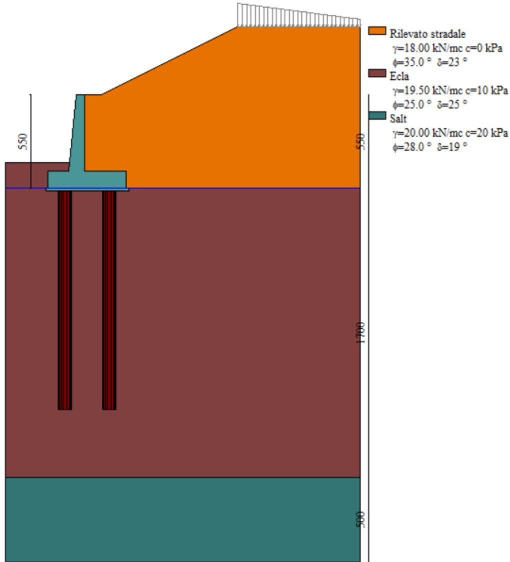
Modello di calcolo muro
