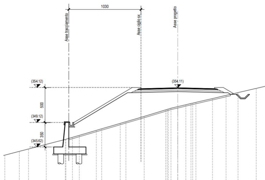
Figura 2.2 – Sezione opera di sottoscarpa di tipo 1, Hparam=2.0m
