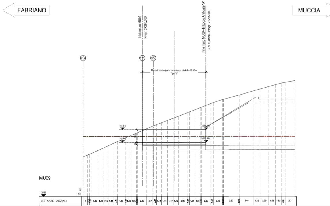
Figura 2.1 - Profilo longitudinale opera di sottoscarpa MU09
