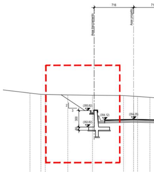
Figura 2.2 – Sezione opera di controripa di tipo 1, Hparam=3.0m
