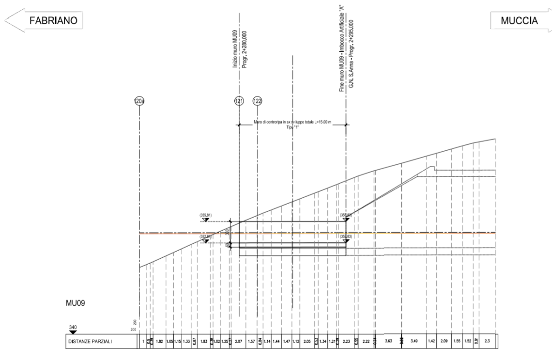
Figura 2.1 - Profilo longitudinale opera di sottoscarpa MU11
