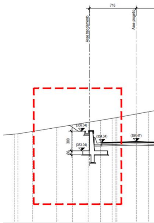
Figura 2.2 – Sezione opera di controripa di tipo 1, Hparam=3.0m
