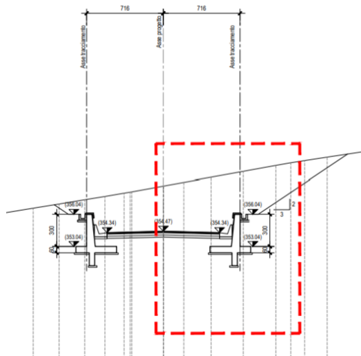
Figura 2.2 – Sezione opera di controripa di tipo 1, Hparam=3.0m
