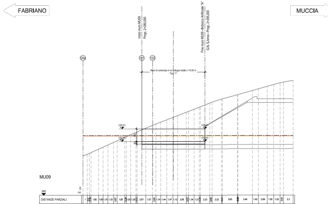
Figura 2.1 - Profilo longitudinale opera di sottoscarpa MU12
