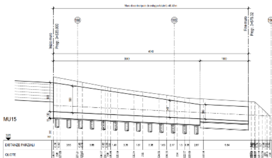
Figura 2.1 - Profilo longitudinale opera di sottoscarpa MU15
