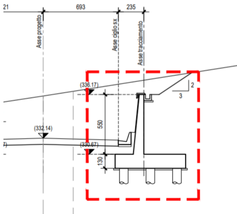
Figura 2.2 – Sezione opera di controripa di tipo 2, Hparam=6m
