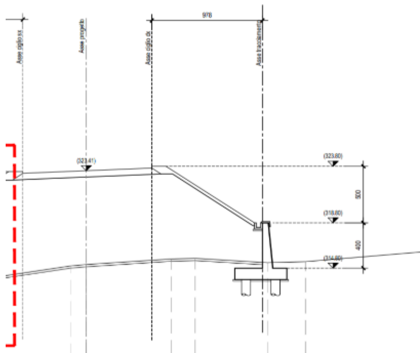
Figura 2.3 – Sezione opera di sottoscarpa di tipo 2, Hparam=4 m
