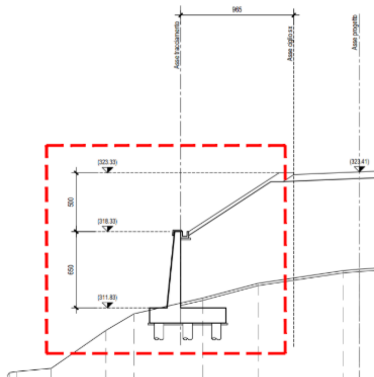
Figura 2.2 – Sezione opera di sottoscarpa di tipo 3, Hparam=6.5m
