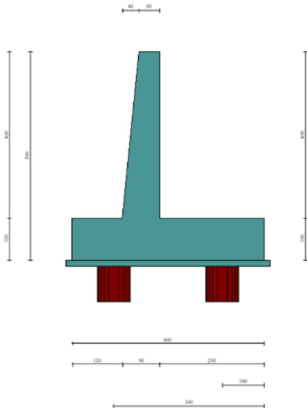
Geometria muro
