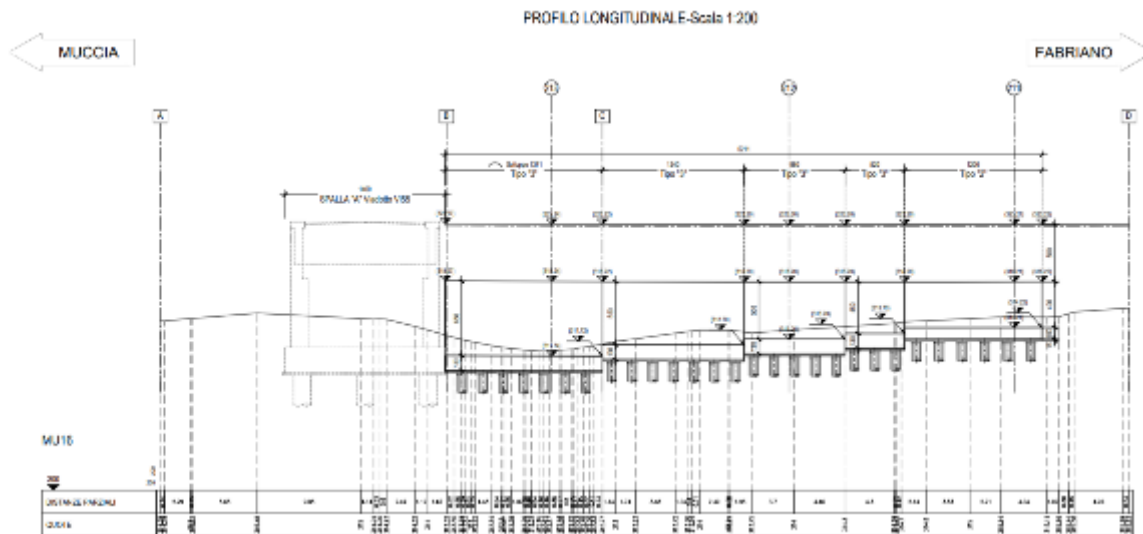
Figura 2.1 - Profilo longitudinale opera di sottoscarpa MU16
