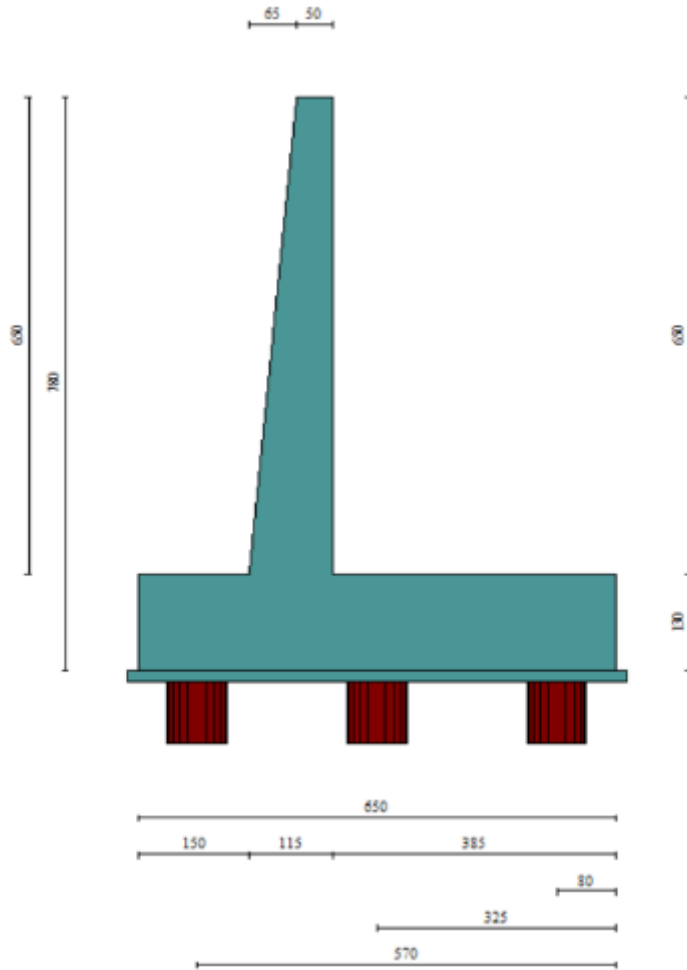
Geometria muro
