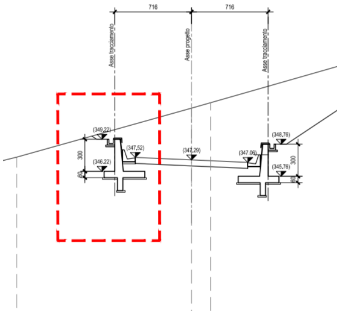
Figura 2.2 – Sezione opera di controripa di tipo 1, Hparam=3.0m
