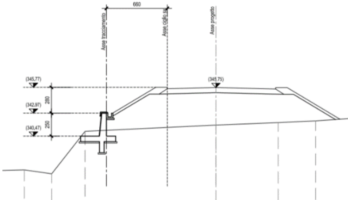
Figura 2.2 – Sezione opera di sottoscarpa di tipo 1, Hparam=3.0m
