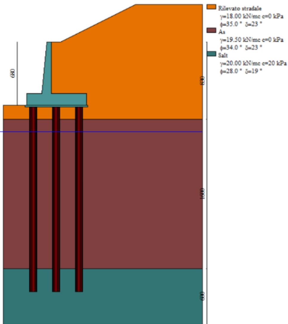
Modello di calcolo muro su PALI
