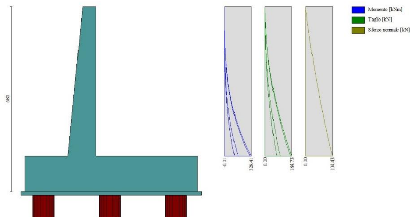
Fig. 6 - Paramento
