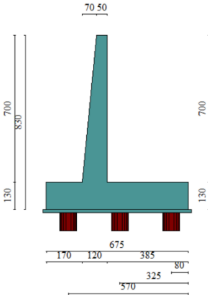
Geometria muro
