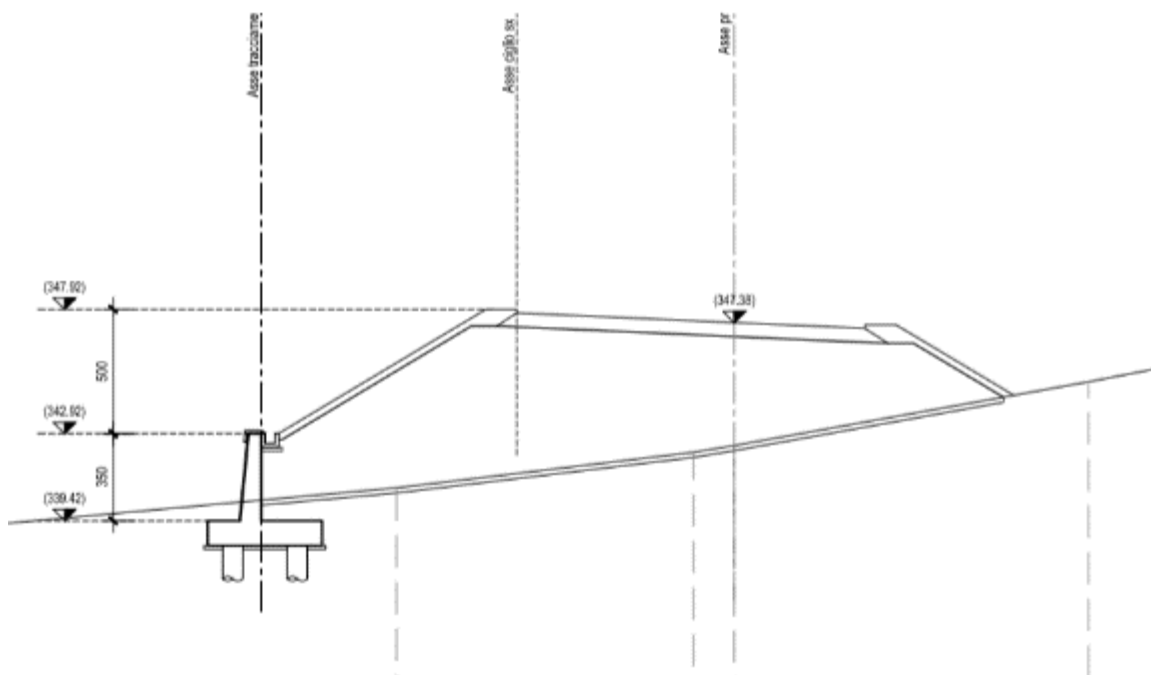
Figura 2.3 – Sezione opera di controripa di tipo 2, Hparam=3.5m
