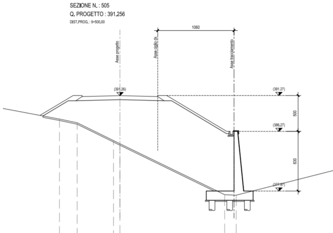
Figura 2.3 – Sezione opera di sottoscarpa di tipo 3, Hparam=8.3 m
