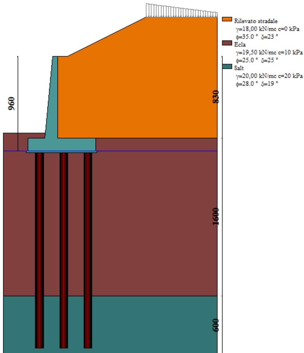
Modello di calcolo muro su PALI
