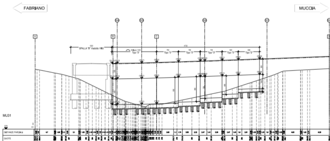
Figura 2.1 - Profilo longitudinale opera di sottoscarpa MU31
