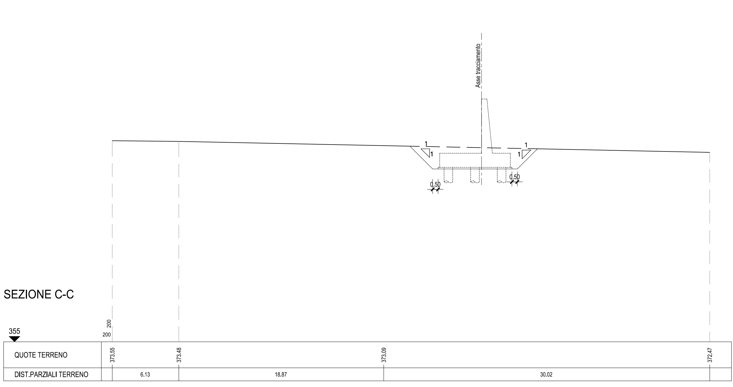
SEZIONE C-C - Scala 1:200
