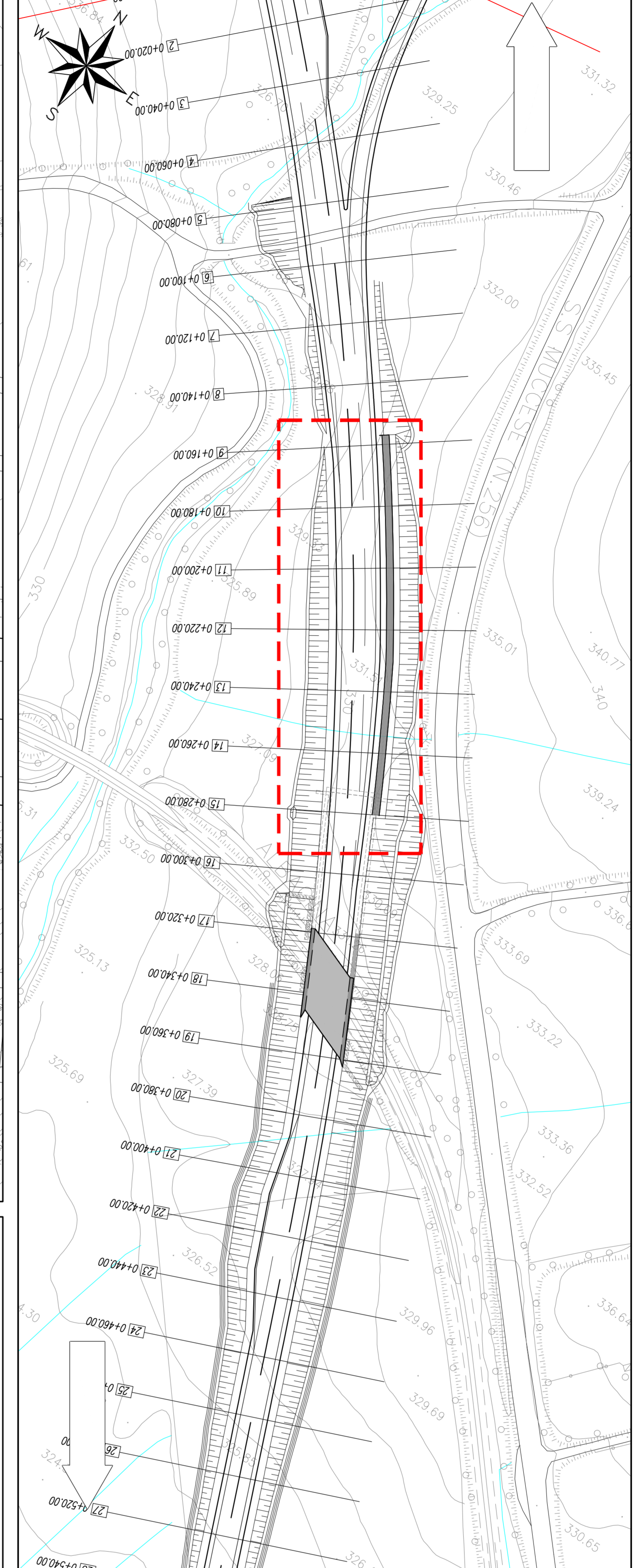
PLANIMETRIA-Scala 1:1000
