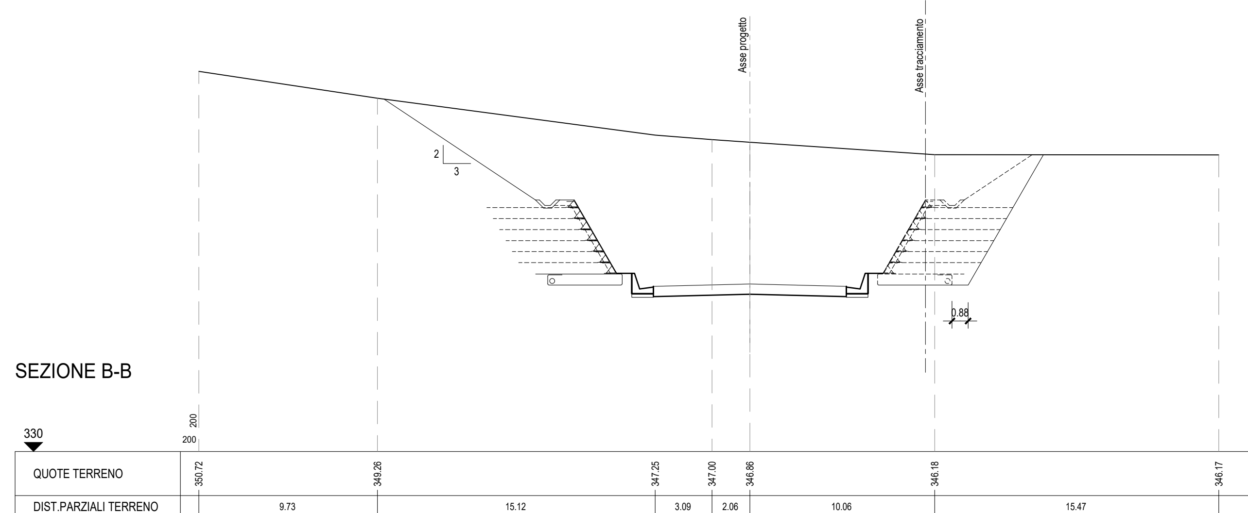
SEZIONE B-B - Scala 1:200
