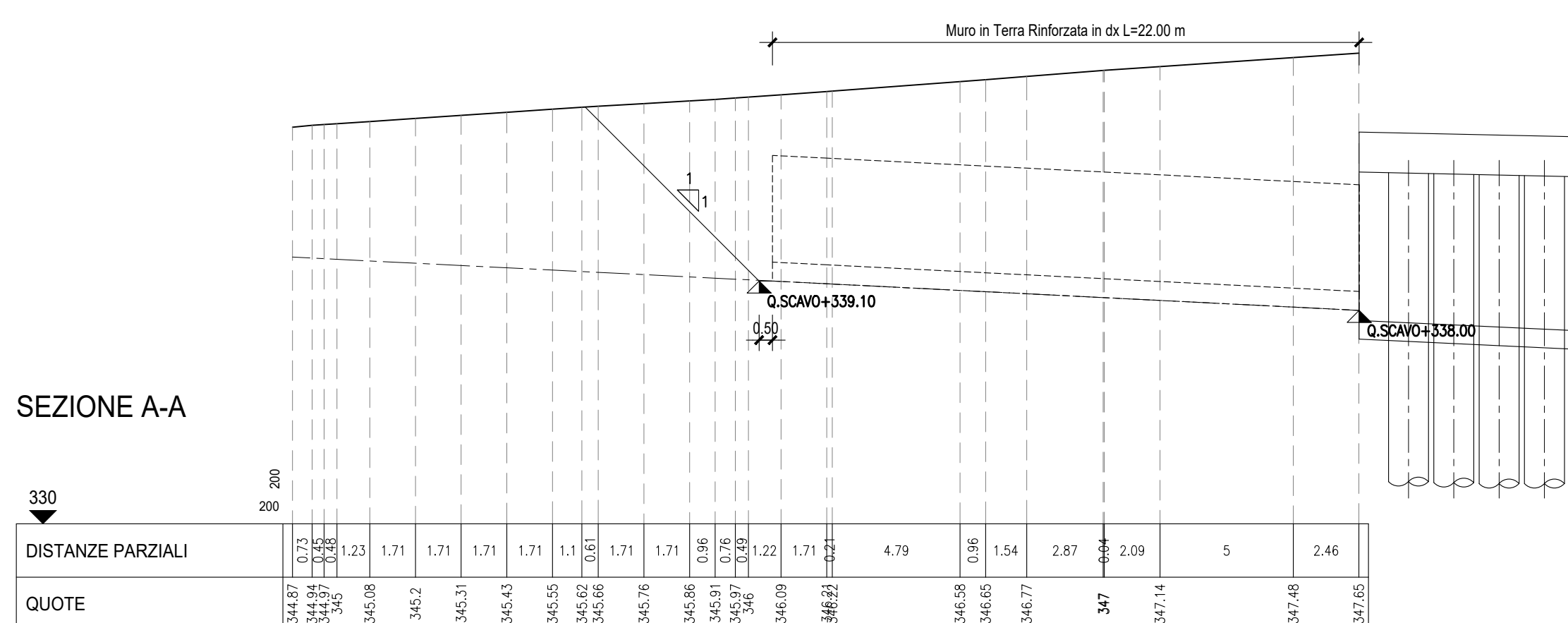
SEZIONE A-A - Scala 1:200
