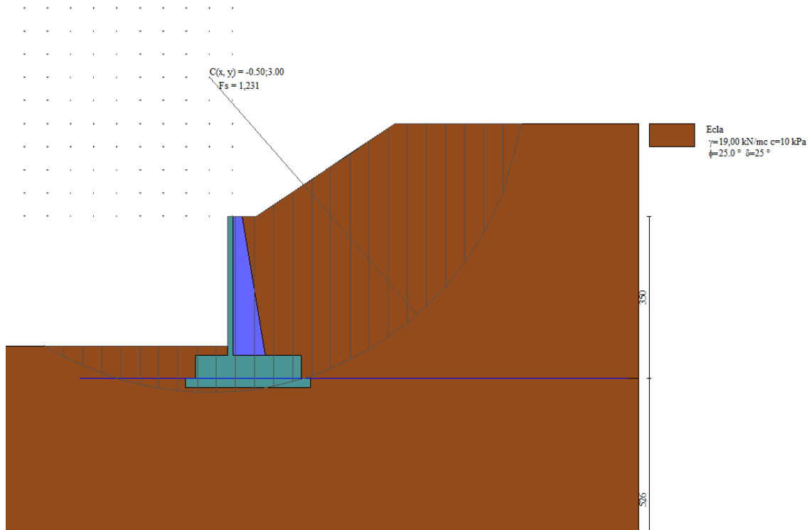
Figura 20 - Verifica di stabilità globale dei MURI DI CONTRORIPA - FONDAZIONE DIRETTA - TIPO 4
