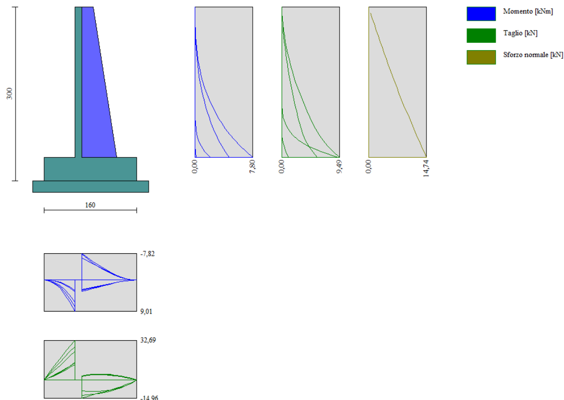
Figura 15 - Inviluppo delle sollecitazioni dei MURI DI CONTRORIPA - FONDAZIONE DIRETTA - TIPO 3
