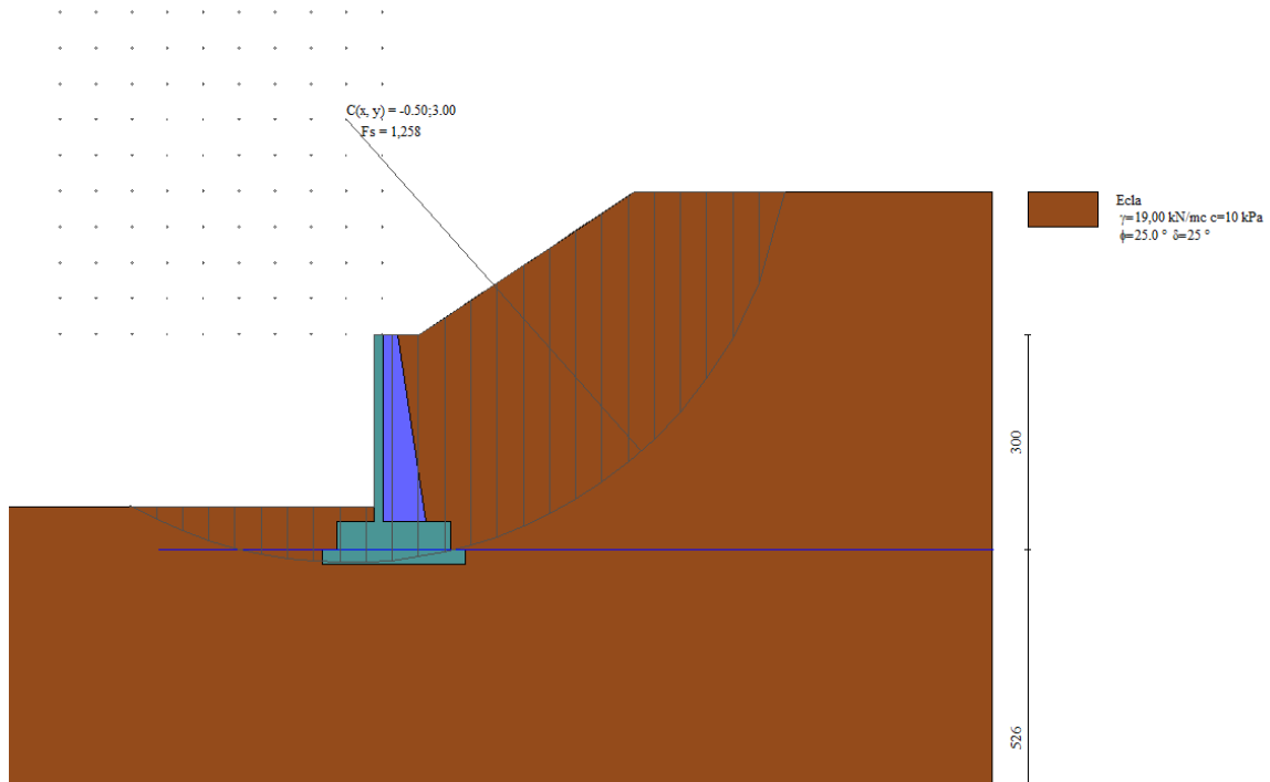
Figura 16 - Verifica di stabilità globale dei MURI DI CONTRORIPA - FONDAZIONE DIRETTA - TIPO 3
