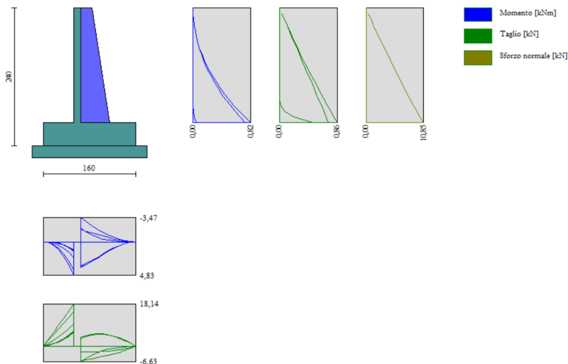
Figura 7 - Involuppo delle sollecitazioni dei MURI DI CONTRORIPA - FONDAZIONE DIRETTA - TIPO 1
