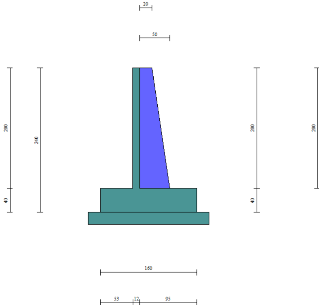
Figura 6 - Geometria dei MURI DI CONTRORIPA - FONDAZIONE DIRETTA - TIPO 1
