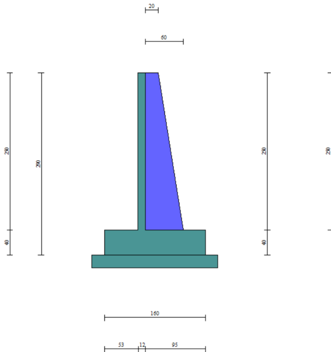
Figura 10 - Geometria dei MURI DI CONTRORIPA - FONDAZIONE DIRETTA - TIPO 2
