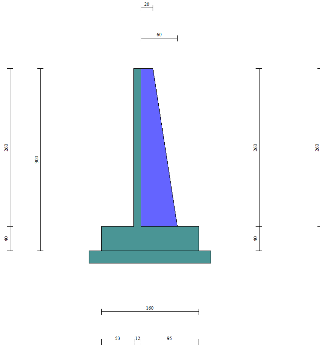
Figura 14 - Geometria dei MURI DI CONTRORIPA - FONDAZIONE DIRETTA - TIPO 3
