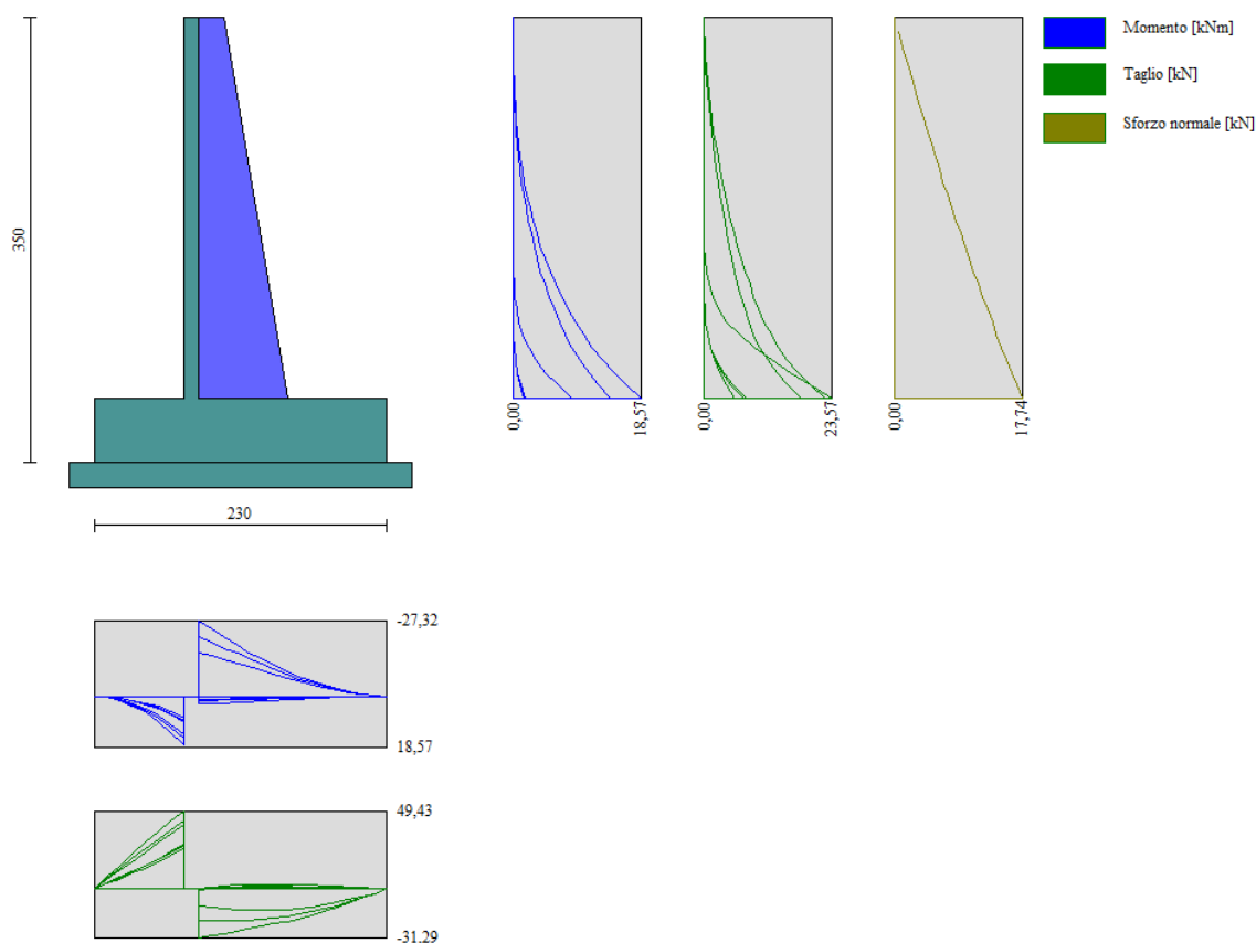
Figura 19 - Involuppo delle sollecitazioni dei MURI DI CONTRORIPA - FONDAZIONE DIRETTA - TIPO 4
