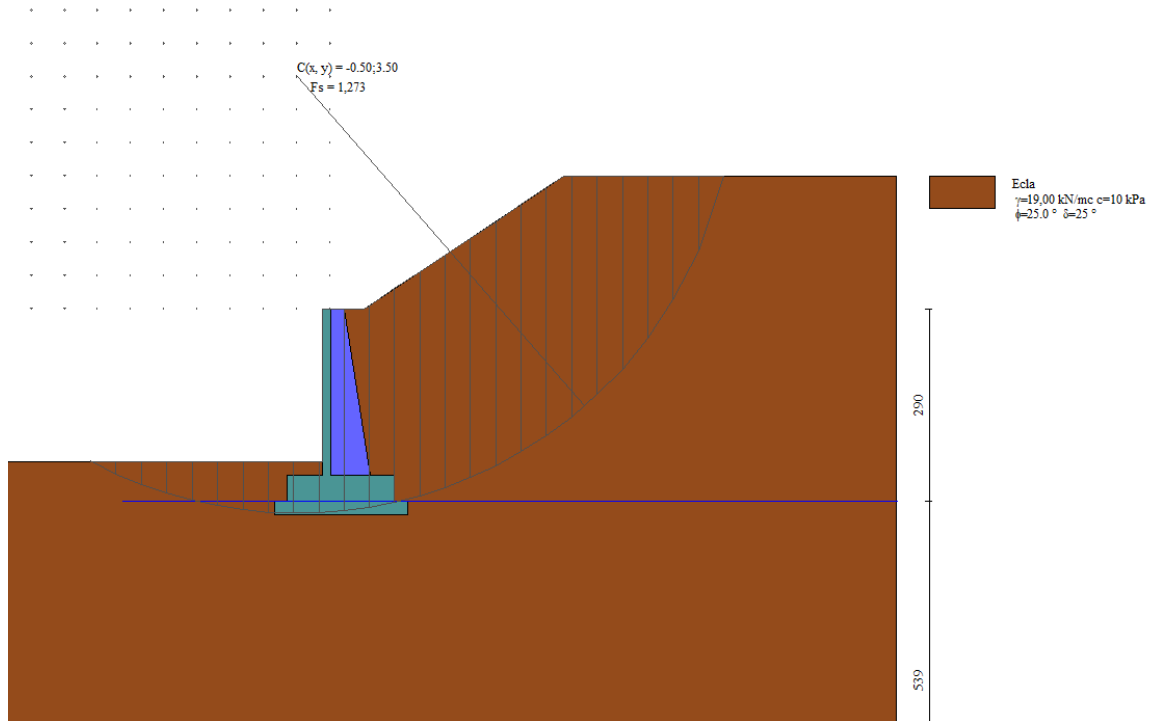
Figura 12 - Verifica di stabilità globale dei MURI DI CONTRORIPA - FONDAZIONE DIRETTA - TIPO 2
