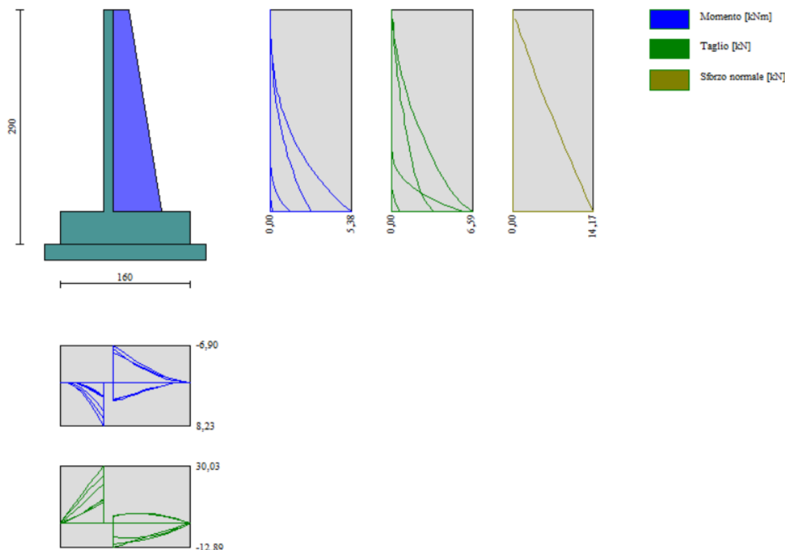
Figura 11 - Inviluppo delle sollecitazioni dei MURI DI CONTRORIPA - FONDAZIONE DIRETTA - TIPO 2
