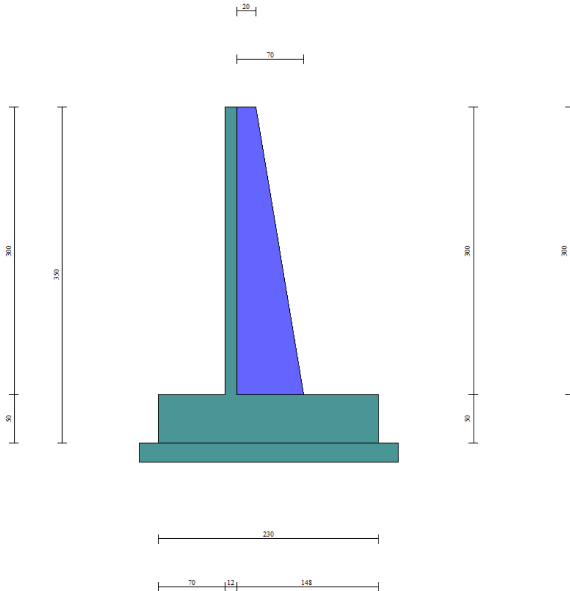
Figura 18 - Geometria dei MURI DI CONTRORIPA - FONDAZIONE DIRETTA - TIPO 4
