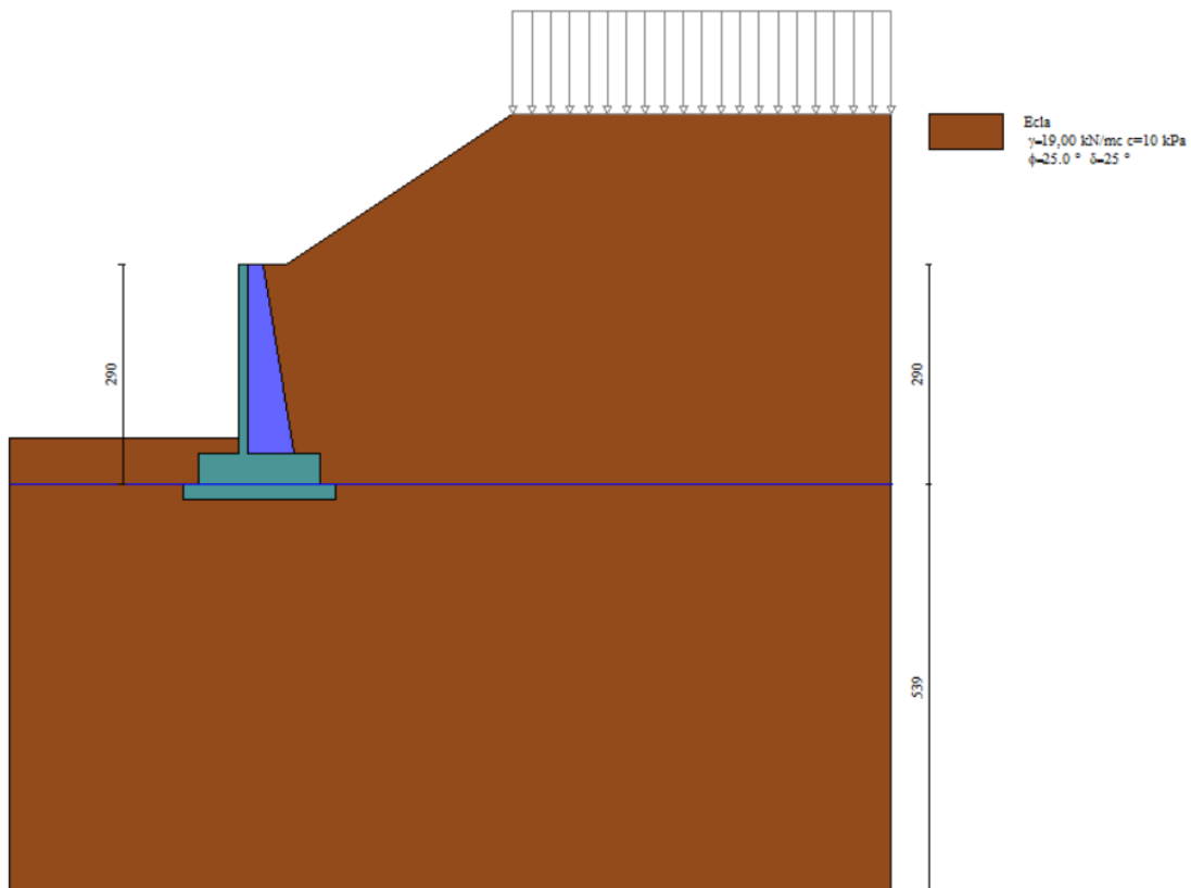
Figura 9 - Modello di calcolo dei MURI DI CONTRORIPA - FONDAZIONE DIRETTA - TIPO 2
