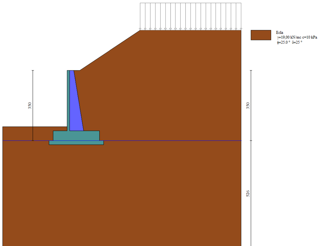
Figura 17 - Modello di calcolo dei MURI DI CONTRORIPA - FONDAZIONE DIRETTA - TIPO 4
