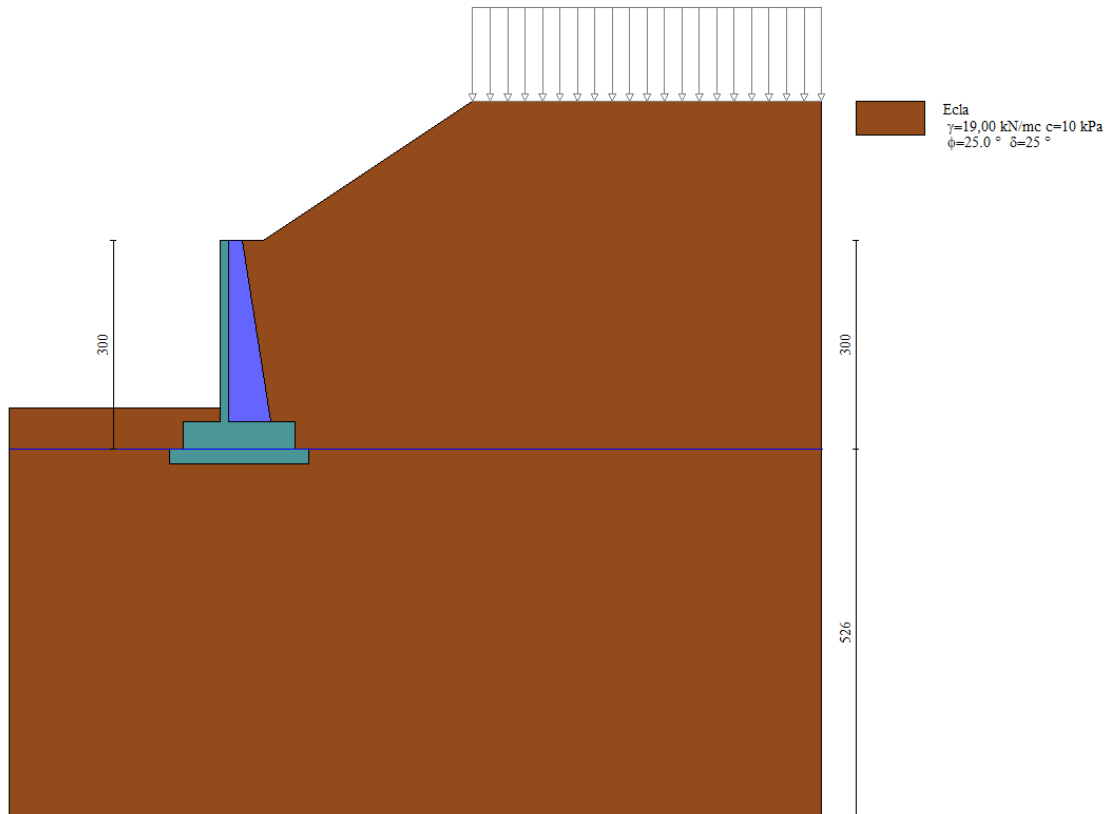
Figura 13 - Modello di calcolo dei MURI DI CONTRORIPA - FONDAZIONE DIRETTA - TIPO 3
