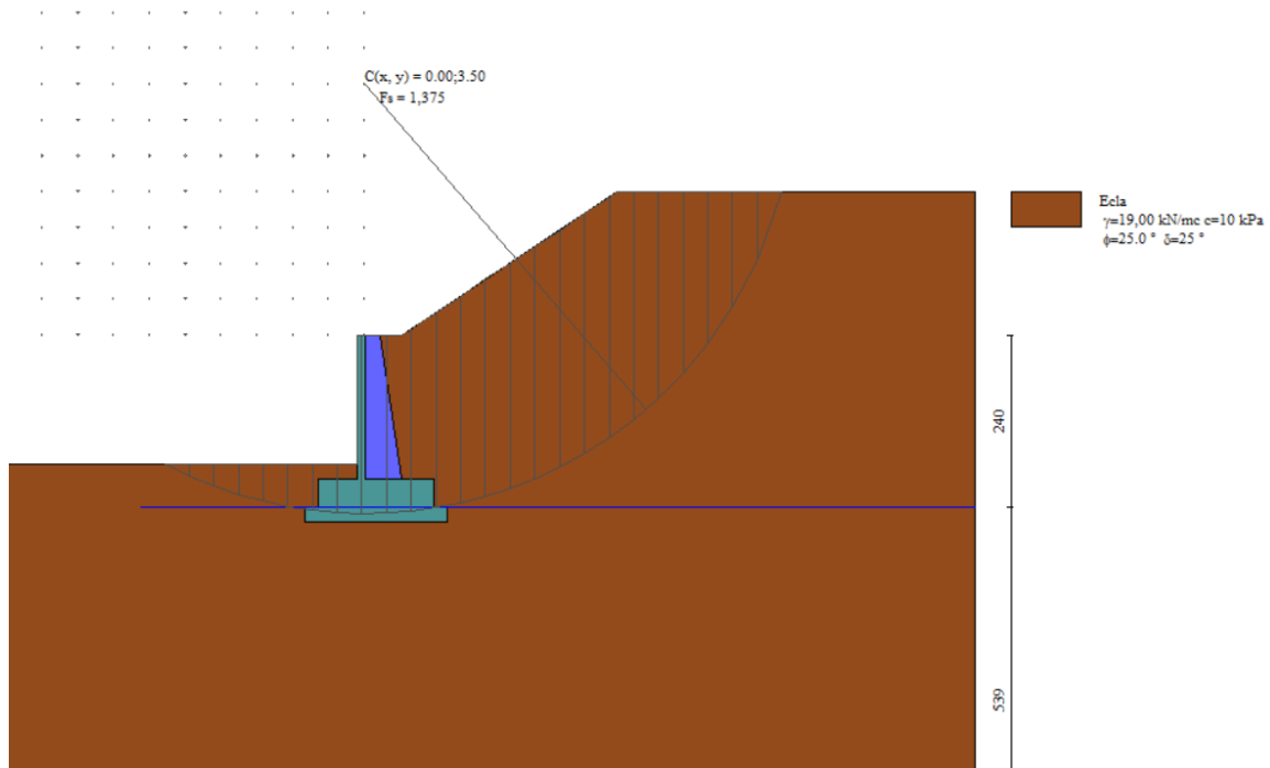
Figura 8 - Verifica di stabilità globale dei MURI DI CONTRORIPA - FONDAZIONE DIRETTA - TIPO 1
