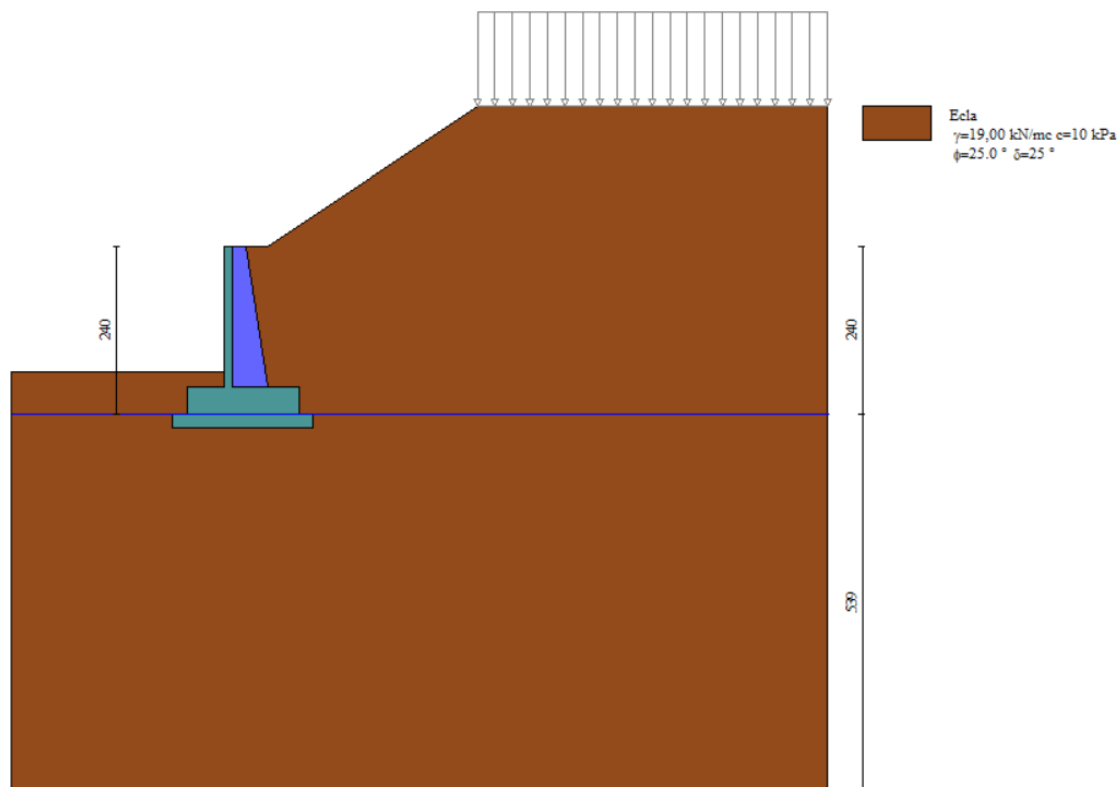
Figura 5 - Modello di calcolo dei MURI DI CONTRORIPA - FONDAZIONE DIRETTA - TIPO 1
