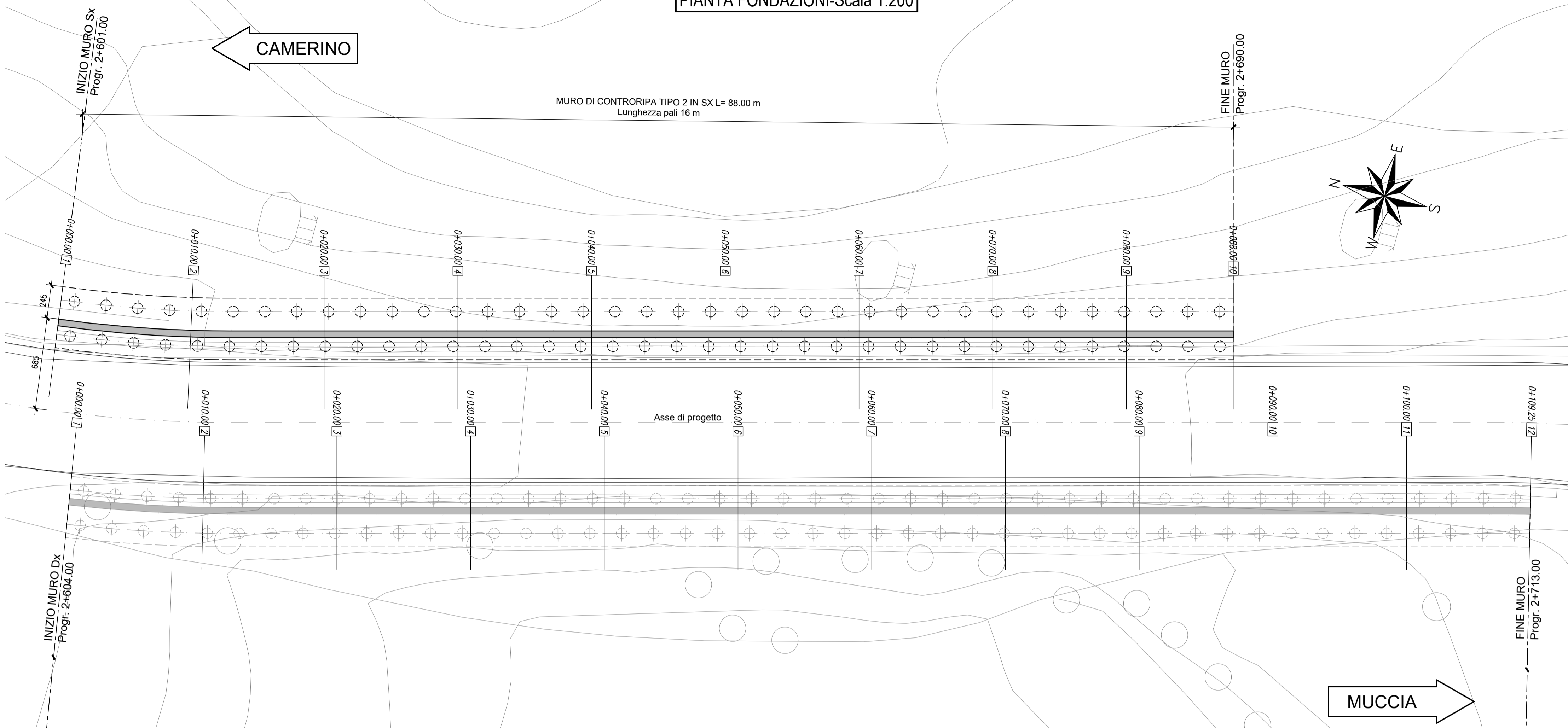
PIANTA FONDAZIONI-Scala 1:200
