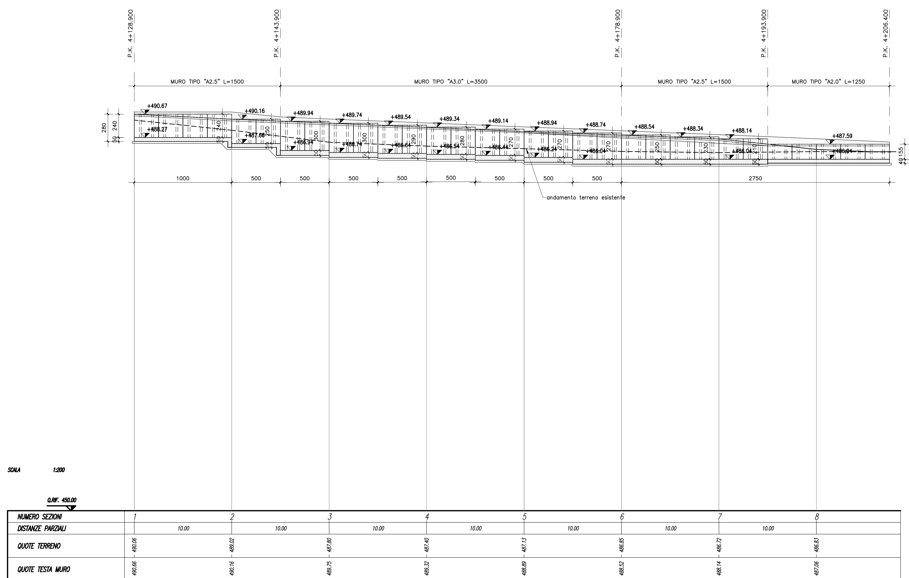
PROFILO LONGITUDINALE MURO DI SOTTOSCARPA IN SX scala 1:200
