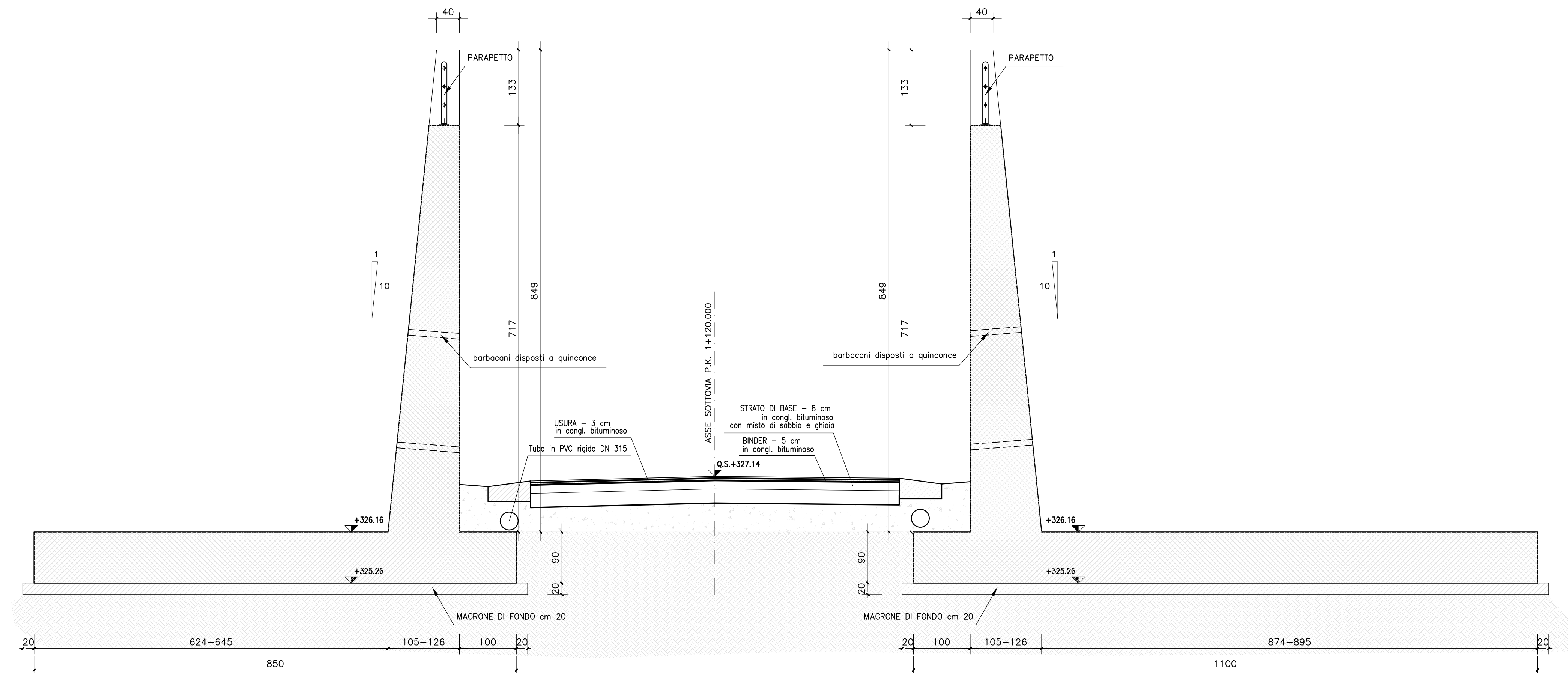
SEZIONE TRASVERSALE C-C scala 1:50
