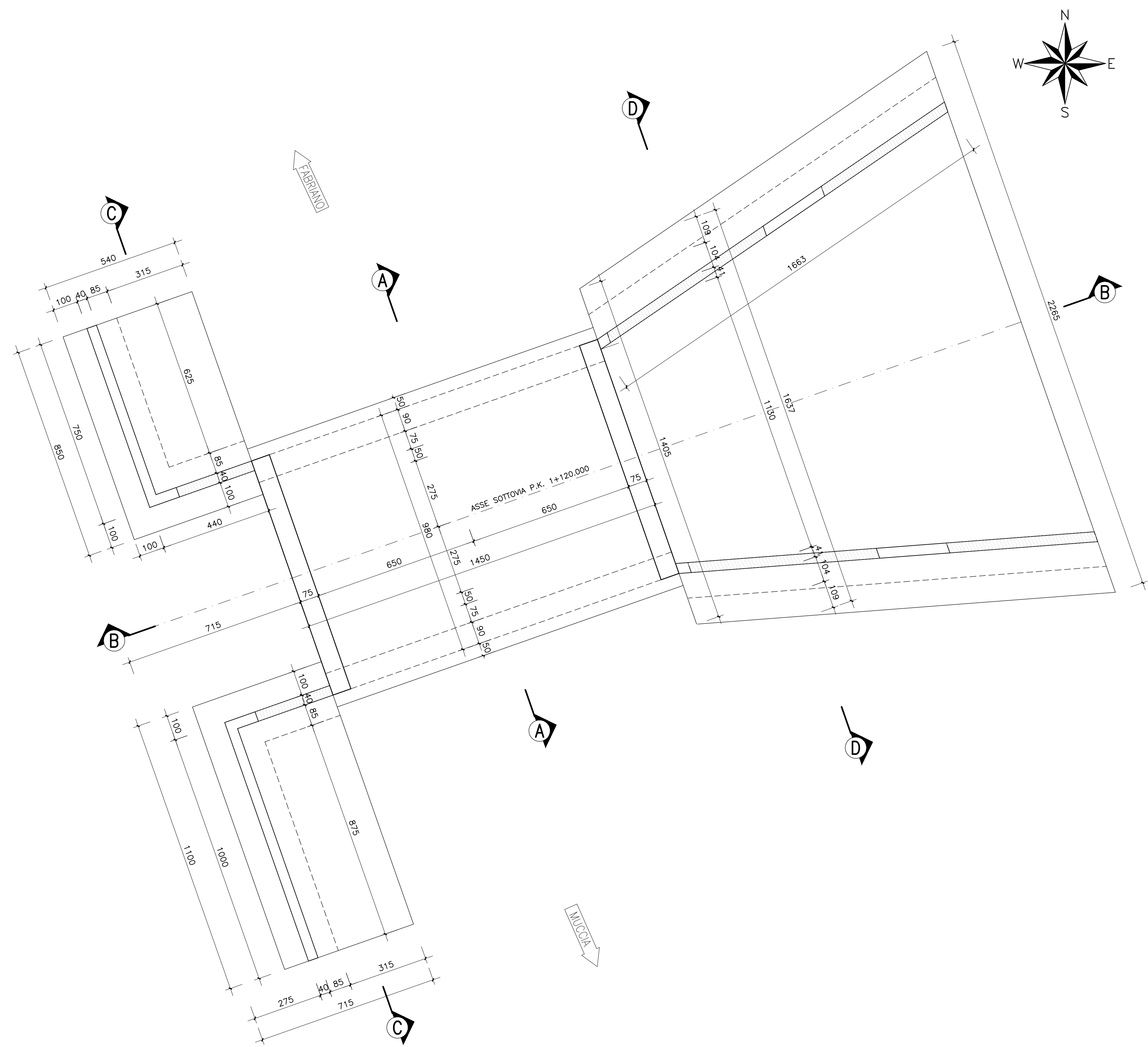
PIANTA scala 1:100
