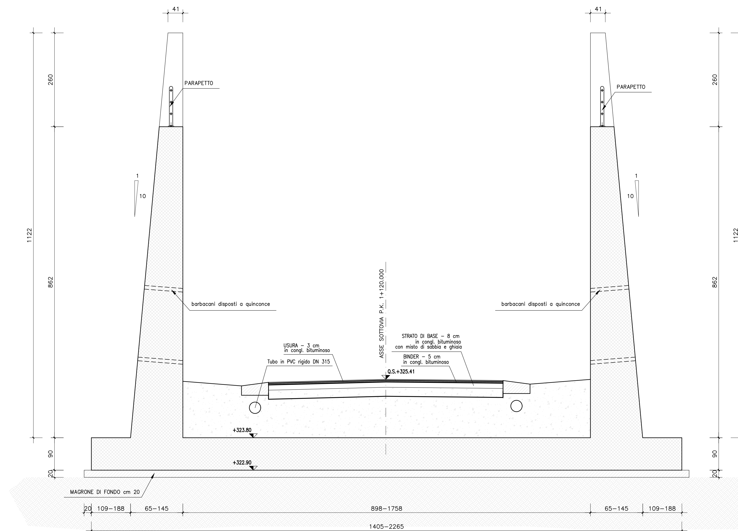
SEZIONE TRASVERSALE D-D scala 1:50
