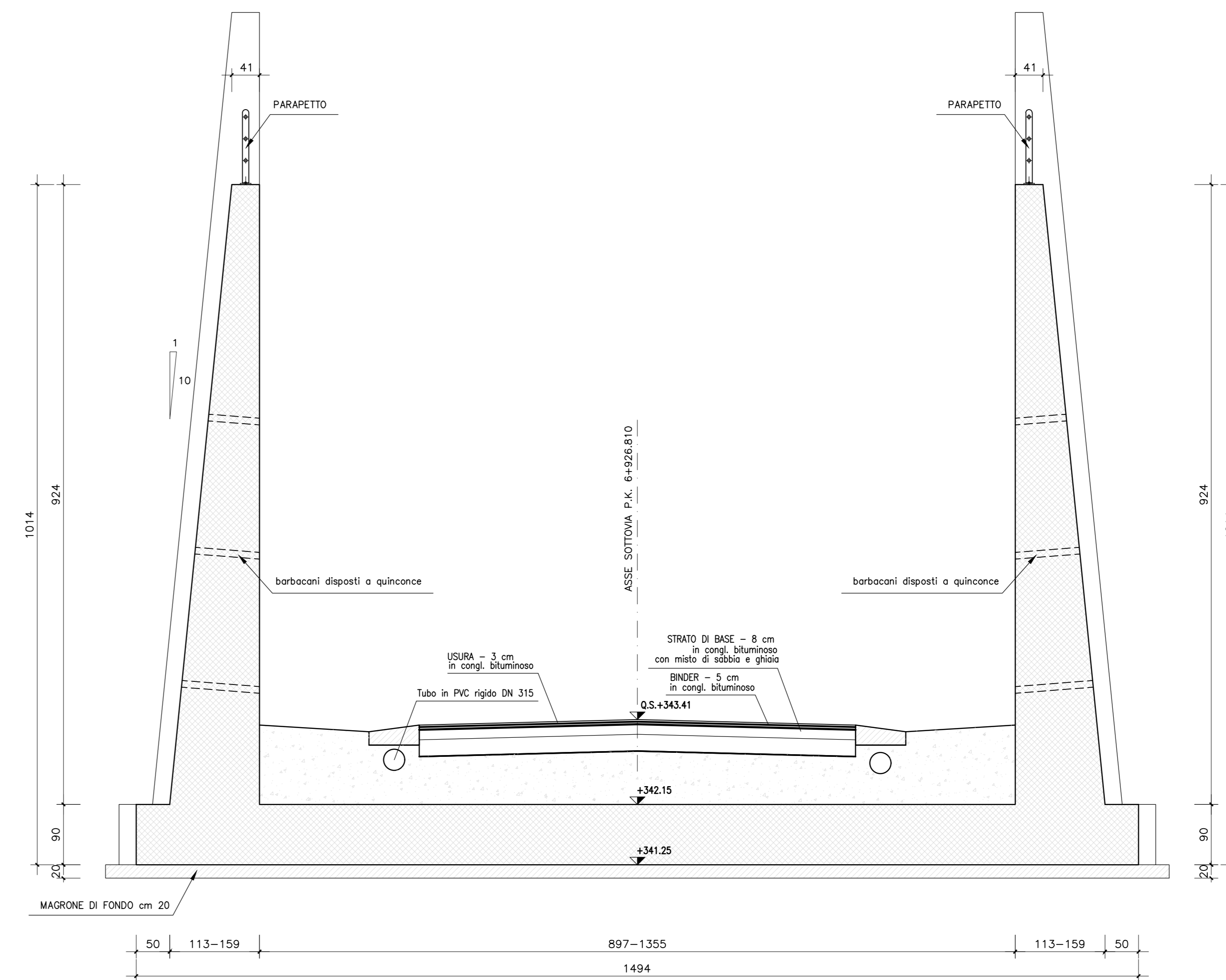
SEZIONE TRASVERSALE D-D scala 1:50
