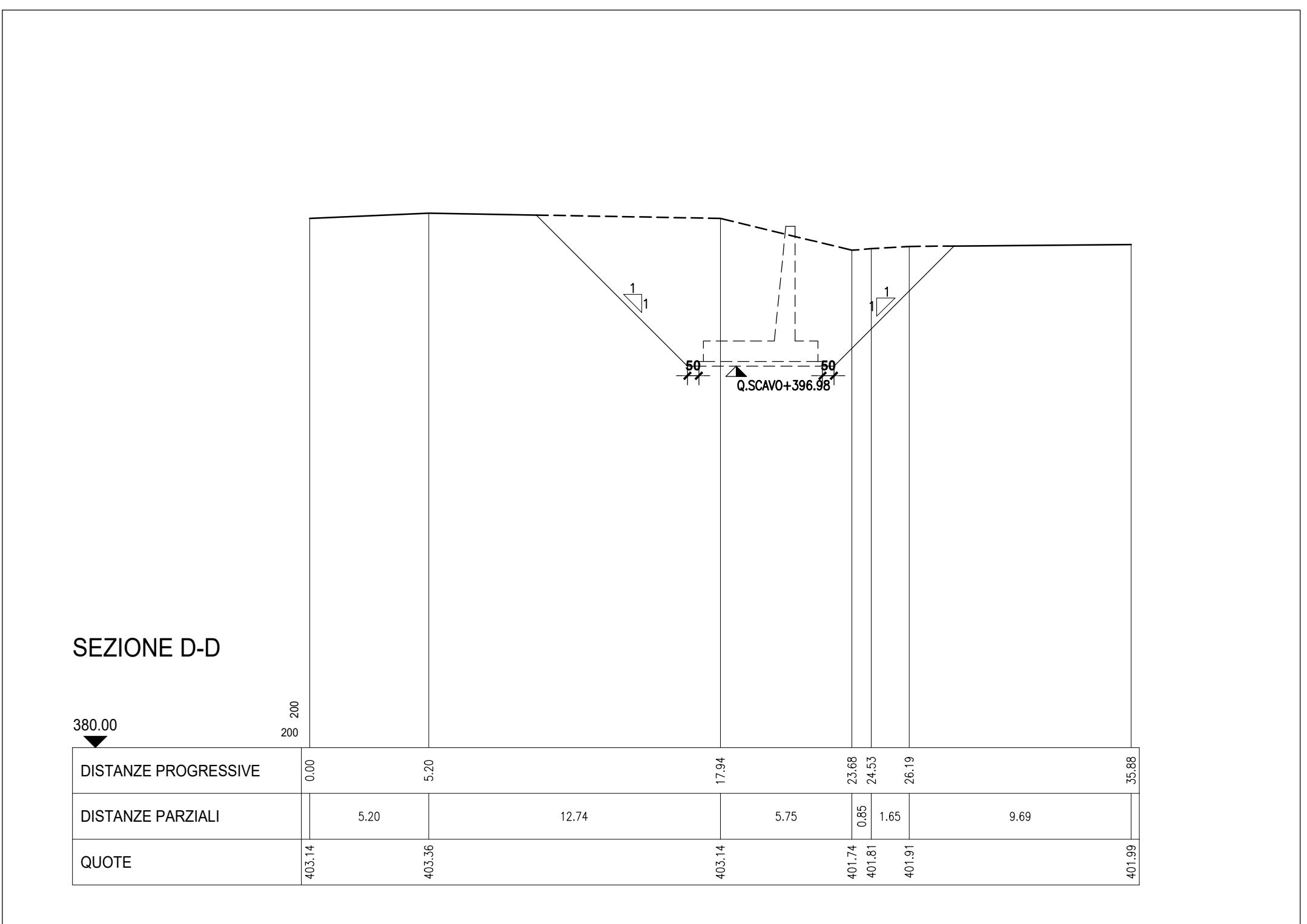
SEZIONE D-D scala 1:200
