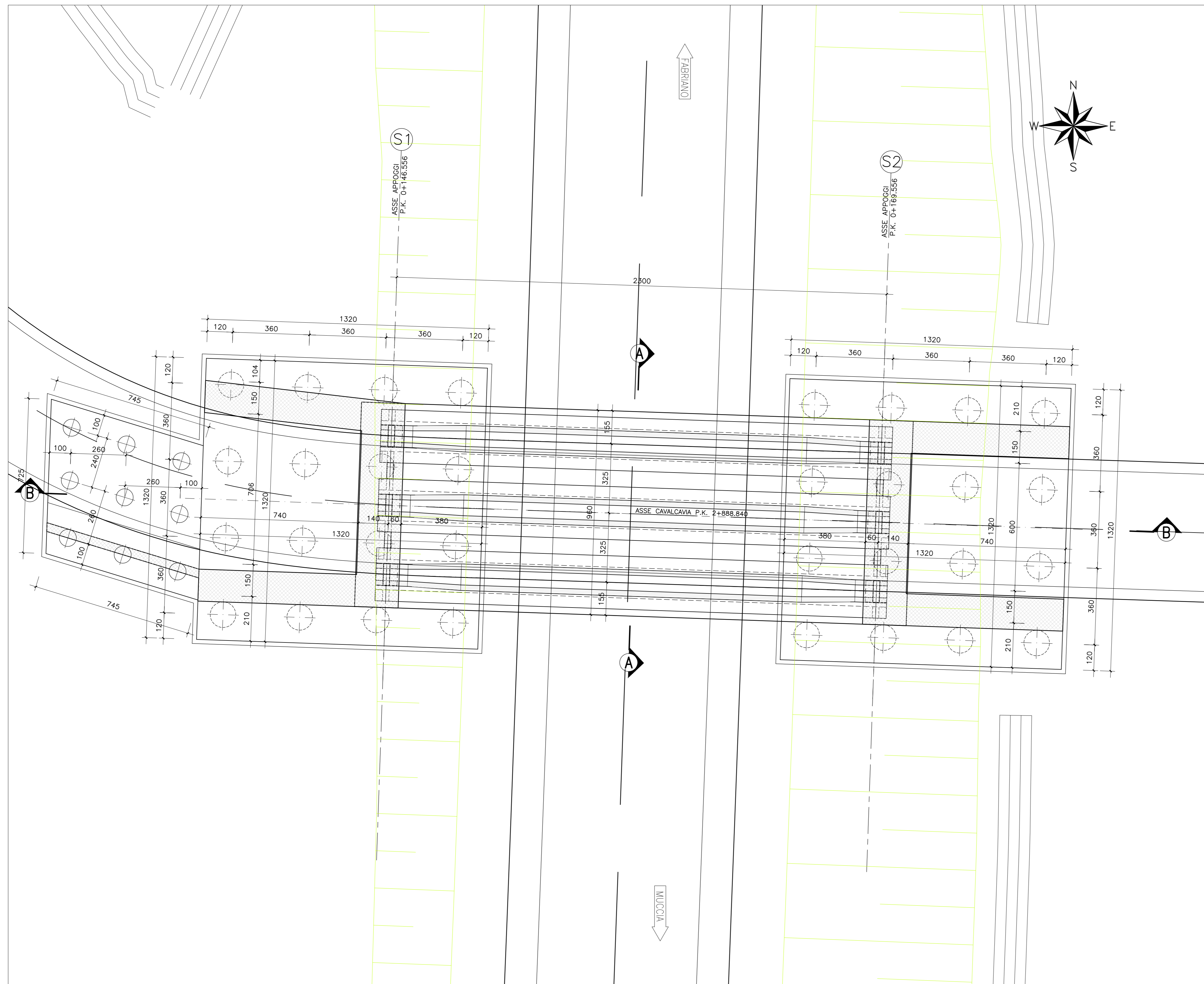
PIANTA scala 1:100
