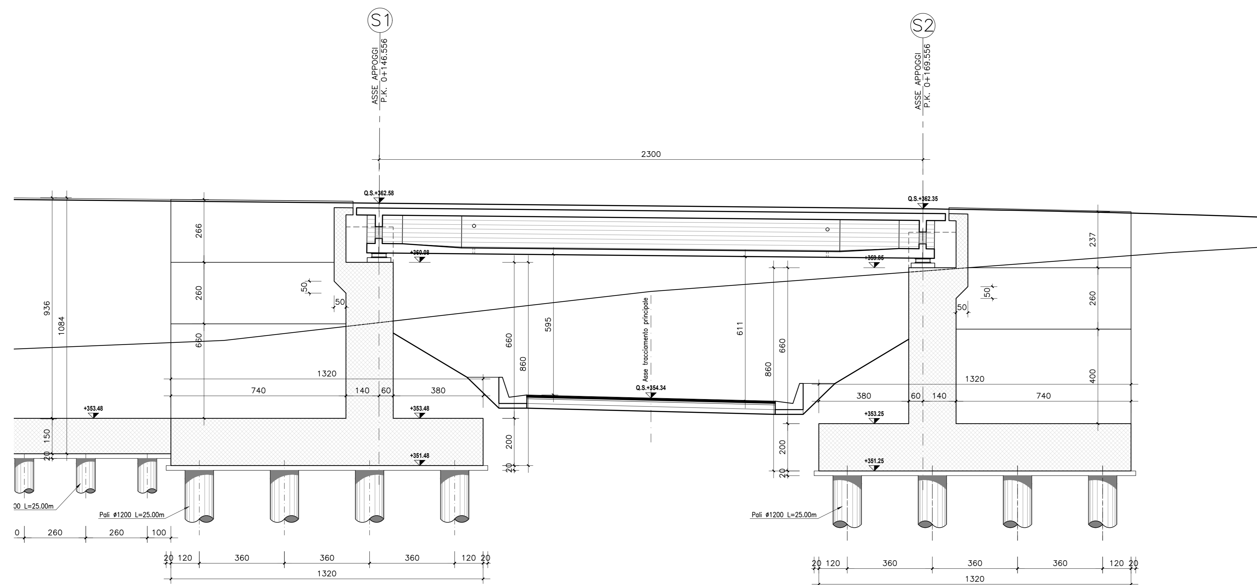
SEZIONE LONGITUDINALE B-B scala 1:100
