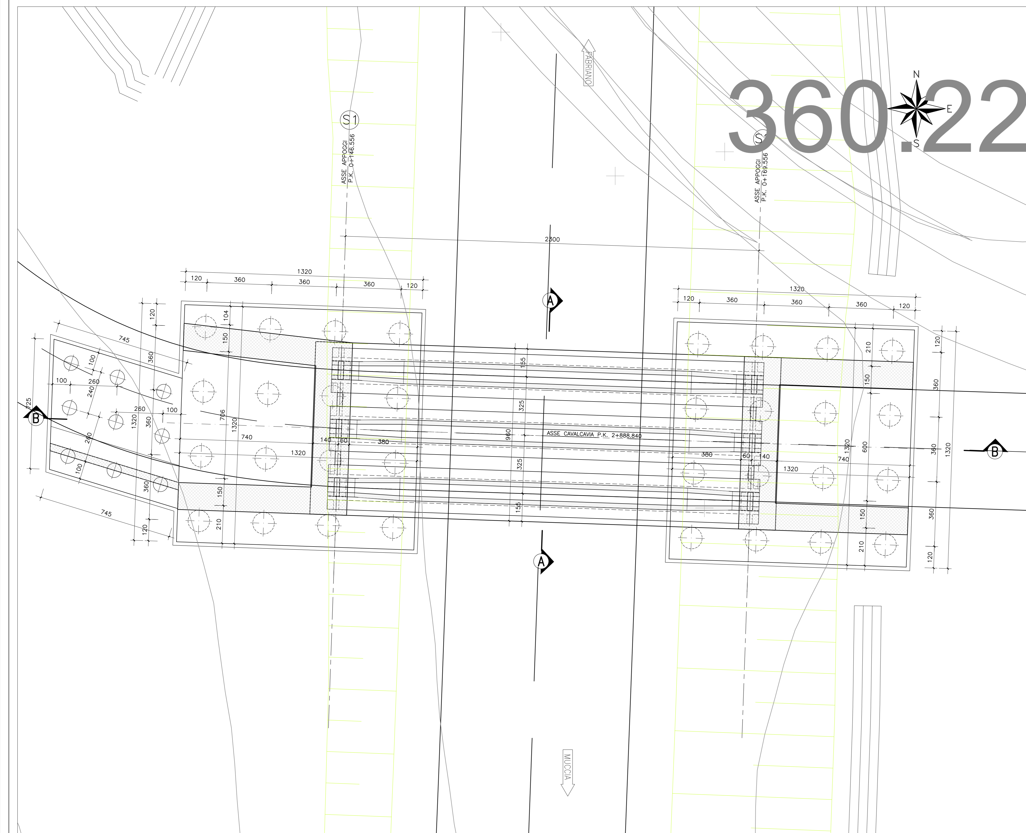
PIANTA A QUOTA PAVIMENTAZIONE scala 1:100
