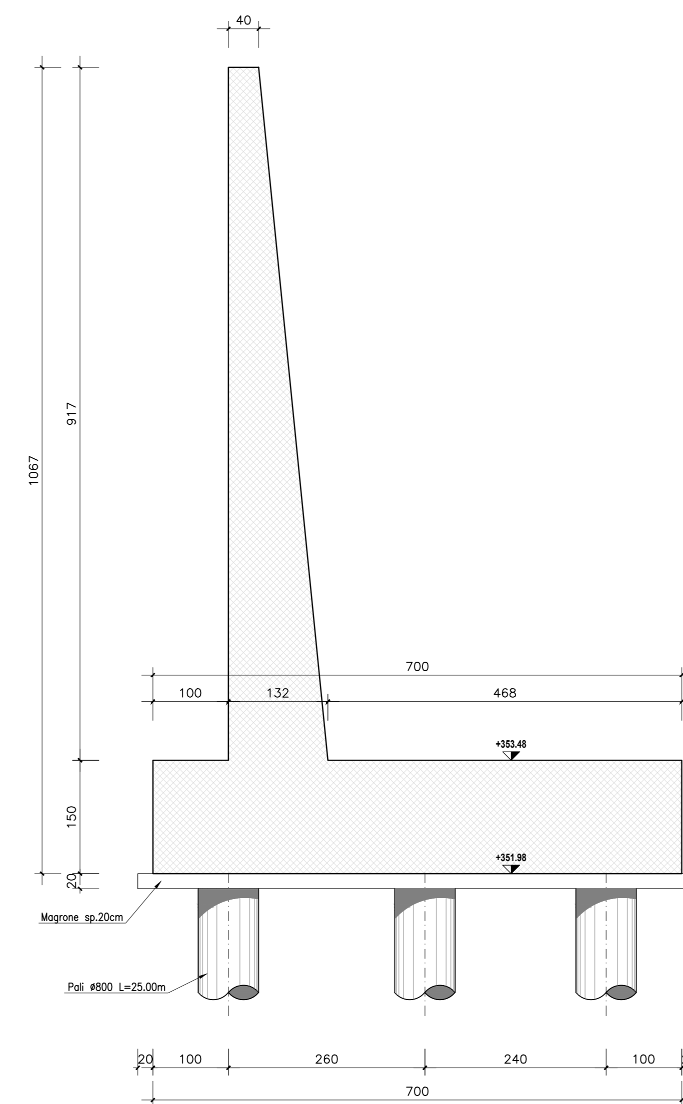
SEZIONE C-C scala 1:50
