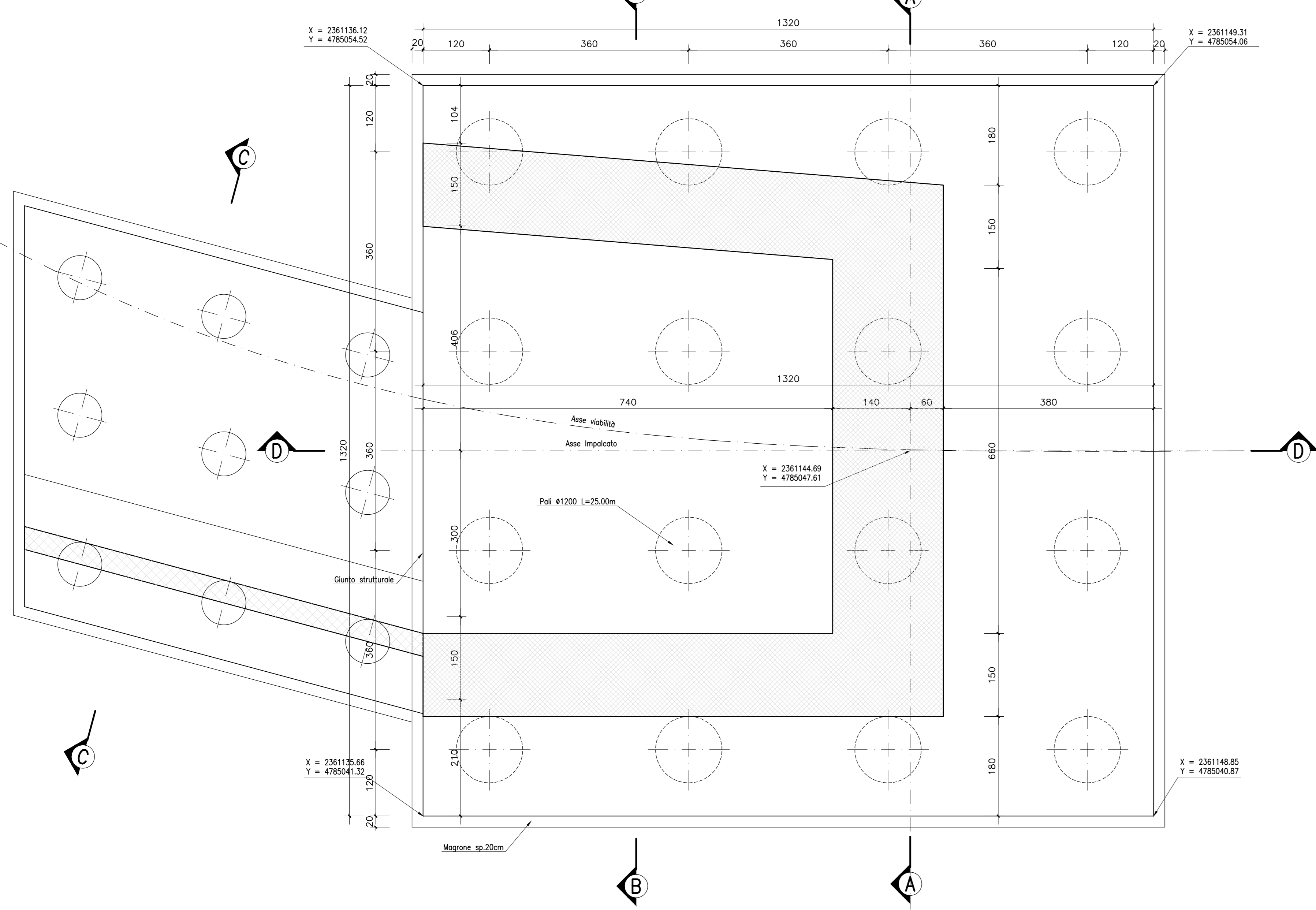
PIANTA FONDAZIONI scala 1:50
