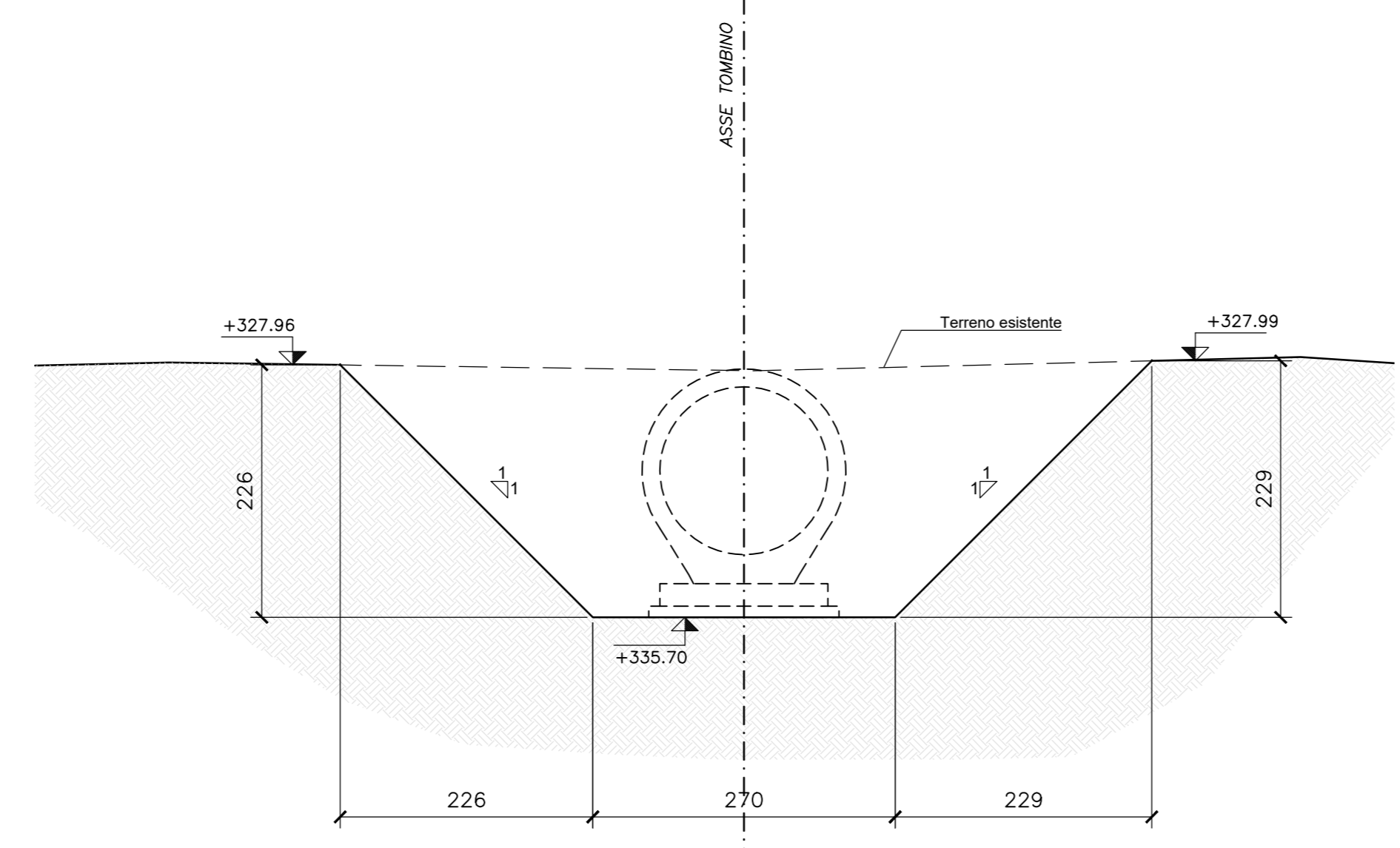
SEZIONE B-B TOMBINO Scala 1:50
