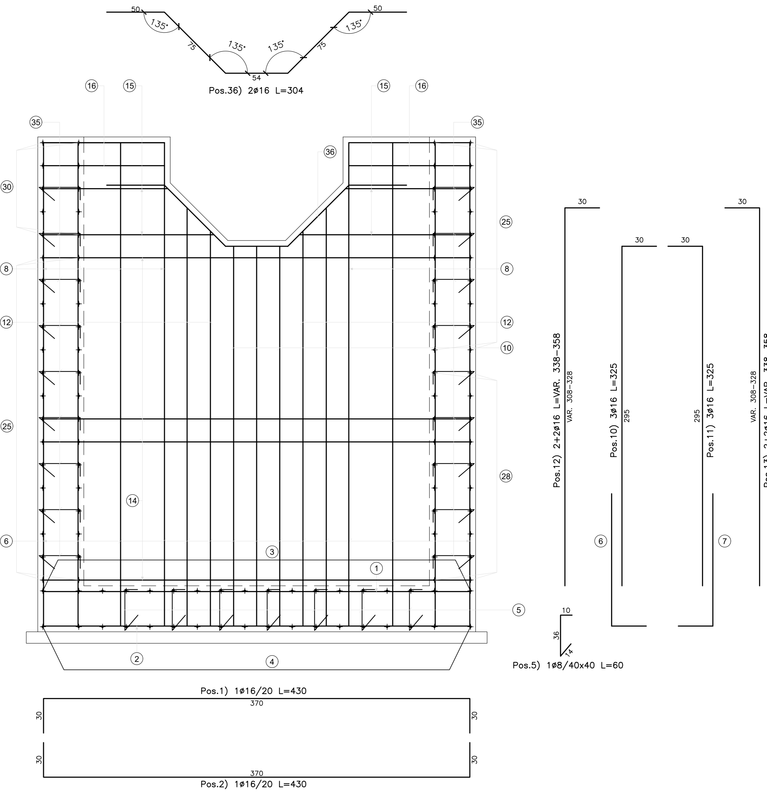
VISTA B-B Scala 1:20
