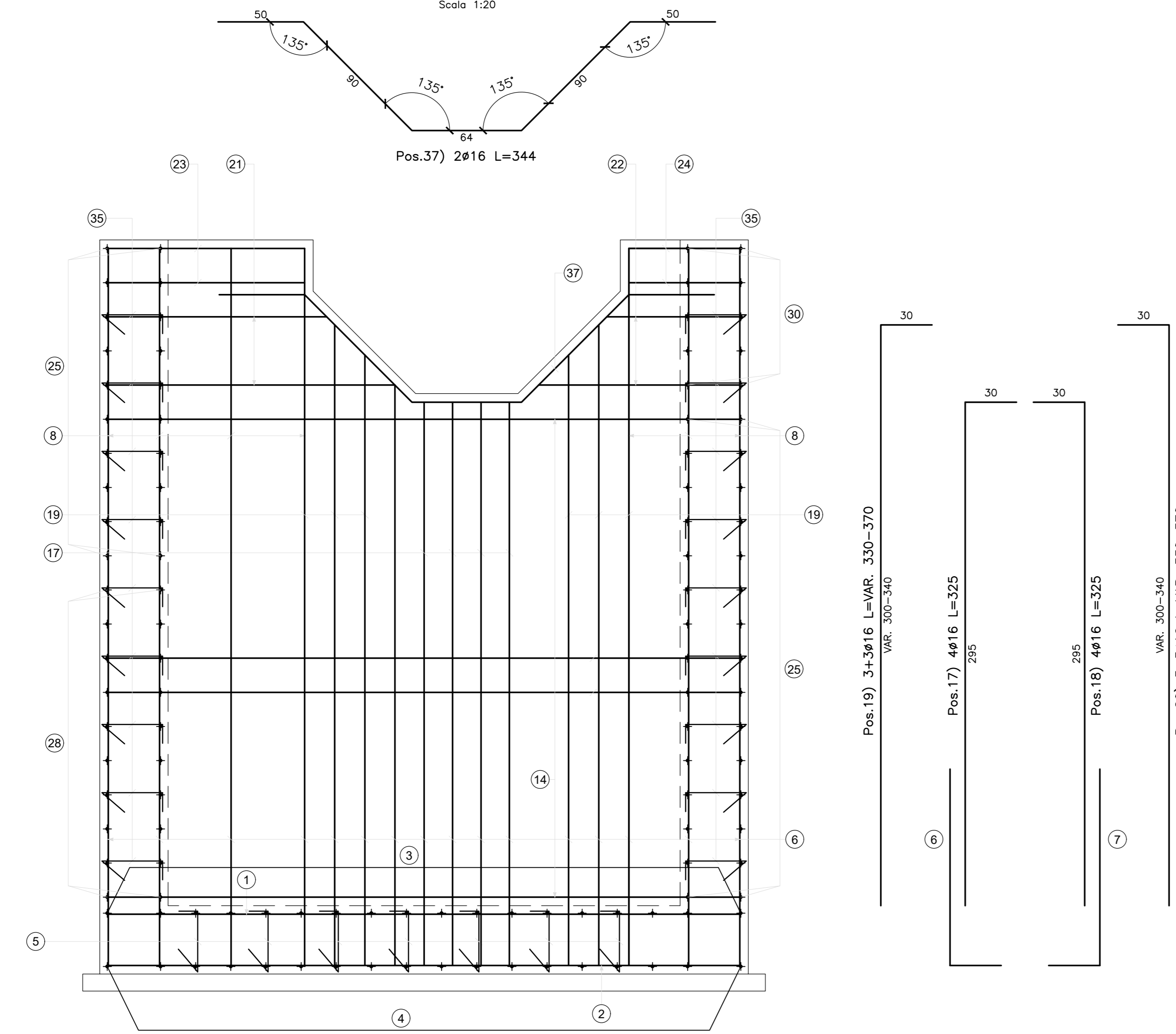
VISTA C-C Scala 1:20
