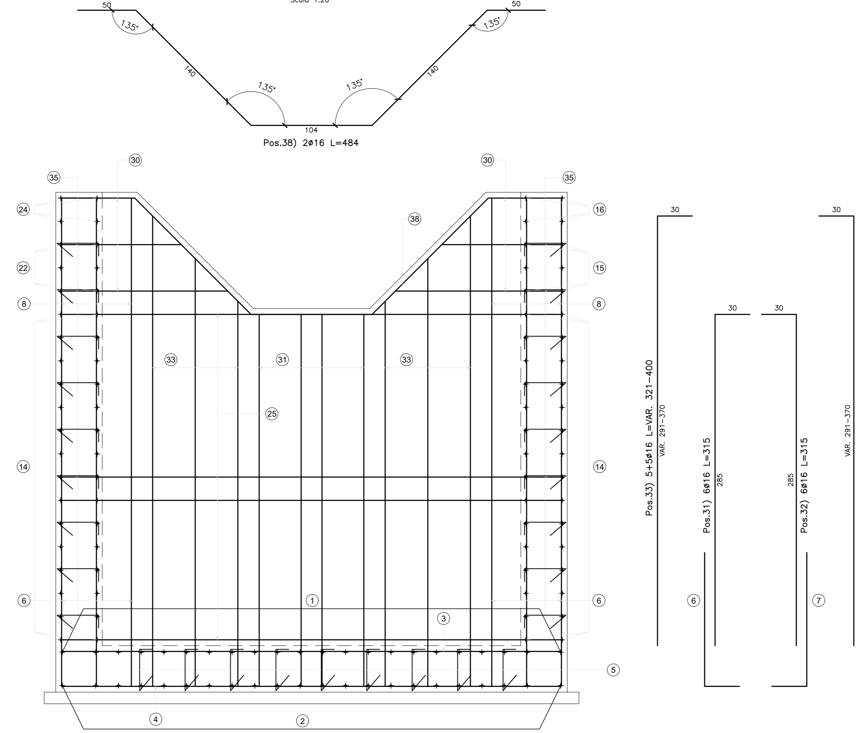
VISTA D-D Scala 1:20
