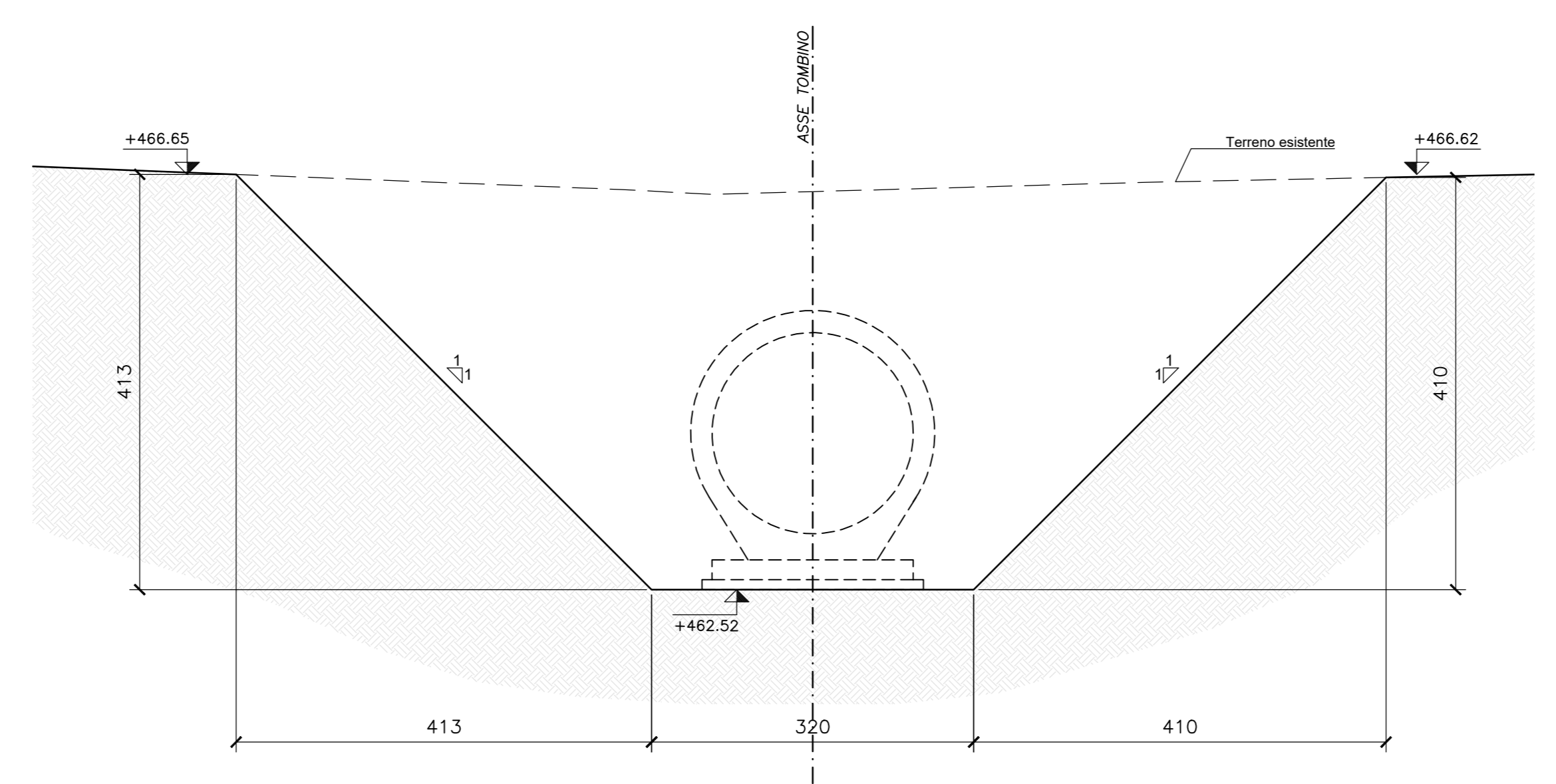
SEZIONE B-B TOMBINO Scala 1:50
