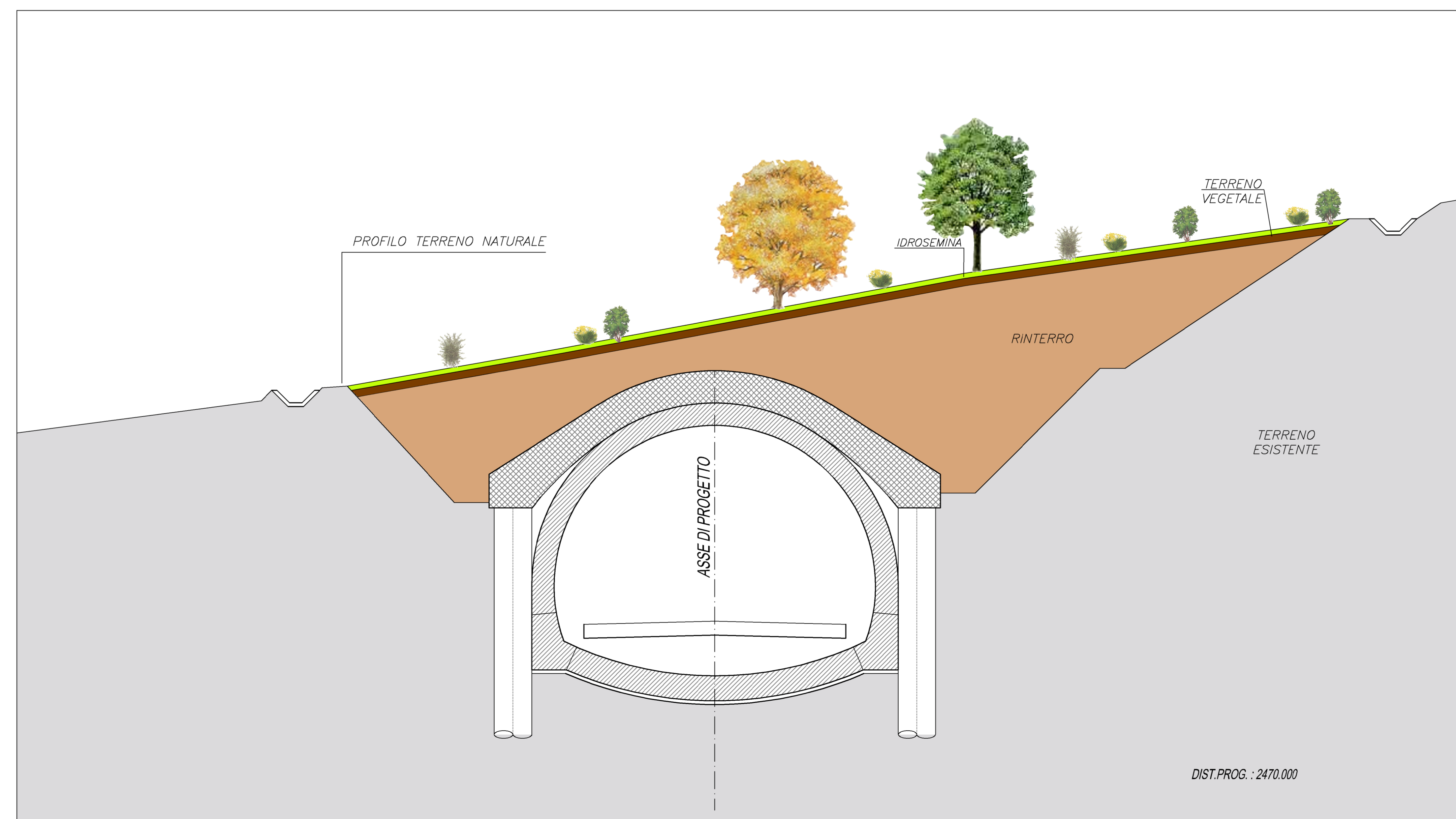
Sezione CD - Scala 1:100
