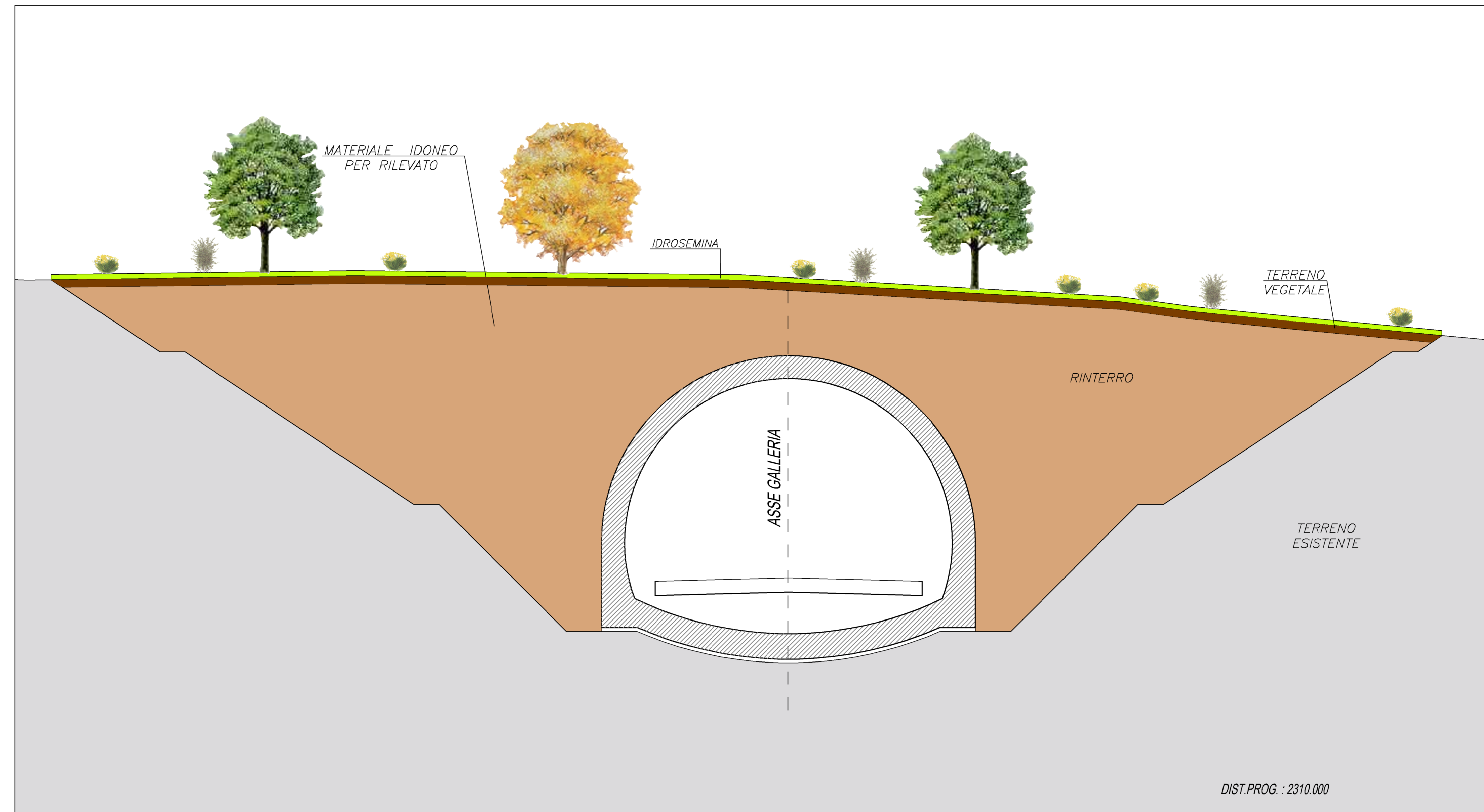
Sezione AB - Scala 1:100
