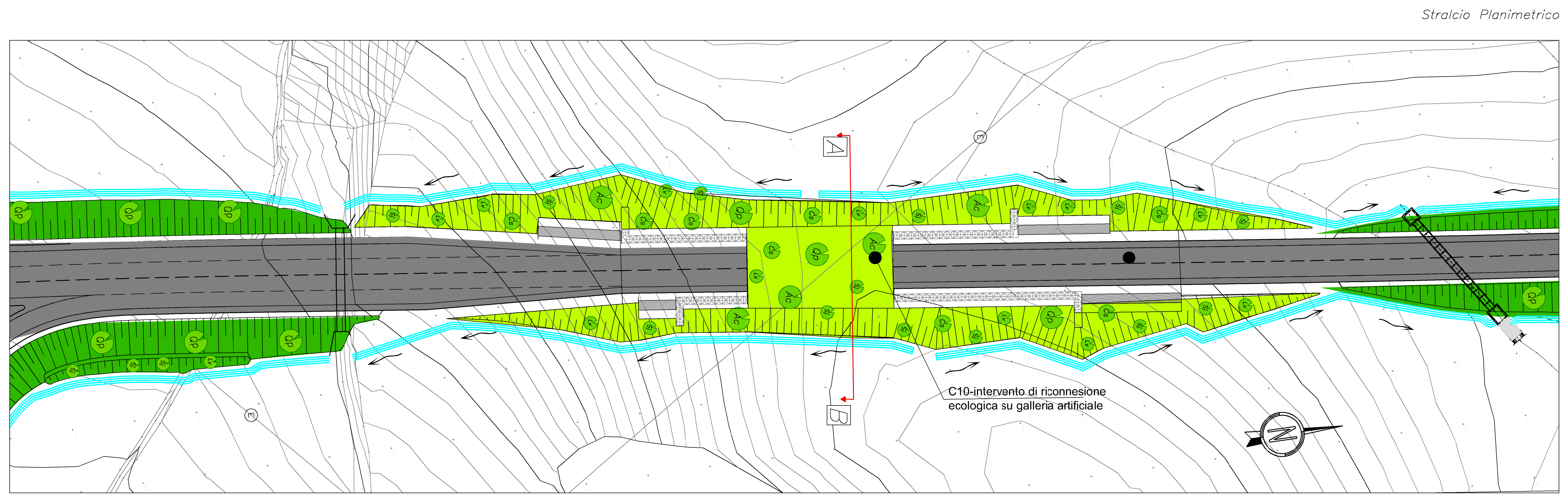
Seano - Galleria artificiale - Scala 1:500 Ambiente basso-collinare in continuità con ambiti a coltivi agrari Cespuglieti arborati a prevalenza di Acer campestre
