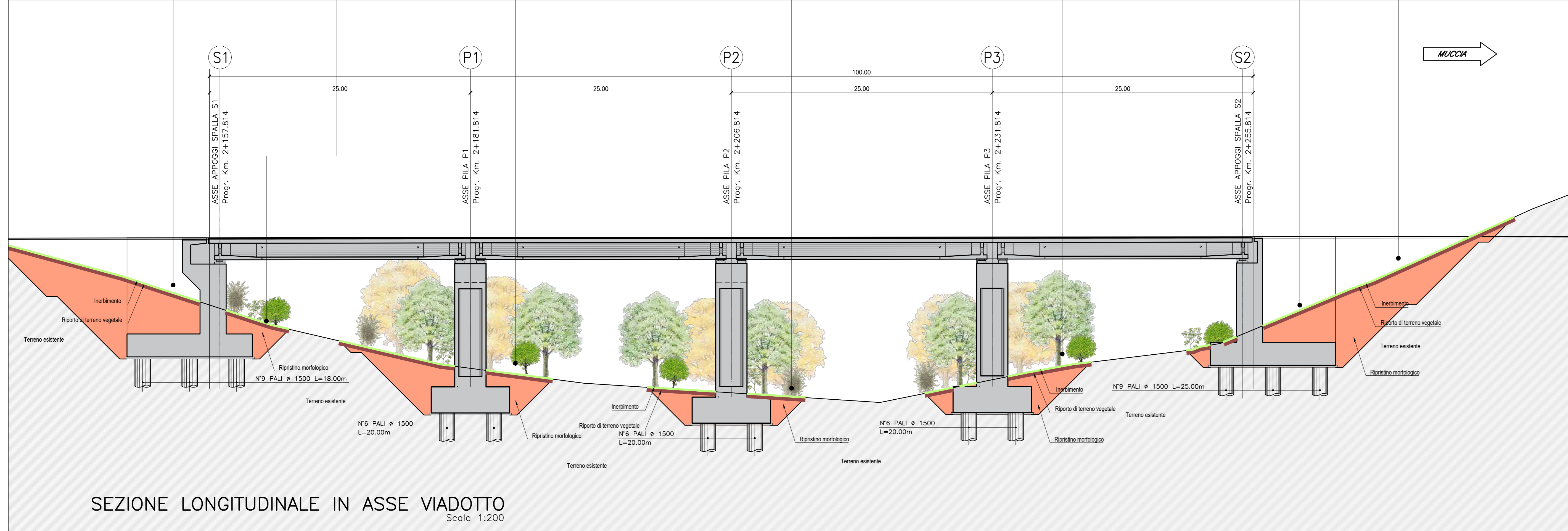
SEZIONE LONGITUDINALE A-A' (scala 1:200)
