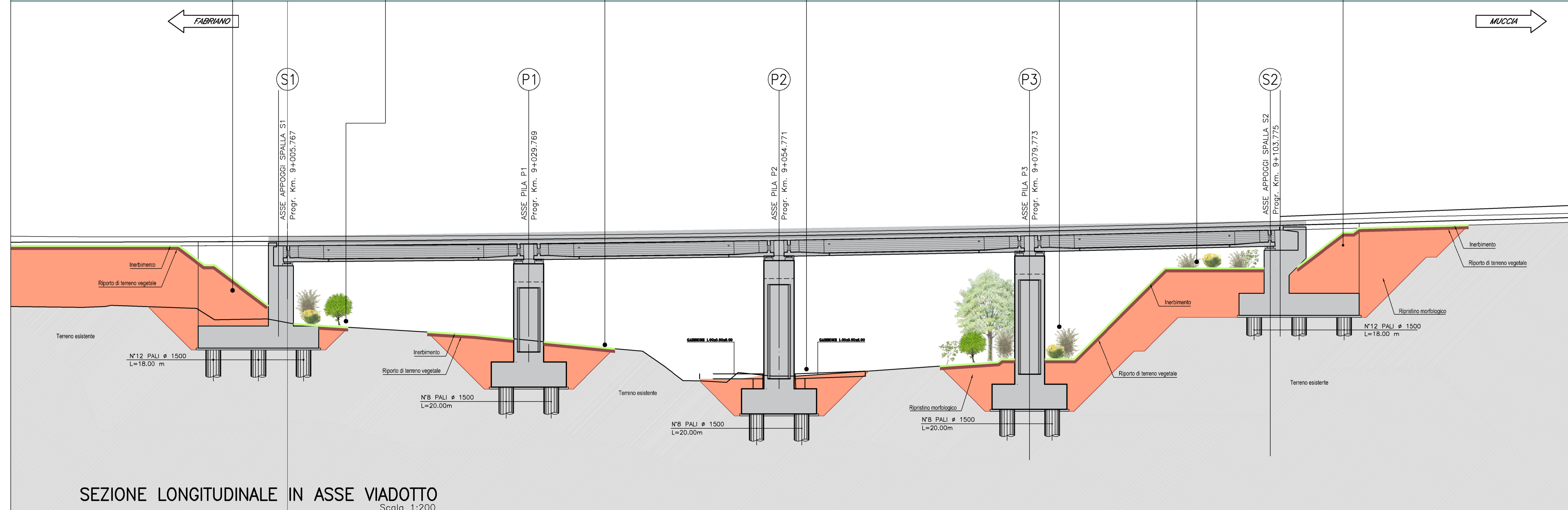
SEZIONE LONGITUDINALE A-A' (scala 1:200)
