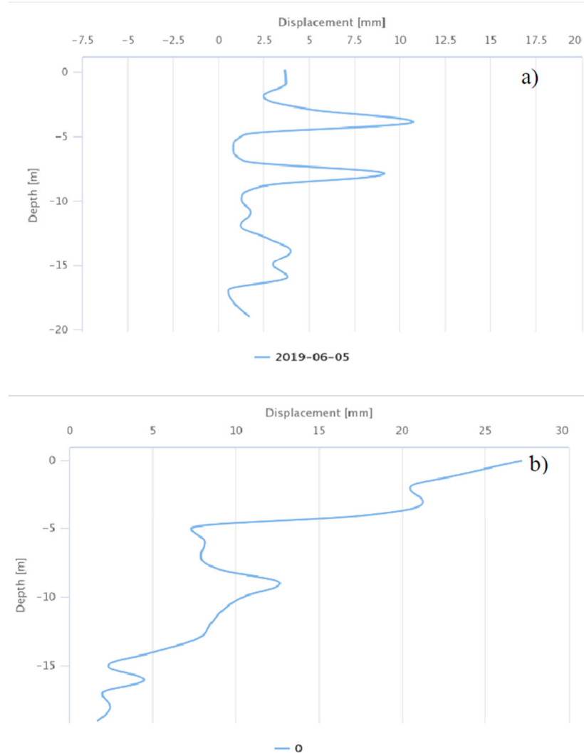
Figura 6: Confronto fra i dati di spostamento differenziale locale in direzione di massima pendenza registrati a) dal MEMS e b) dalla cella elettrolitica per l'inclinometro SF MUMS.
