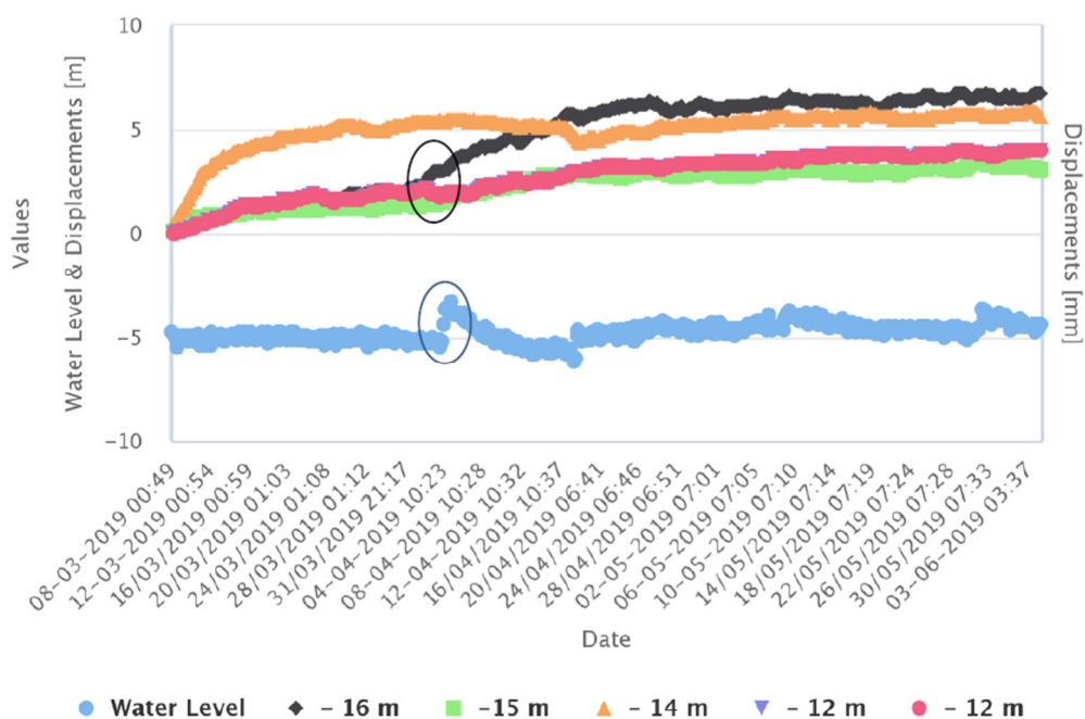
Figura 25: Confronto fra i principali spostamenti differenziali locali e livello della falda idrica registrata dai due piezometri per l'inclinometro SA MUMS.
