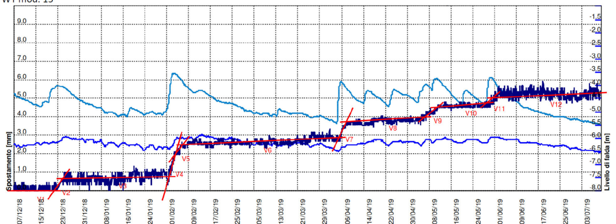
Figura 29: Confronto del modulo di spostamento (in blu scuro) con il monitoraggio della posizione della falda (in azzurro e blu elettrico).
