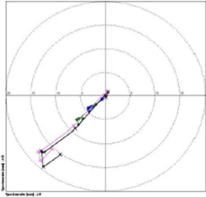
Diagramma polare cumulato Rif. lettura zero 11/03/2019
