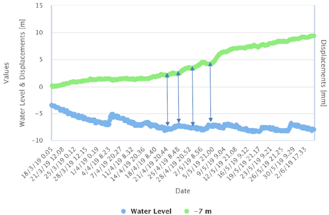
Figura 11: Confronto fra spostamenti differenziali locali alla profondità di 7 metri e livello idrico per l'inclinometro SG MUMS.
