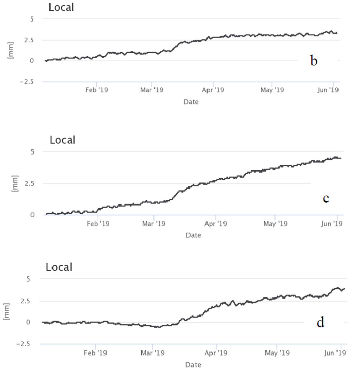
Figura 16: Andamento nel tempo degli spostamenti differenziali locali in direzione di massima pendenza registrati rispettivamente alle profondità di a) 10, b) 9, c) 8 e d) 6 m per l'inclinometro SC MUMS.
