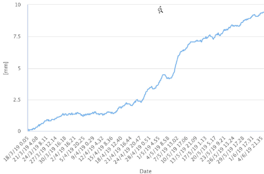
Figura 10: Andamento nel tempo degli spostamenti locali registrati a 7 metri di profondità (MEMS) per l'inclinometro SG MUMS.
