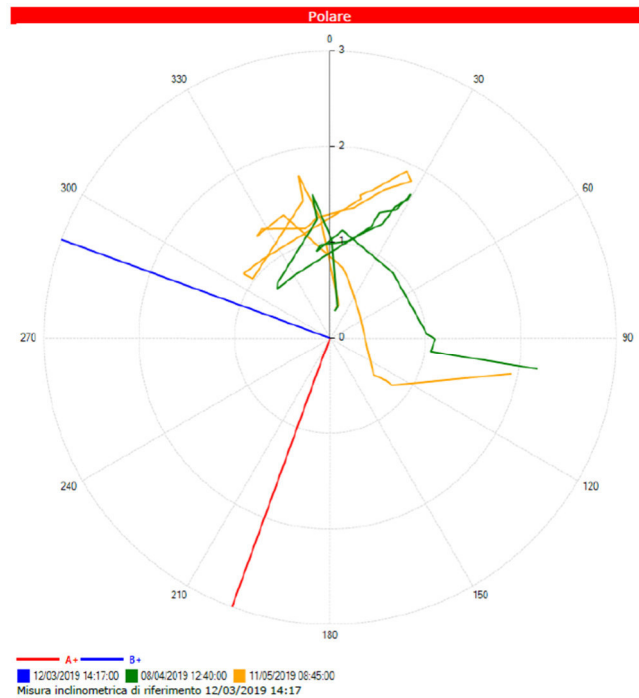
Figura 28: Diagramma polare degli azimuth degli spostamenti registrati nell'inclinometro SB INCL.
