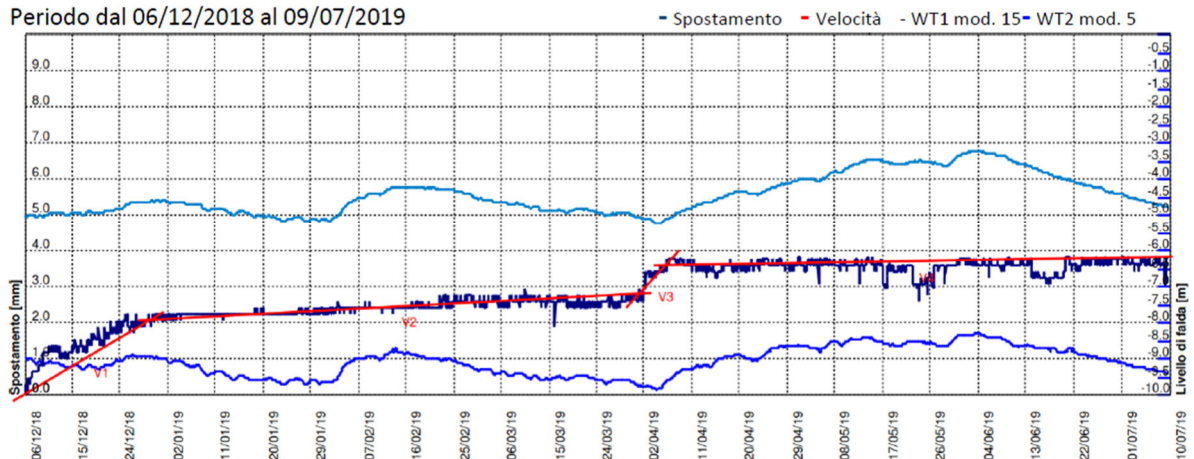
Figura 19: Grafico del modulo di spostamento (in blu scuro) con indicazione delle velocità (in rosso) e dell'andamento della posizione della falda (in azzurro e blu elettrico) per l'inclinometro SD DMS.
