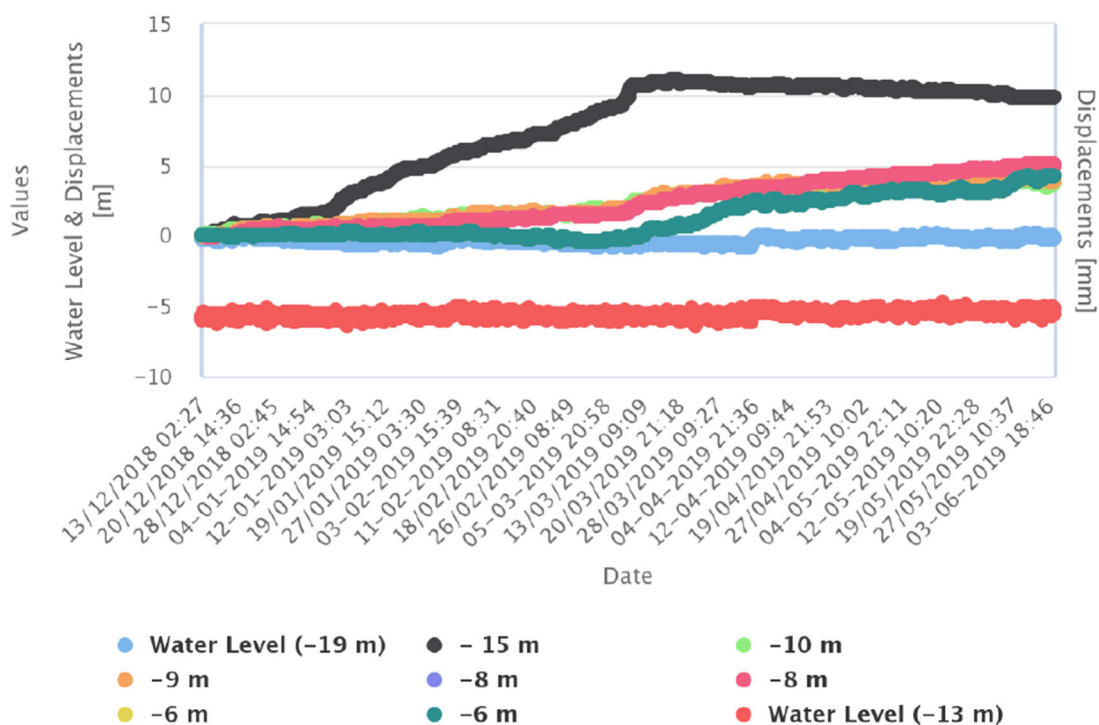
Figura 17: Confronto fra i principali spostamenti differenziali locali e livello della falda idrica registrata dai due piezometri per l'inclinometro SC MUMS.
