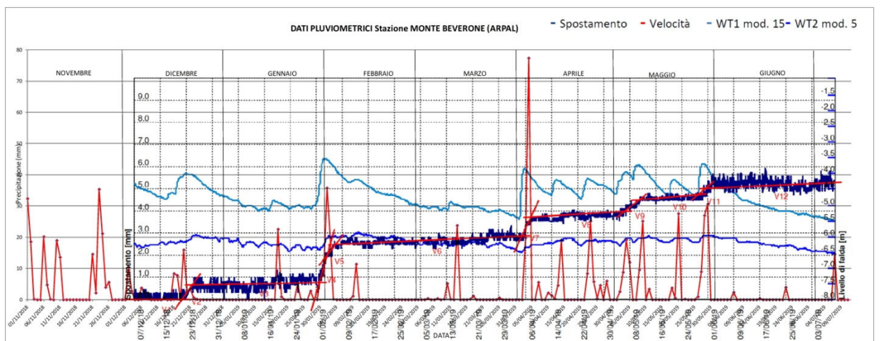
Figura 31: Sovrapposizione grafico modulo spostamento-monitoraggio piezometrico di Figura 29 con il grafico delle precipitazioni cumulate nel periodo Novembre 2018-Maggio 2019 registrate dalla stazione pluviometrica di Monte Beverone Figura 30.
