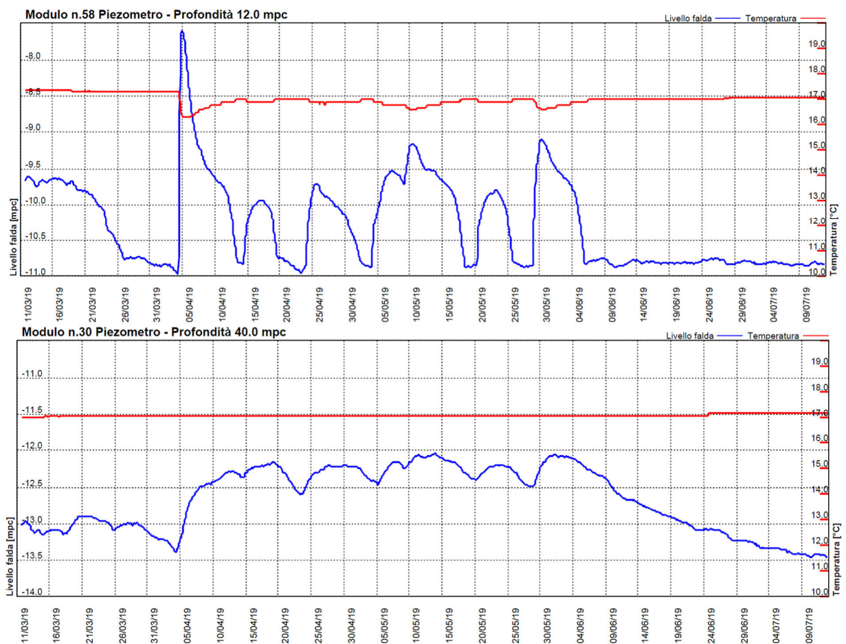
Figura 21: Grafici dell'andamento della posizione della falda (in blu) e della temperatura misurate rispettivamente nei sensori WT1 e WT2. Per l'inclinometro SA DMS.
