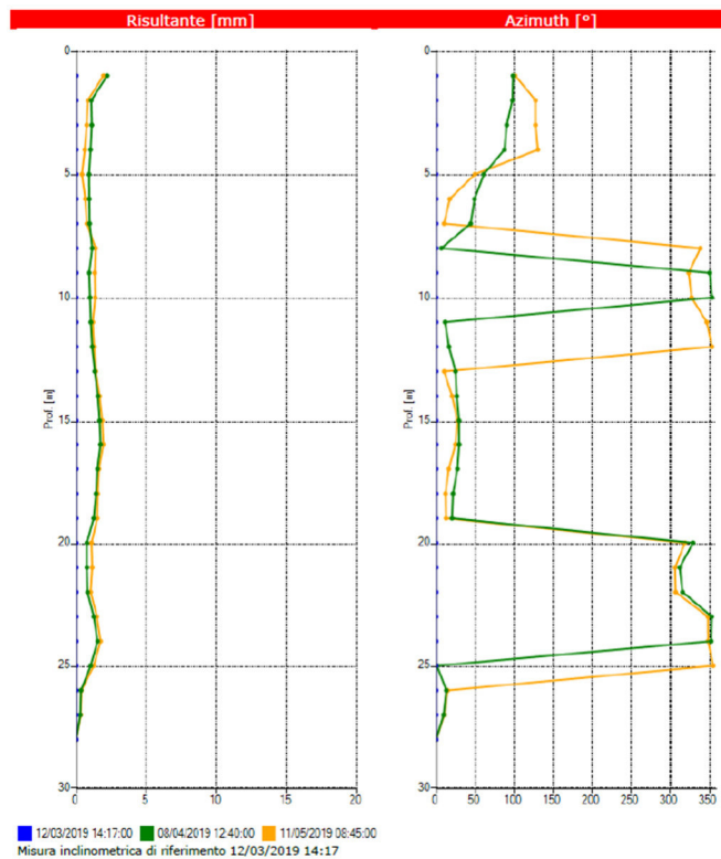
Figura 27: Grafici degli spostamenti cumulati e azimutali registrati nell'inclinometro SB INCL.
