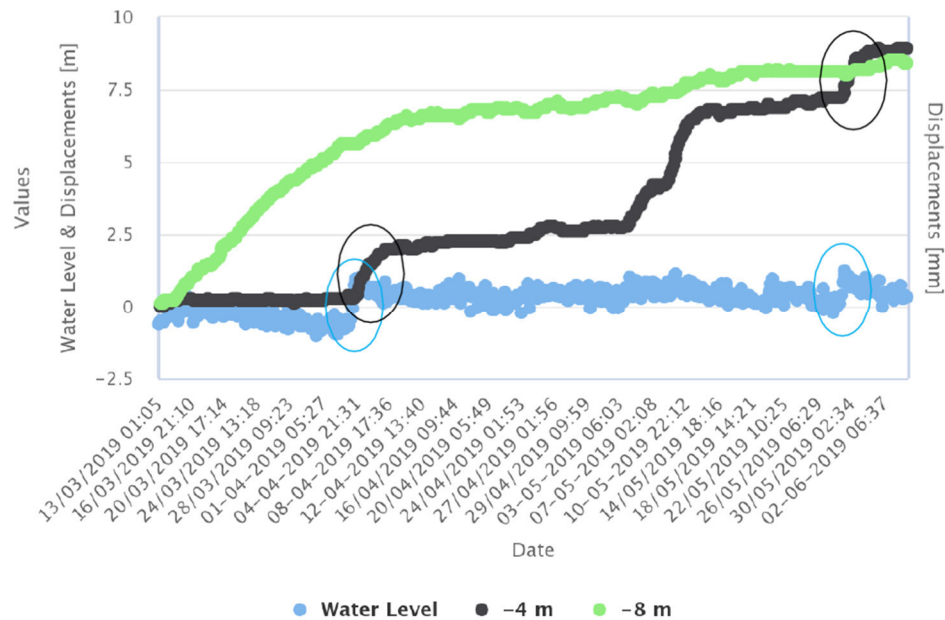
Figura 8: Confronto fra spostamenti differenziali locali alla profondità di 8 e 4 metri e livello idrico per l'inclinometro SF MUMS.
