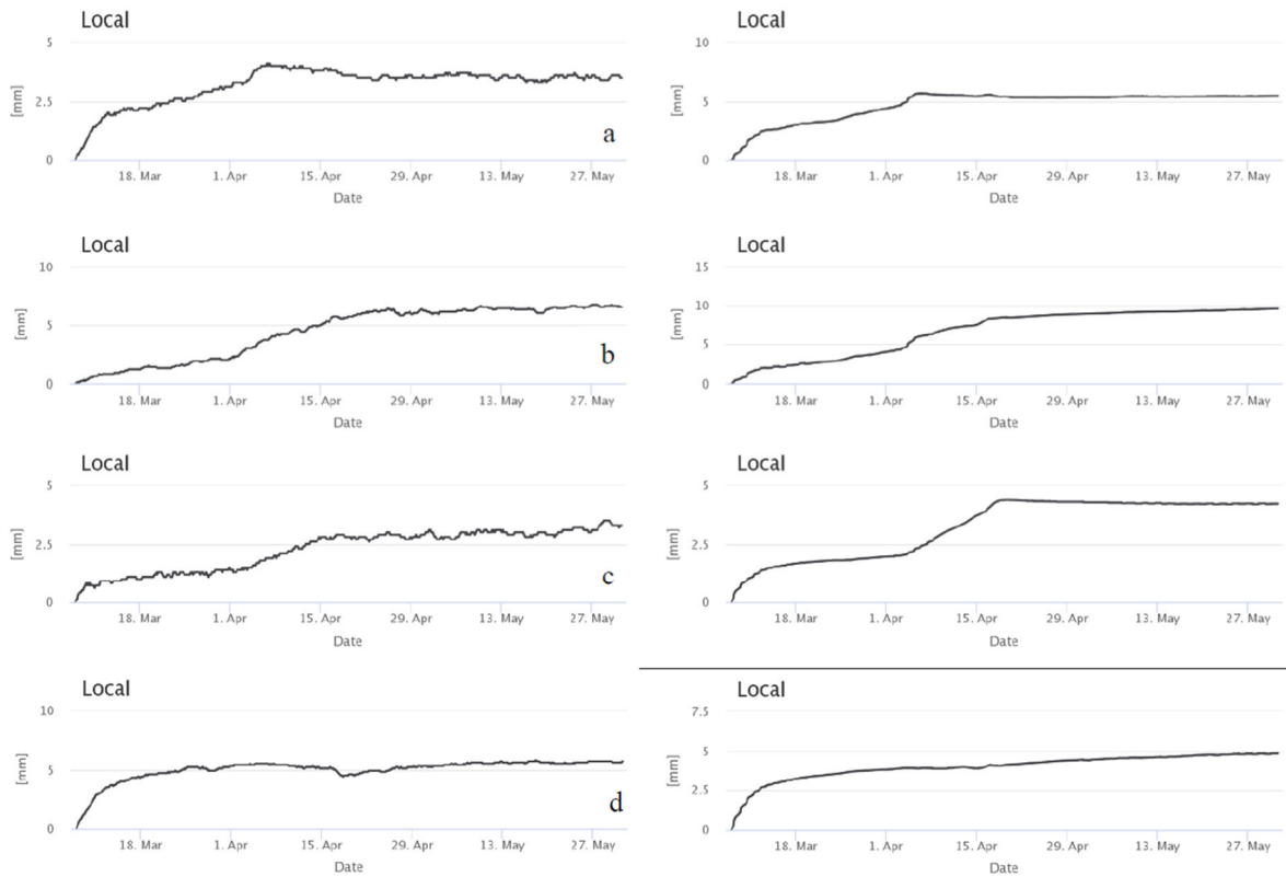
Figura 23: Andamento nel tempo degli spostamenti locali registrati da MEMS 3D (sinistra) e sensore elettrolitico 2D (destra) alle profondità rispettivamente (dall'alto) di a) 17, b) 16, c) 15 e d) 14 m per l'inclinometro SA MUMS.
