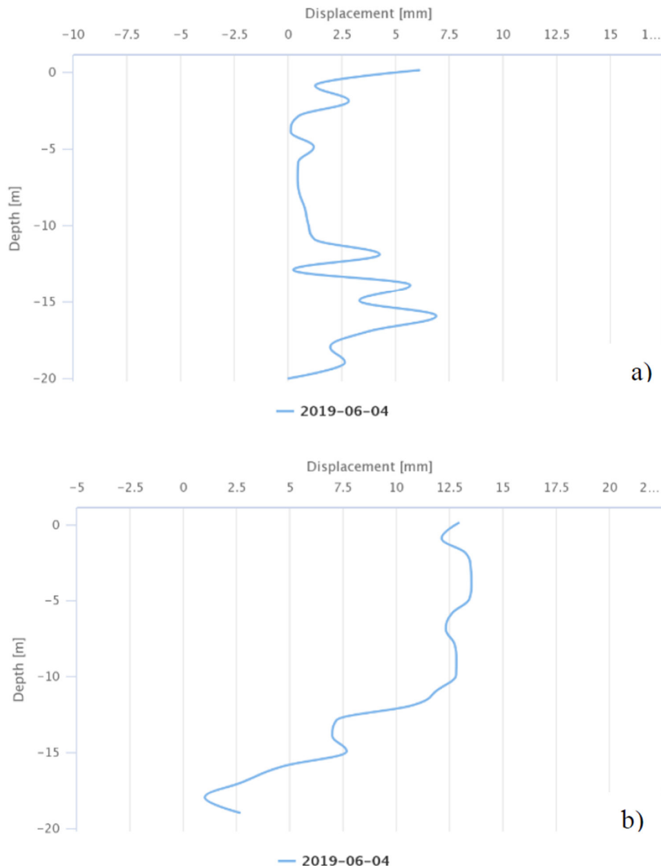
Figura 22: Dati di spostamento differenziale locale e cumulato in direzione di massima pendenza registrati dai sensori MEMS per l'inclinometro SA MUMS.
