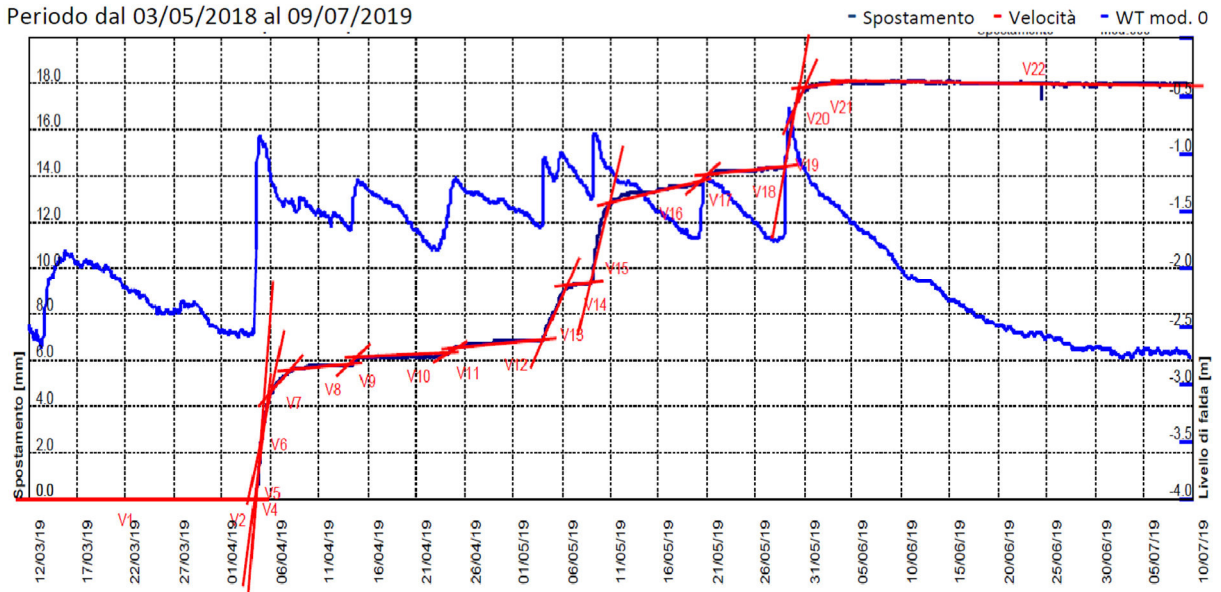
Figura 5: Grafico del modulo di spostamento (in blu scuro) con indicazione delle velocità (in rosso) e dell'andamento della posizione della falda (blu elettrico) per l'inclinometro SF DMS.
