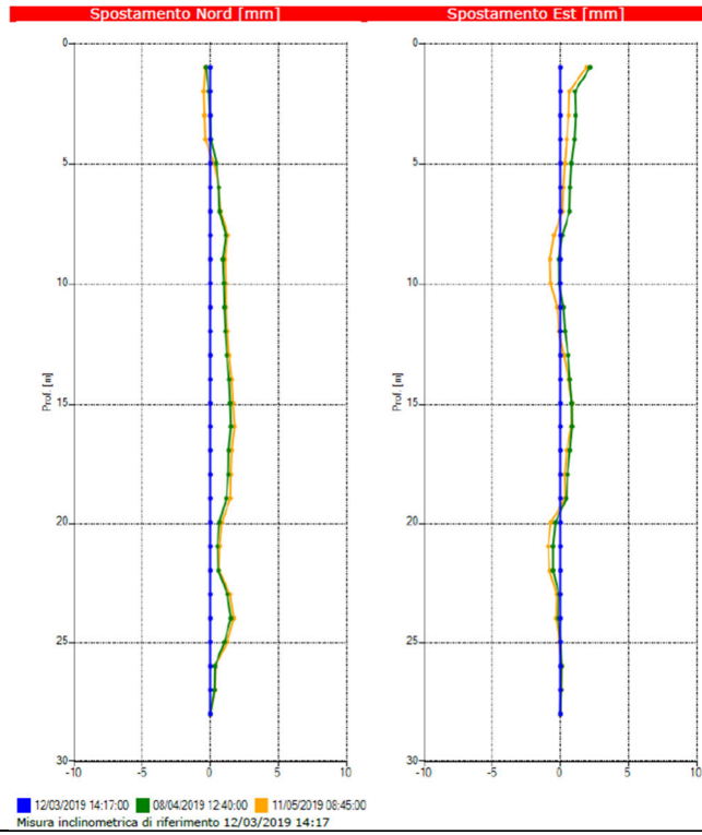
Figura 26: Grafici degli spostamenti differenziali locali (Nord ed Est) registrati nell'inclinometro SB INCL.
