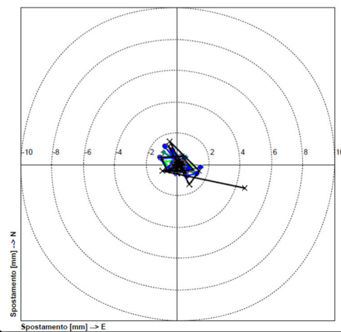
Figura 20: Grafici spostamenti differenziali e cumulativi e relativi vettori di spostamento per l'inclinometro SA DMS.
