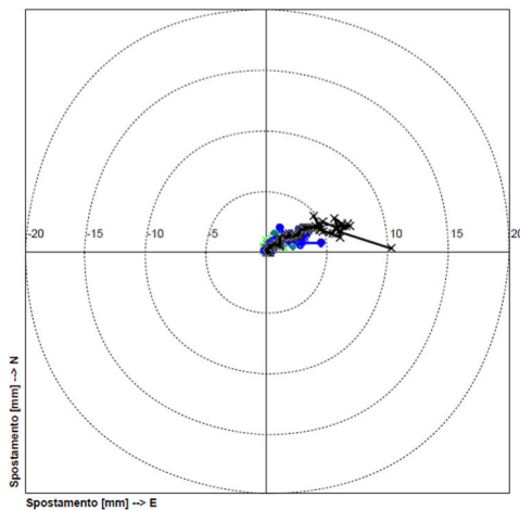
Figura 20: Grafici spostamenti differenziali e cumulativi e relativi vettori di spostamento per l'inclinometro SA DMS.
