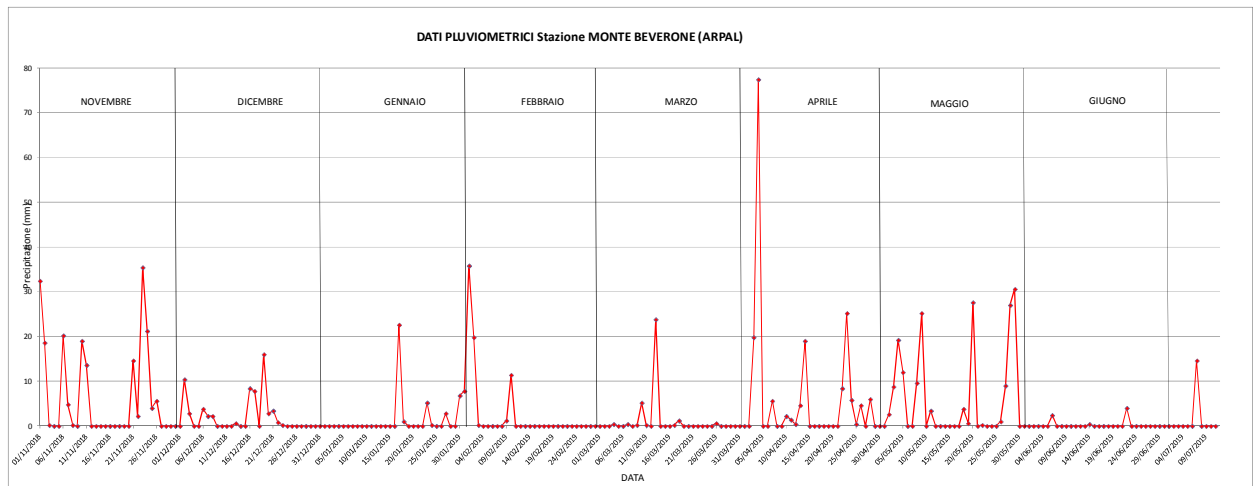
Figura 30: Grafico delle precipitazioni cumulate nel periodo Novembre 2018-Maggio 2019 registrate dalla stazione pluviometrica di Monte Beverone.
