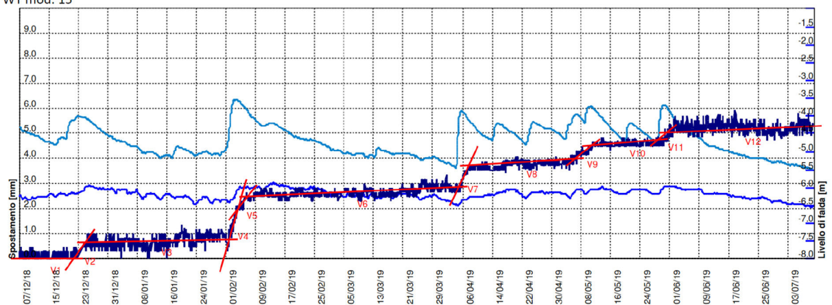
Figura 13: Grafico del modulo di spostamento (in blu scuro) con indicazione delle velocità (in rosso) e dell'andamento della posizione della falda (in azzurro e blu elettrico) per l'inclinometro SF DMS.
