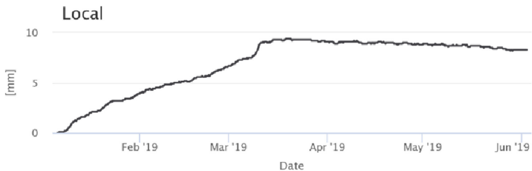
Figura 15: Andamento nel tempo degli spostamenti differenziali locali in direzione di massima pendenza registrati a 15 m di profondità per l'inclinometro SC MUMS.
