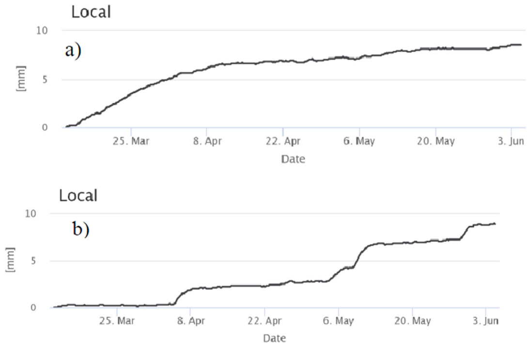
Figura 7: Andamento nel tempo degli spostamenti locali registrati a a) 8 e b) 4 m di profondità (MEMS) per l'inclinometro SF MUMS.
