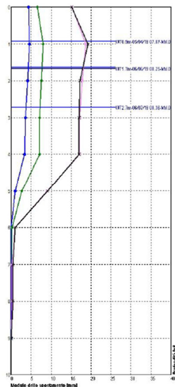
Modulo dello spostamento cumulato
