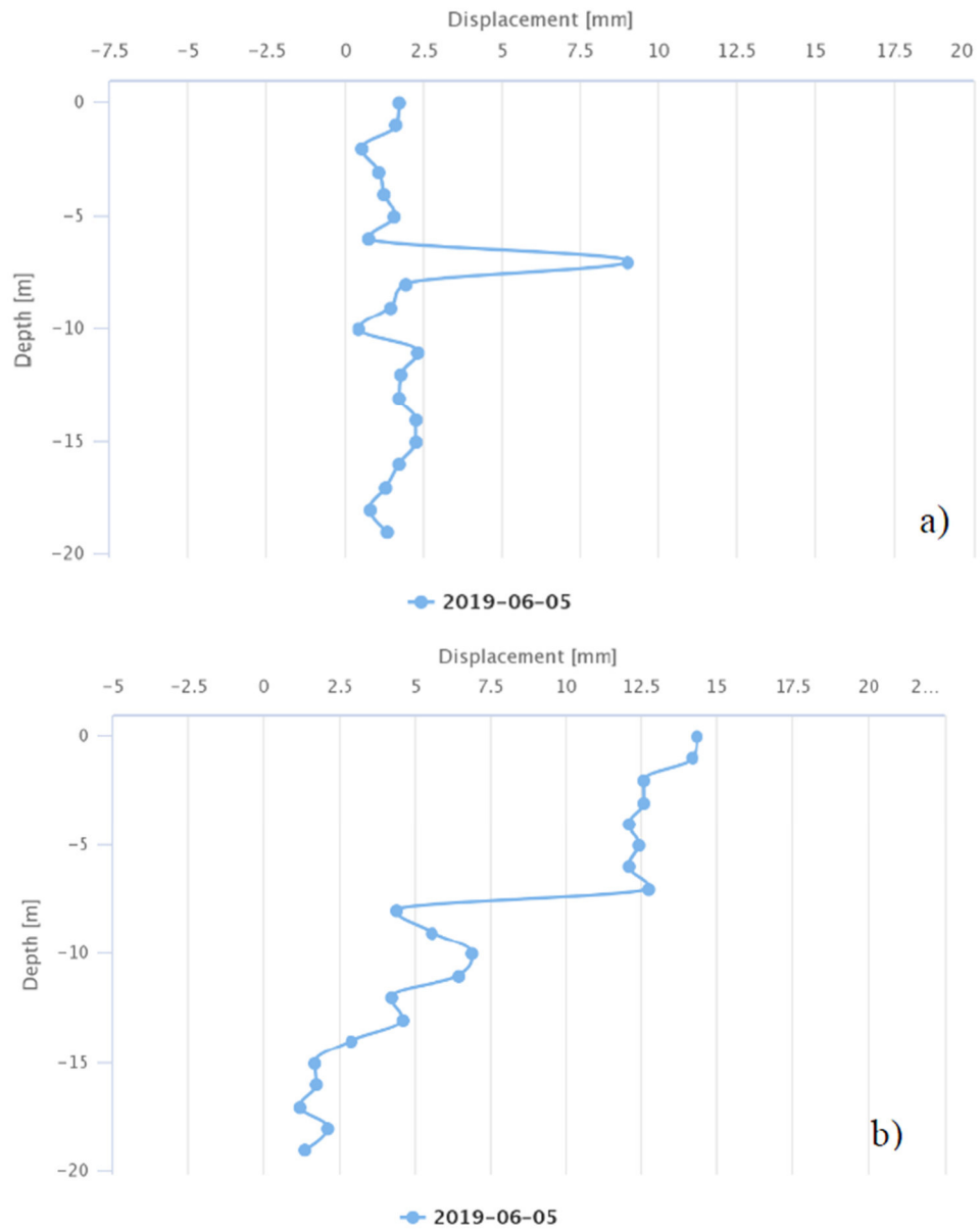
Figura 9: Confronto fra i dati di spostamento differenziale locale in direzione di massima pendenza registrati a) dal MEMS e b) dalla cella elettrolitica per l'inclinometro SG MUMS.
