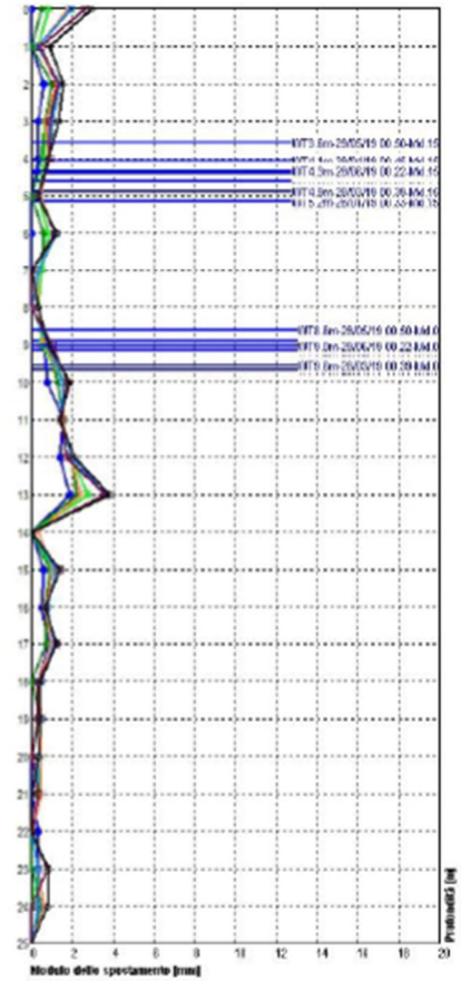
Modulo dello spostamento differenziale Rif. lettura zero 05/12/2018
