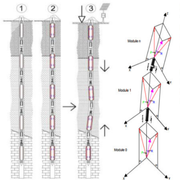
Figura 1: Esempio di funzionamento di una colonna tipo DMS.
