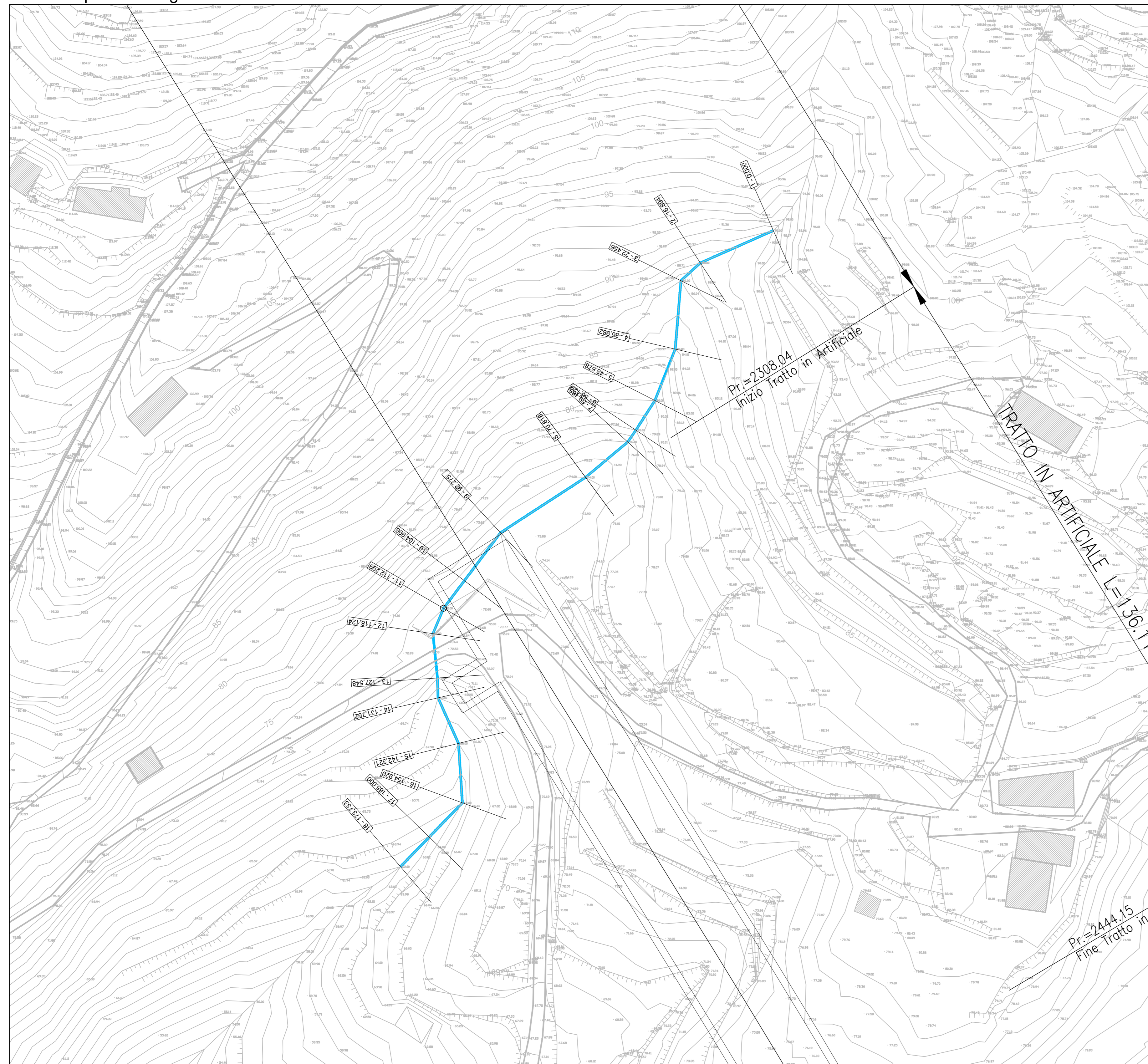
planimetria generale 1:500
