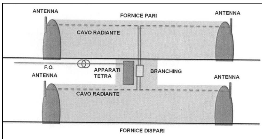
Tipologico installazione sistema TETRA per gallerie a doppio fornice
