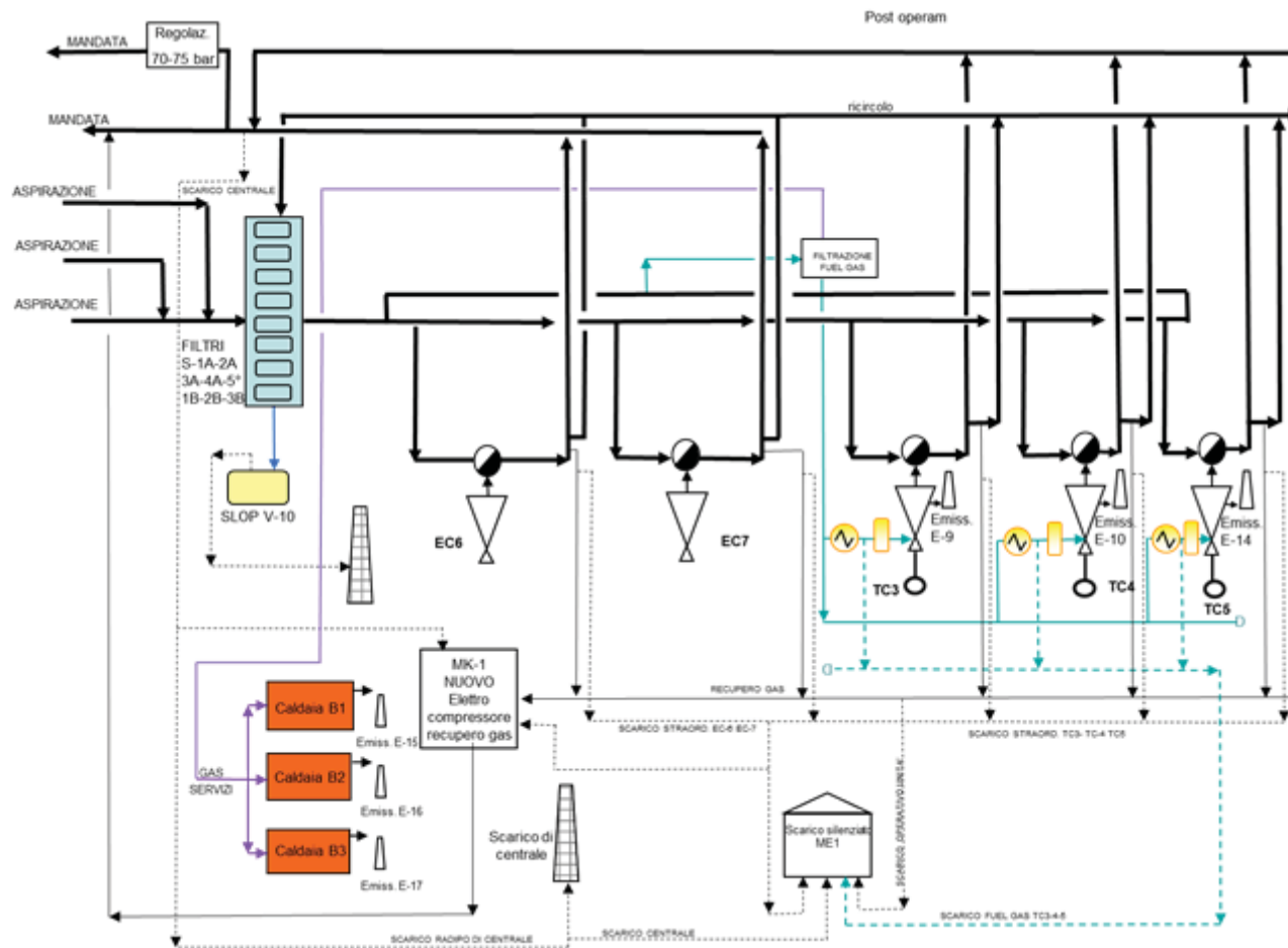
Figura 2.2-1: Schema semplificato di processo – post operam
