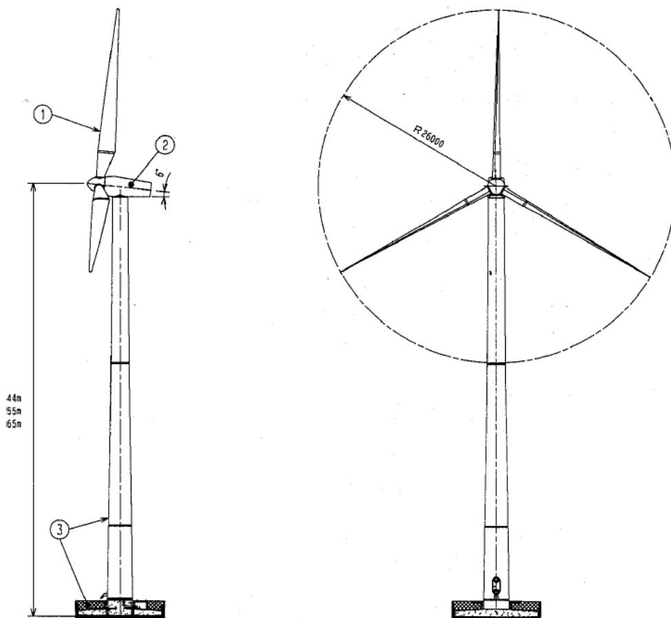
Figura 2-4: Dimensioni principali di una Gamesa G52
