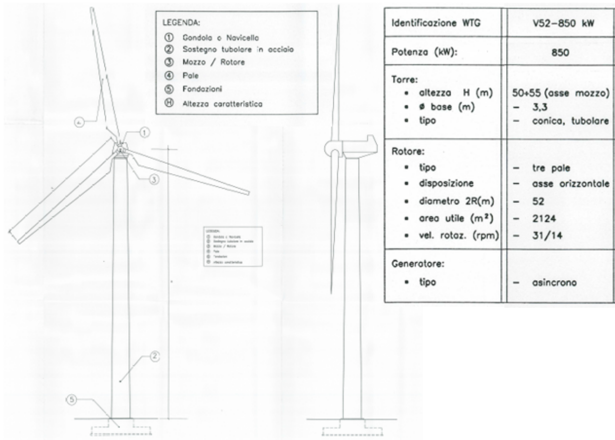
Figura 2-3: Dimensioni principali di una Vestas V52
