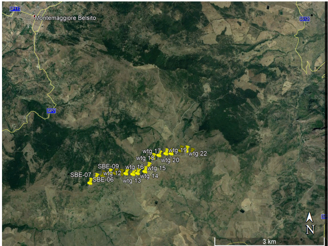
Figura 2-2: Configurazione dell'impianto esistente su ortofoto
