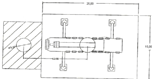
Figura 2-1: Spazio di manovra per gru
