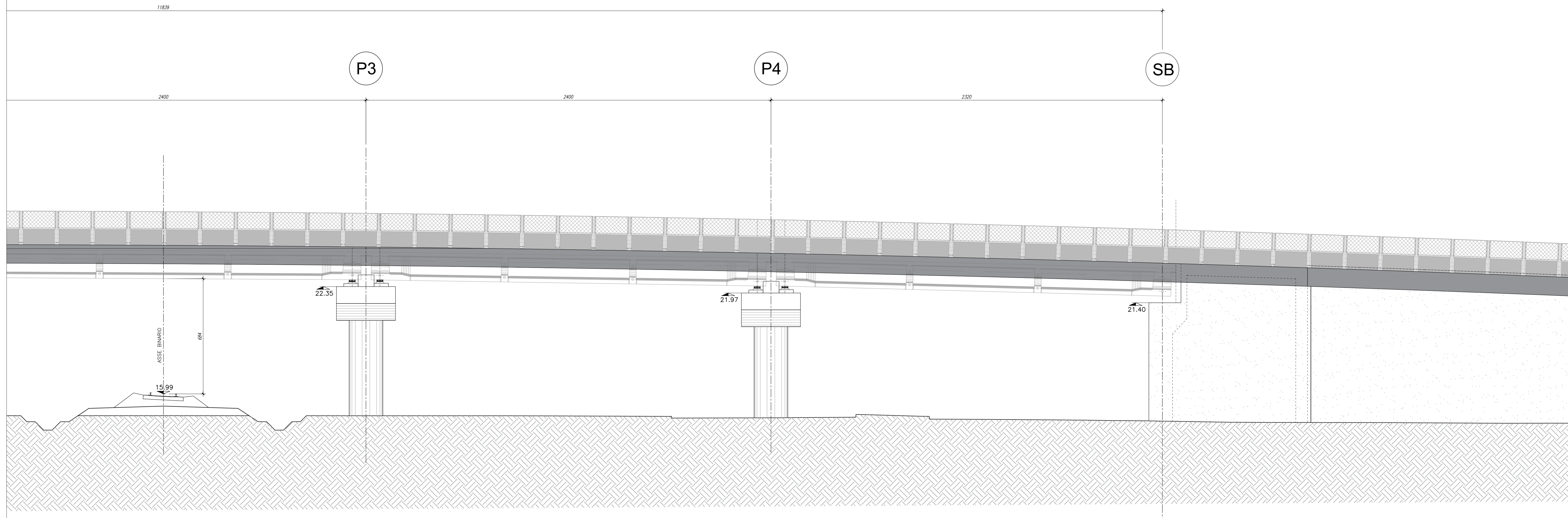
PROSPETTO LATERALE 2/2 Scala 1:100
