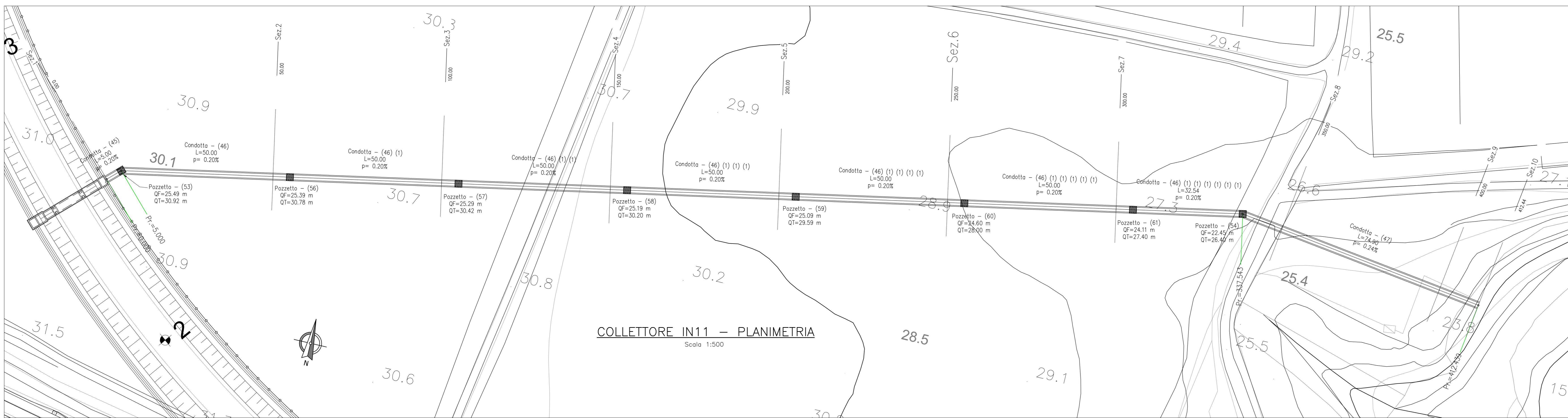
KEY PLAN – COLLETTORE IN11 (412.44 mt) Scala 1:5000
