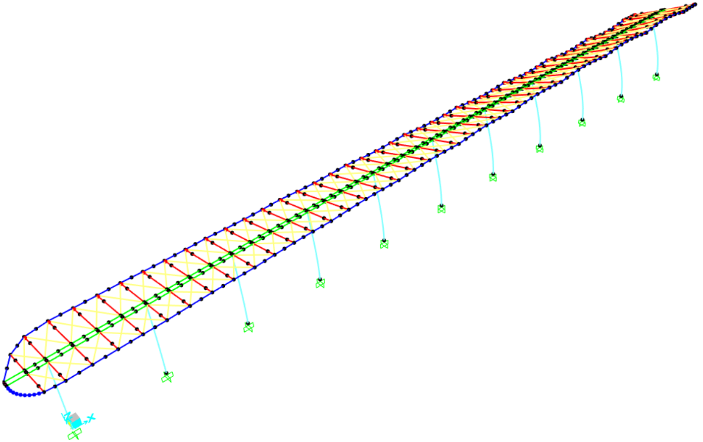
Figura 13. Deformata modale associata al primo modo.
