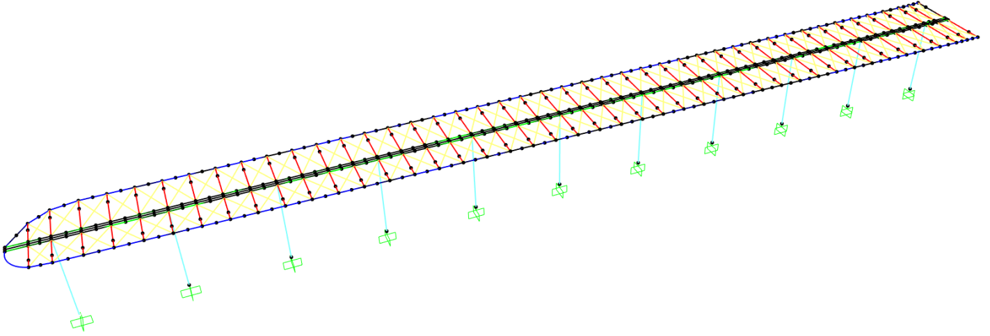
Figura 6. Modello SAP2000 struttura.
