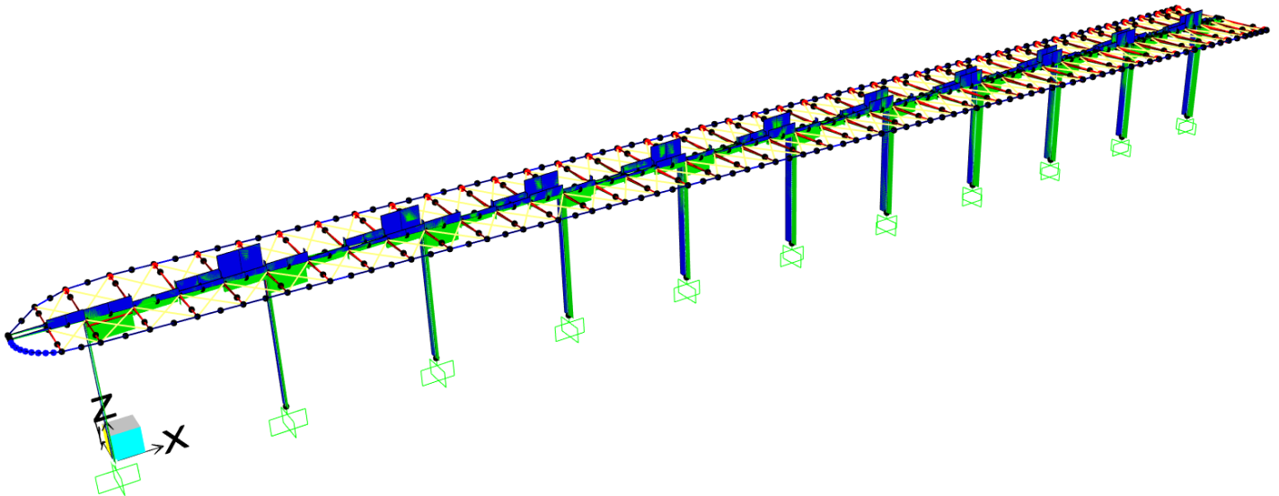
Figura 22. Diagramma del taglio V2-2 in combinazione involuppo SLV.
