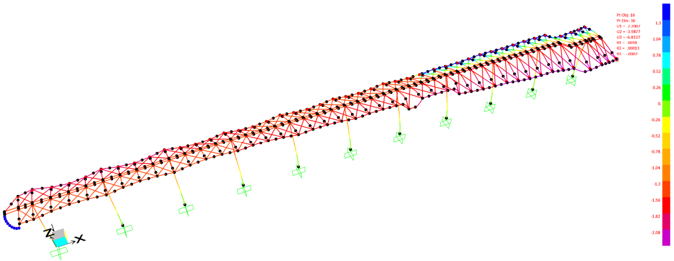
Figura 32. Spostamenti in direzione X in condizioni sismiche
