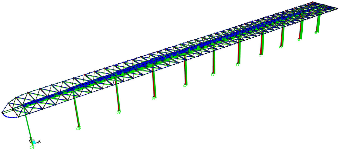
Figura 20 Diagramma dello sforzo normale in combinazione di inviluppo SLU.
