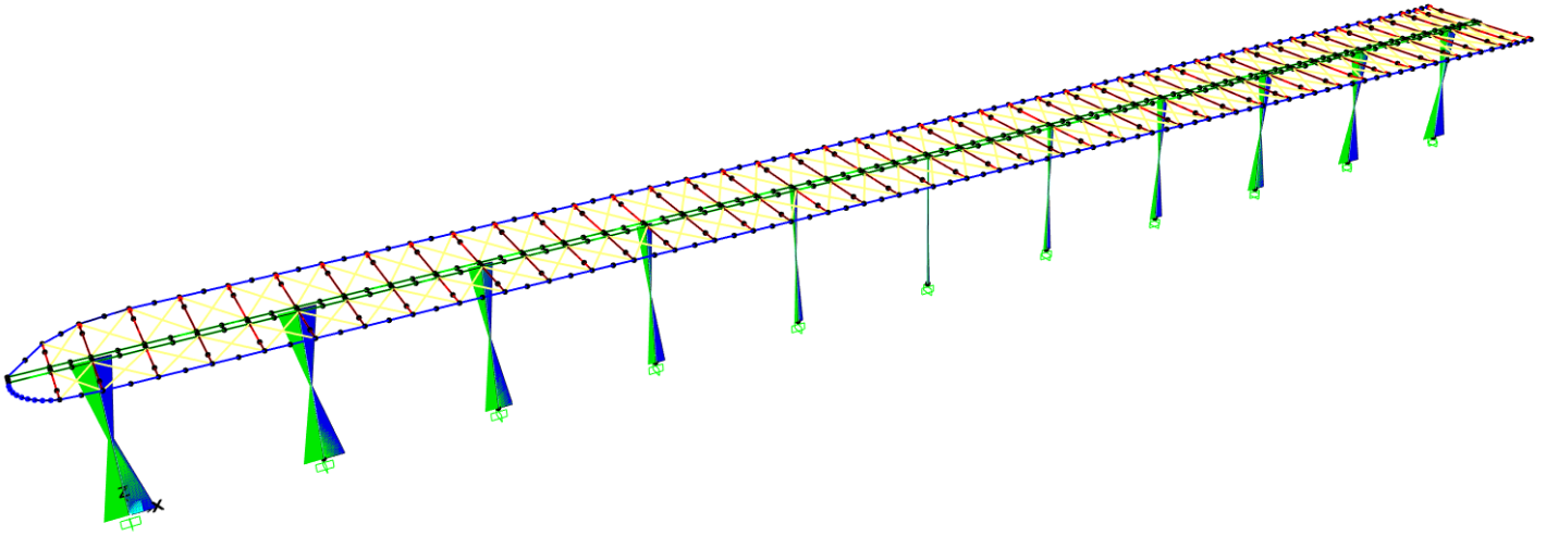
Figura 17. Diagramma del momento flettente M2-2 in combinazione di involucro SLU.
