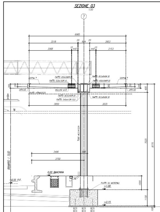
Figura 3. Sezione 03 carpenteria.
