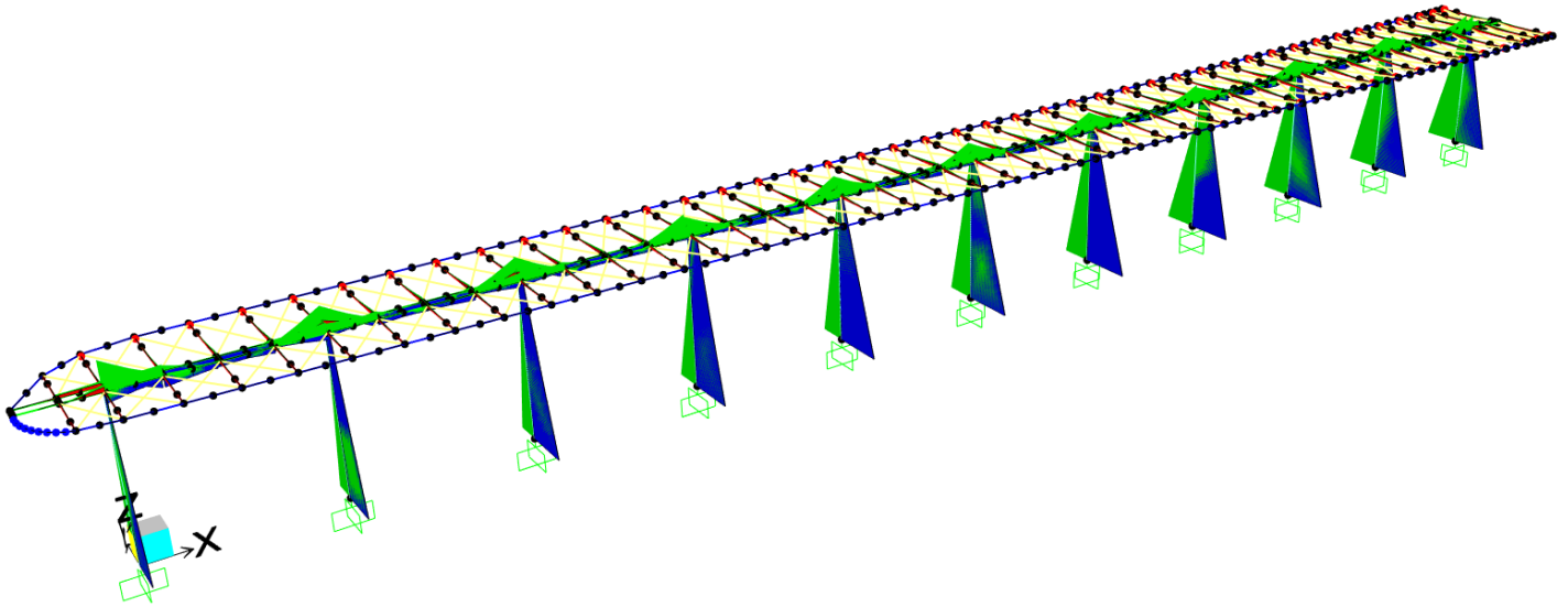
Figura 21. Diagramma del momento flettente M3-3 in combinazione involuppo SLV.
