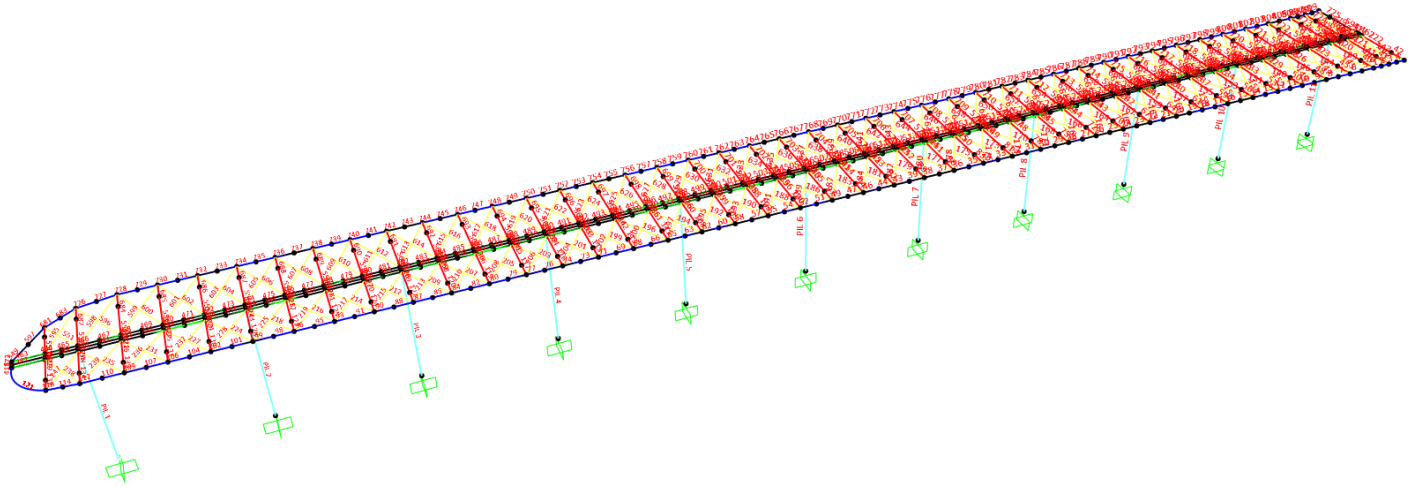
Figura 10. Modello SAP2000 struttura – numerazione degli elementi vista 3D.
