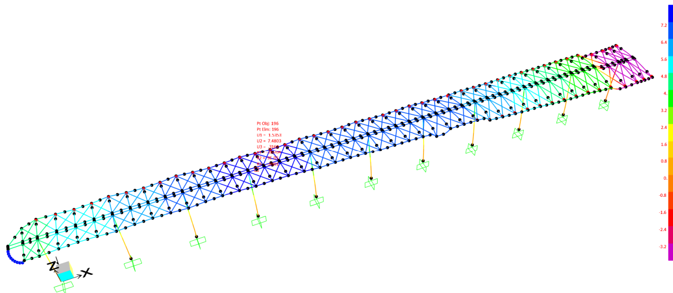
Figura 33. Spostamenti in direzione Y in condizioni sismiche.
