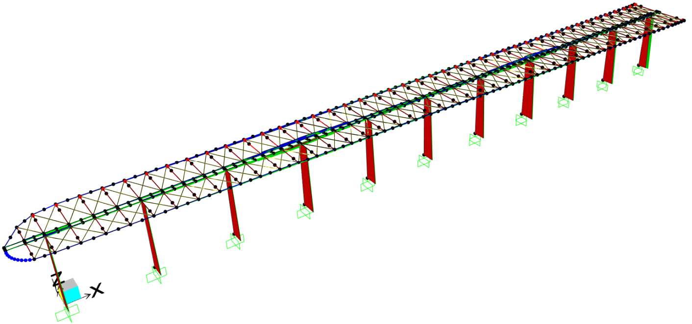
Figura 26 Diagramma dello sforzo normale in combinazione di inviluppo SLV.
