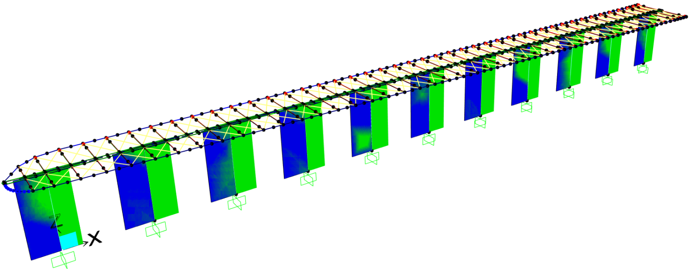
Figura 24. Diagramma del taglio V3-3 in combinazione di involucro SLV.
