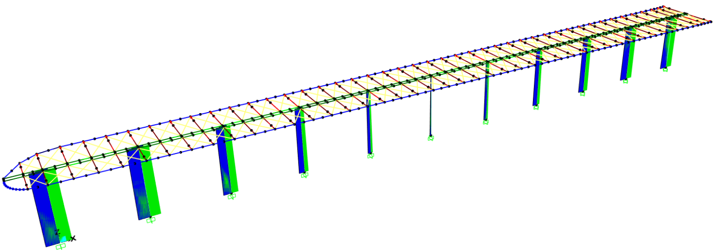
Figura 18. Diagramma del taglio V3-3 in combinazione di involucro SLU.
