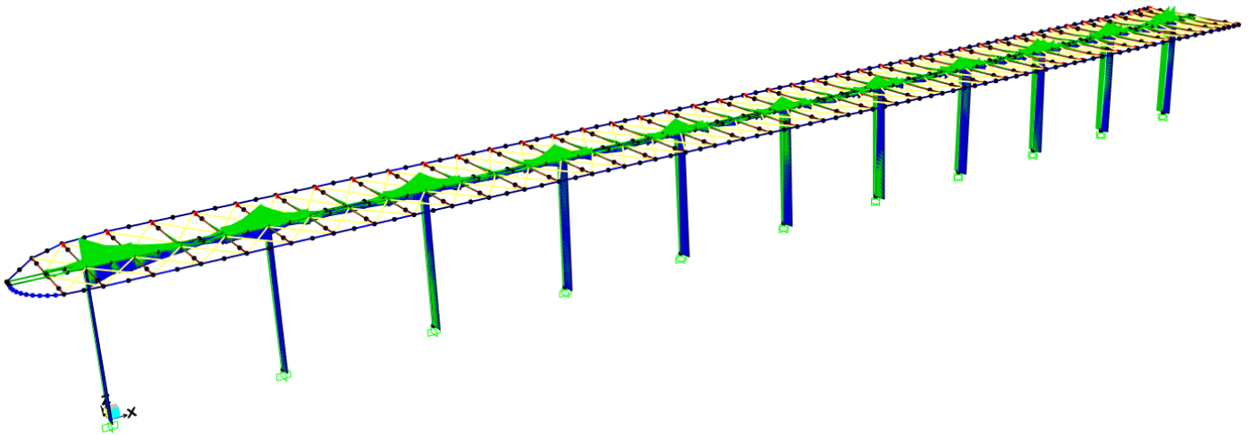
Figura 15. Diagramma del momento flettente M3-3 in combinazione involucro SLU.
