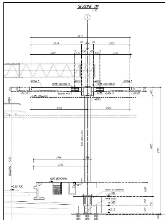
Figura 2. Sezione 02 carpenteria.
