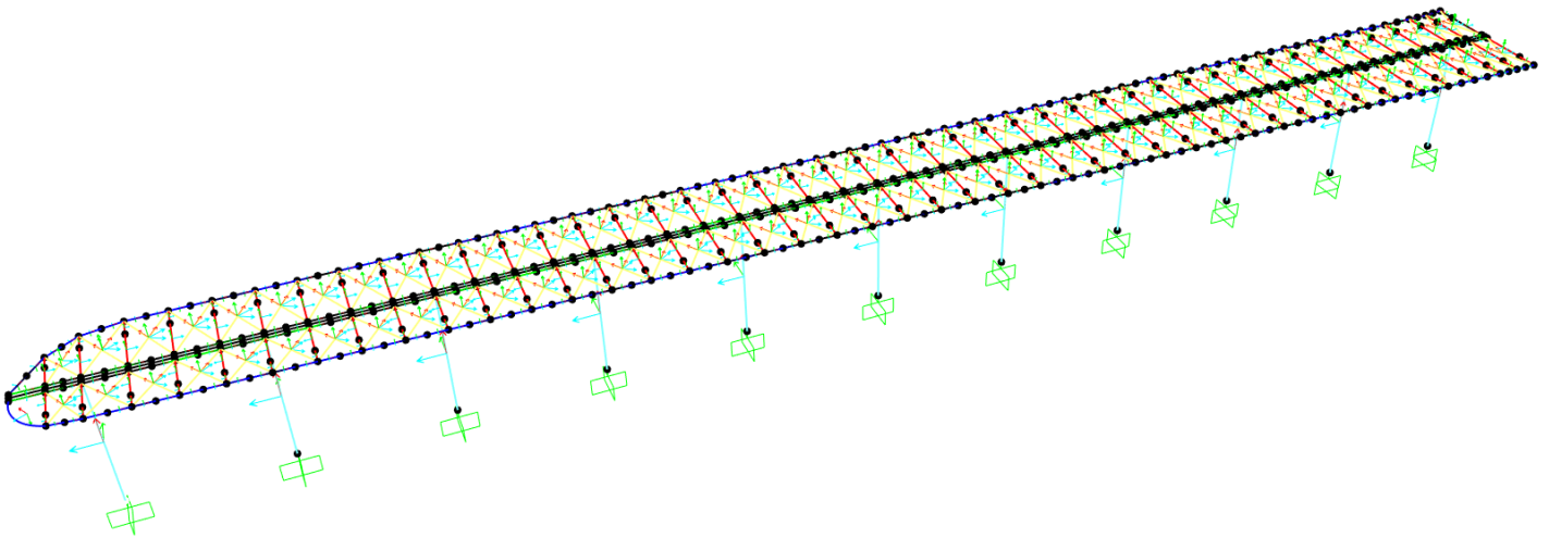
Figura 7. Assi locali elementi frame.
