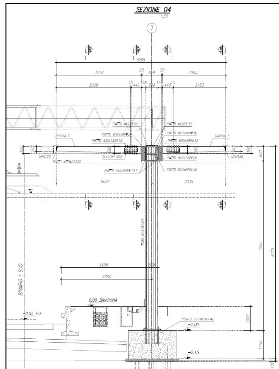
Figura 4. Sezione 04 carpenteria.
