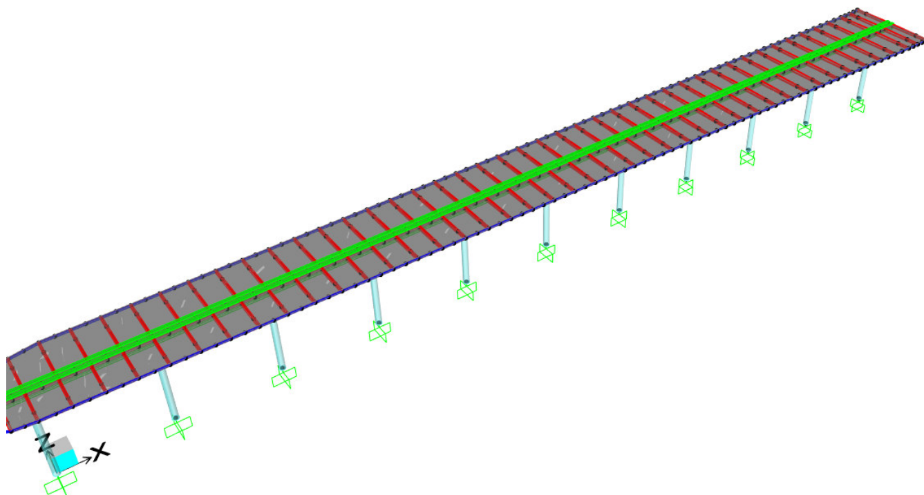
Figura 5. Modello SAP2000 struttura – Vista estrusa.
