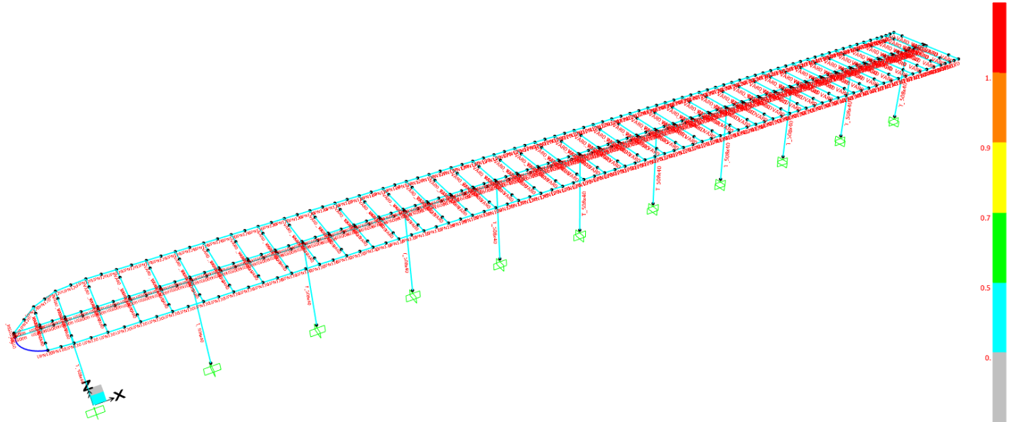
Figura 28. Sfruttamento delle membrature in acciaio.
