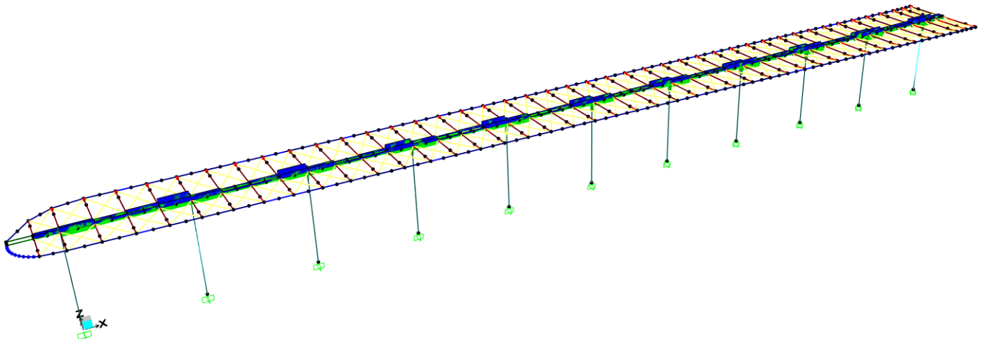
Figura 16. Diagramma del taglio V2-2 in combinazione involucro SLU.
