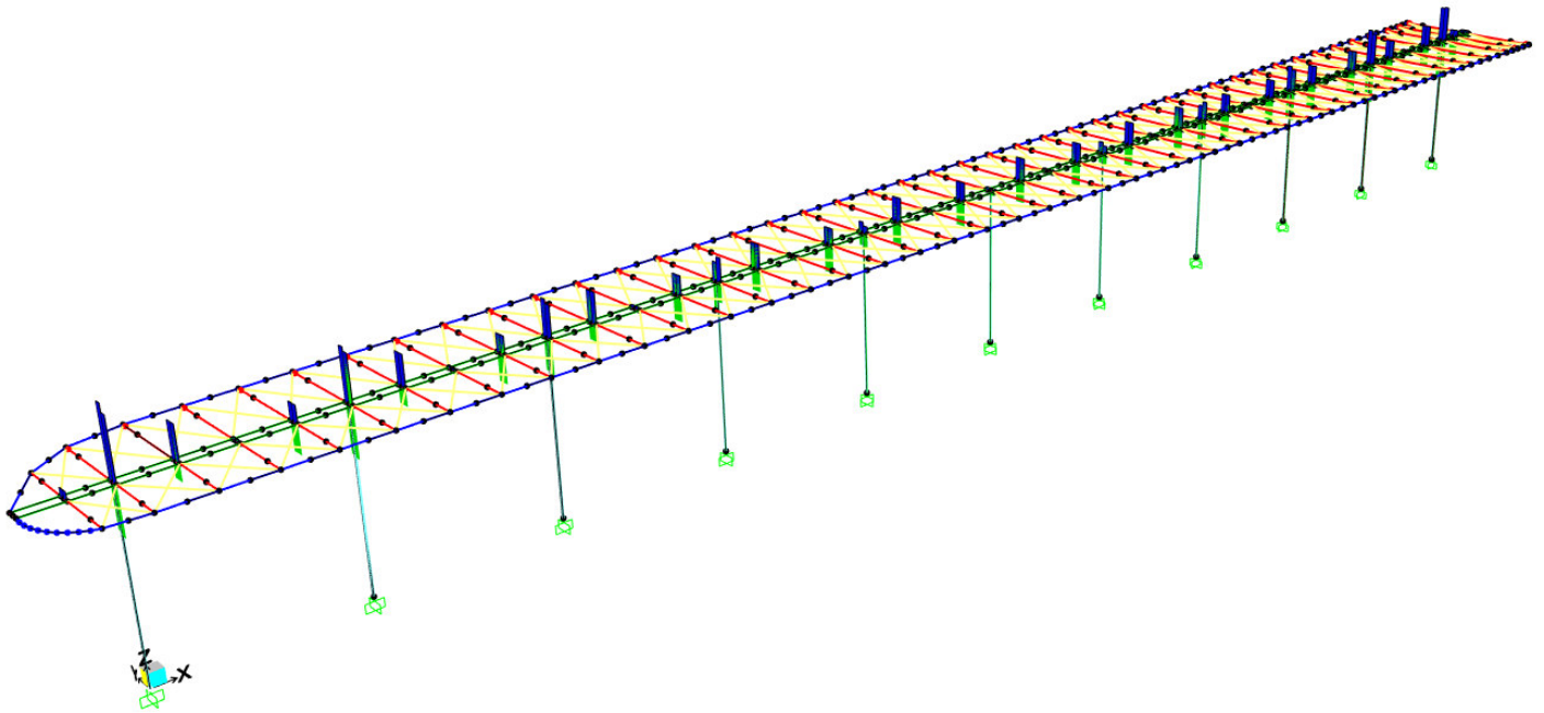
Figura 19 Diagramma del momento torcente in combinazione di inviluppo SLU.
