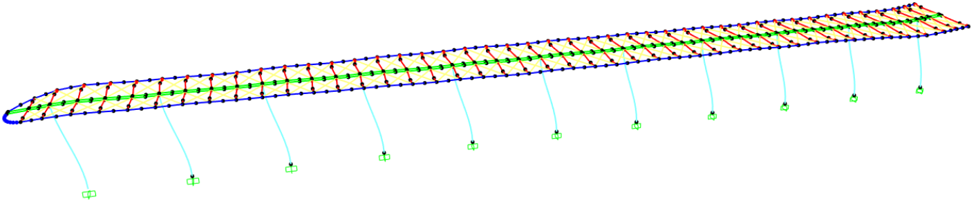
Figura 14. Deformata modale associata al quinto modo.
