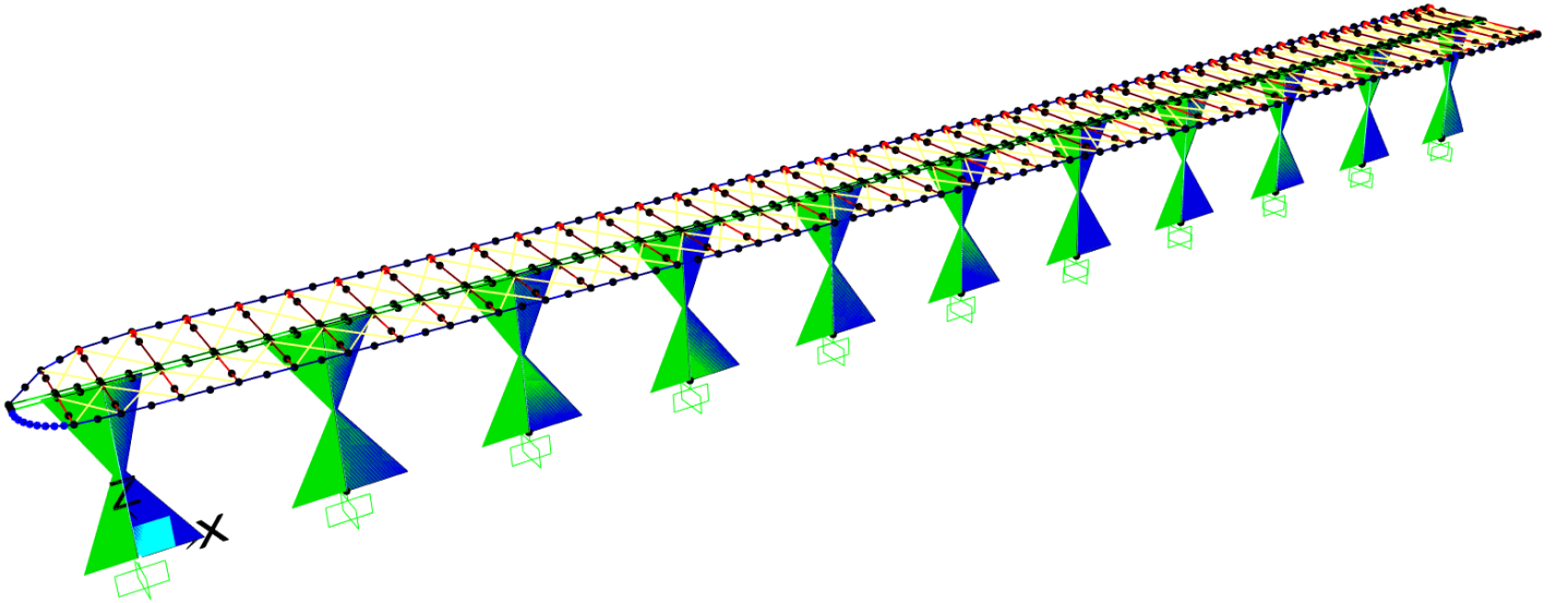
Figura 23. Diagramma del momento flettente M2-2 in combinazione di involucro SLV.
